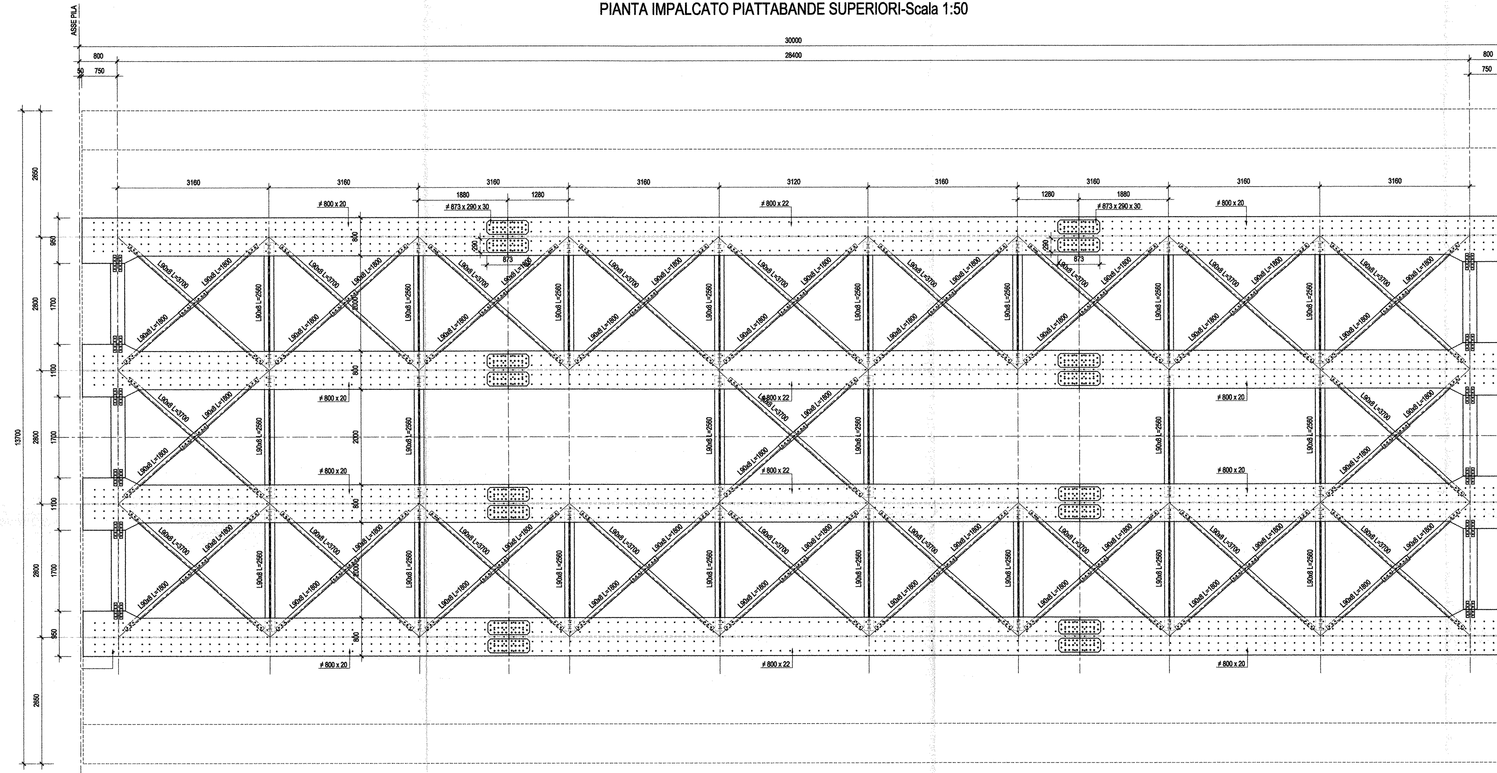
PIANTA IMPALCATO PIATTABANDE SUPERIORI-Scala 1:50
