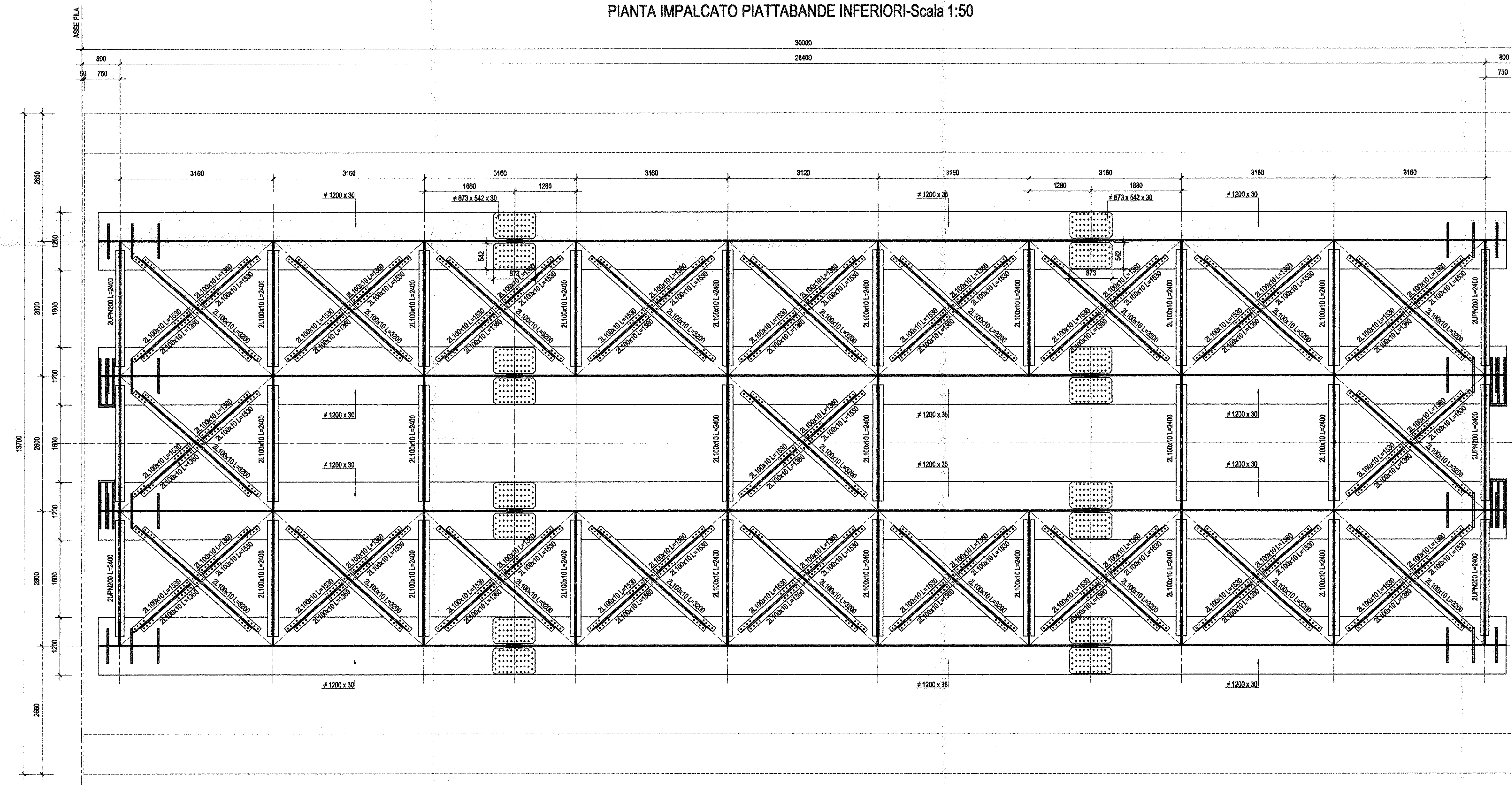
PIANTA IMPALCATO PIATTABANDE INFERIORI-Scala 1:50
