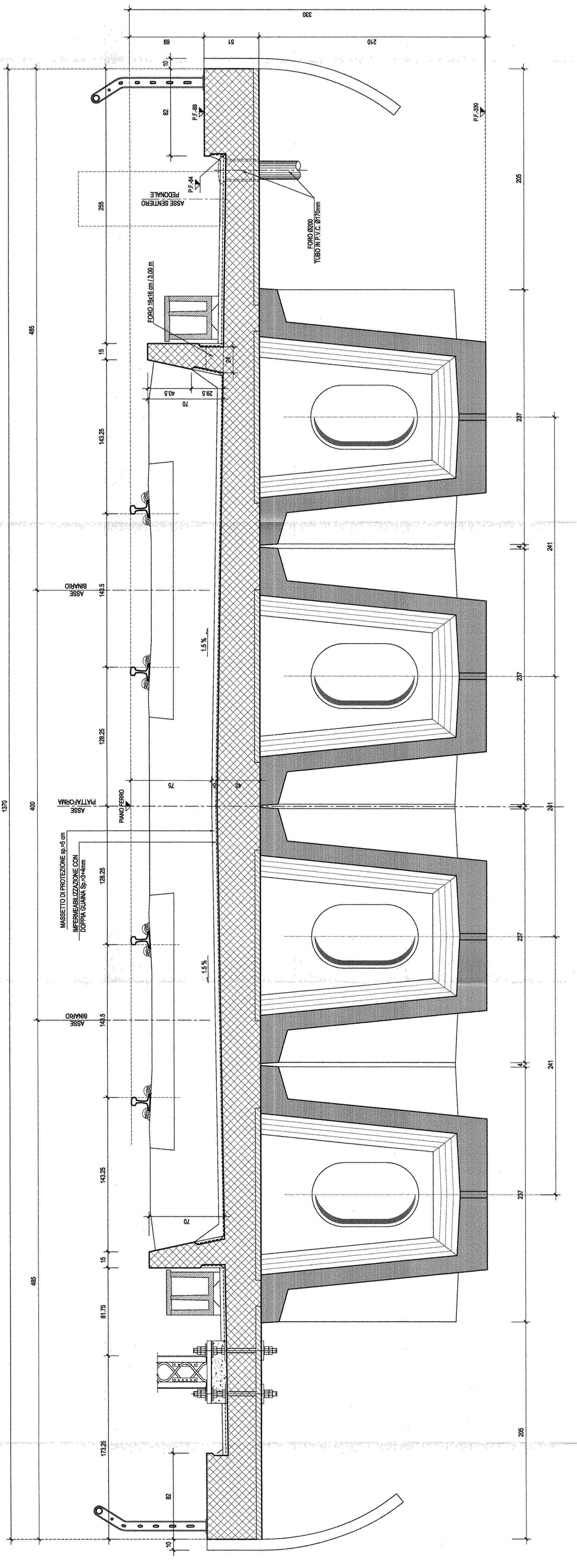
SEZIONE TRASVERSALE-Scala 1:20
