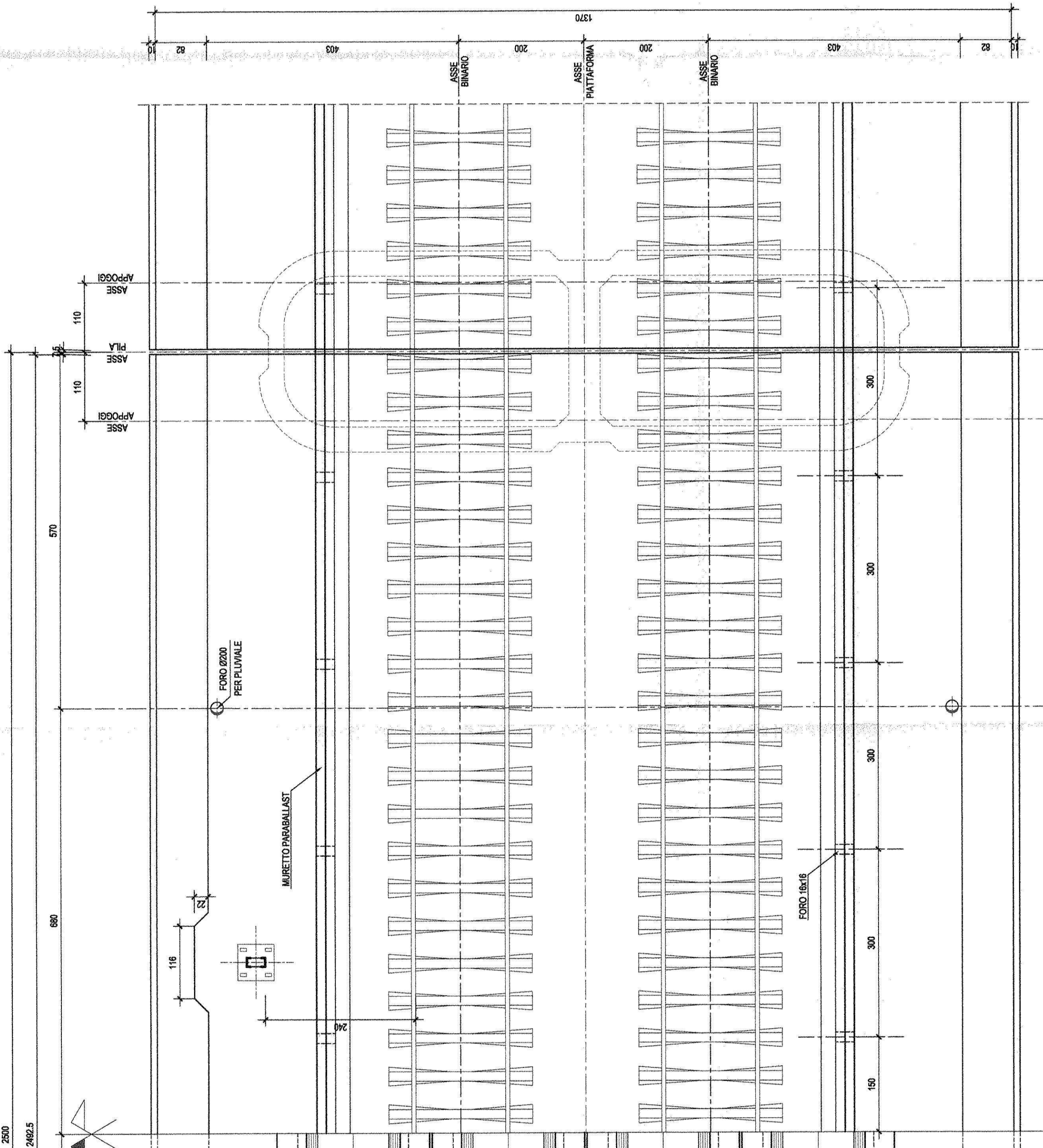
1/2 PIANTA A Q. SOLETTA-Scala 1:50
