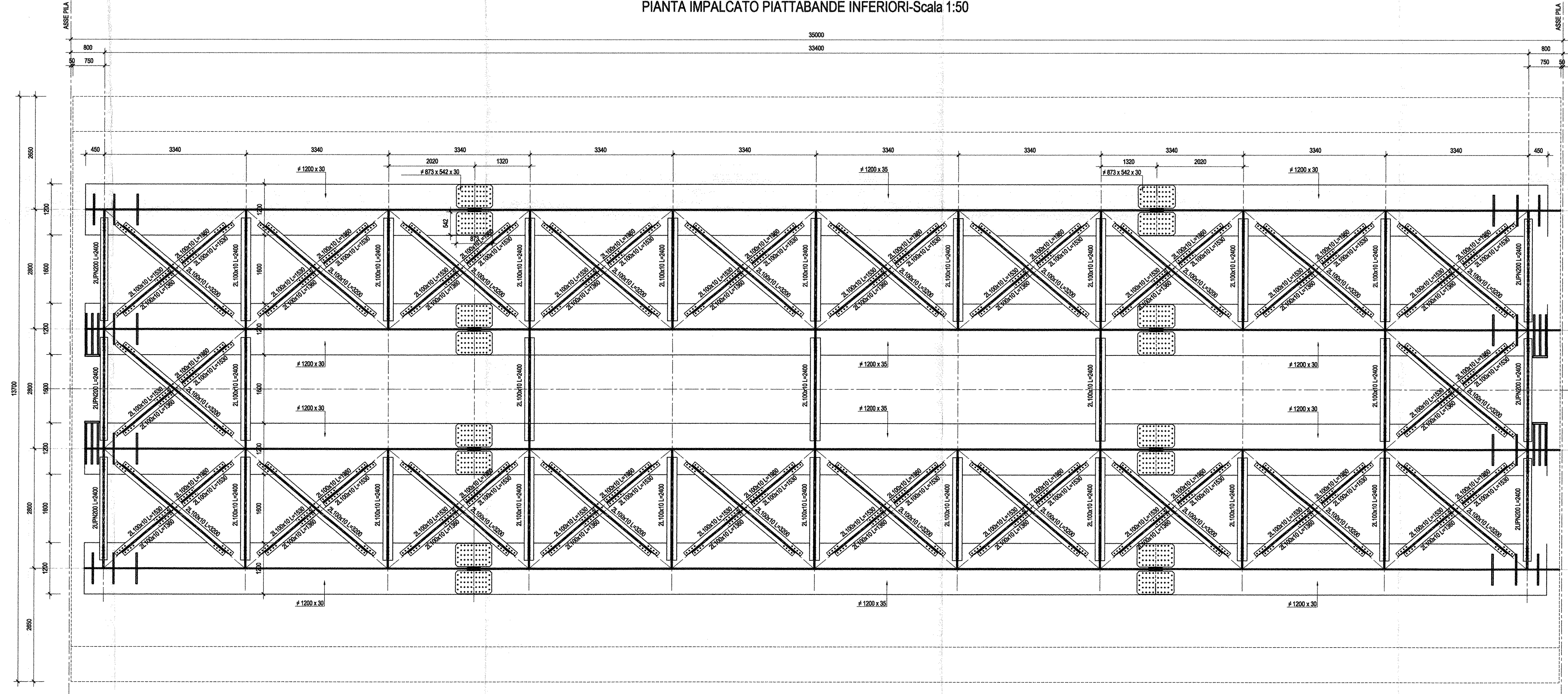
PIANTA IMPALCATO PIATTABANDE INFERIORI-Scala 1:50
