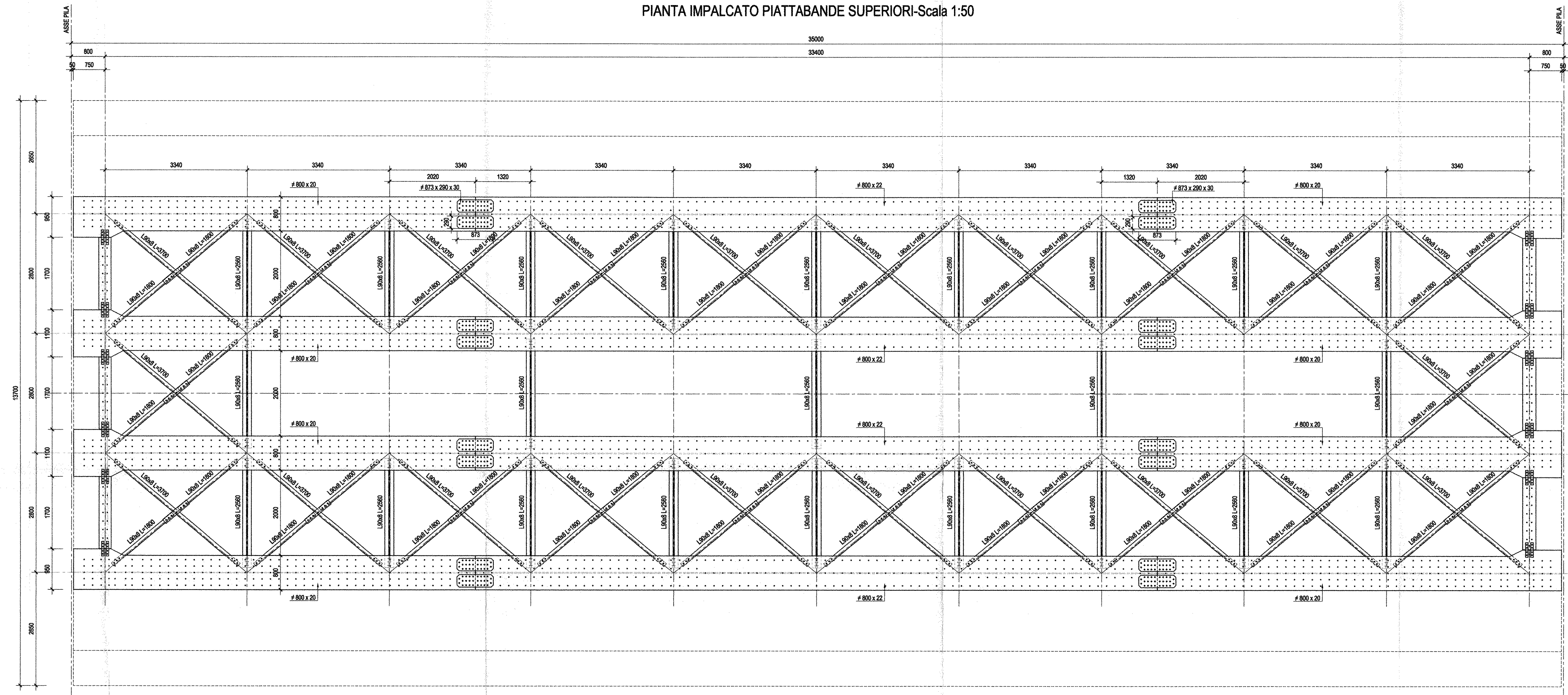
PIANTA IMPALCATO PIATTABANDE SUPERIORI-Scala 1:50
