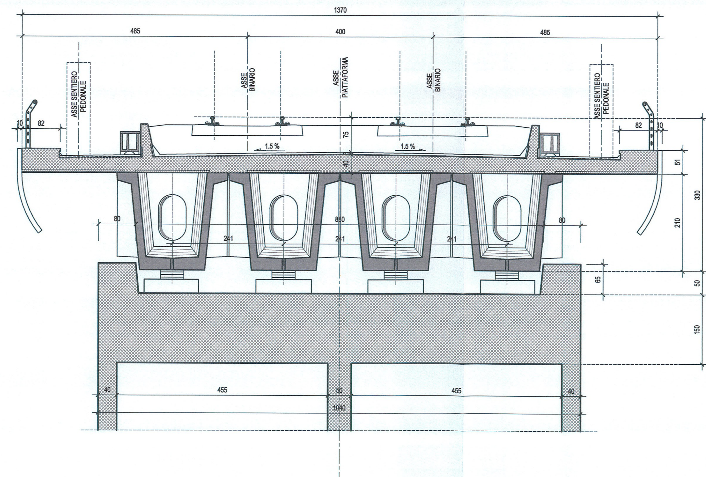
SEZIONE TIPO IN ASSE APPOGGIO-Scala 1:50
