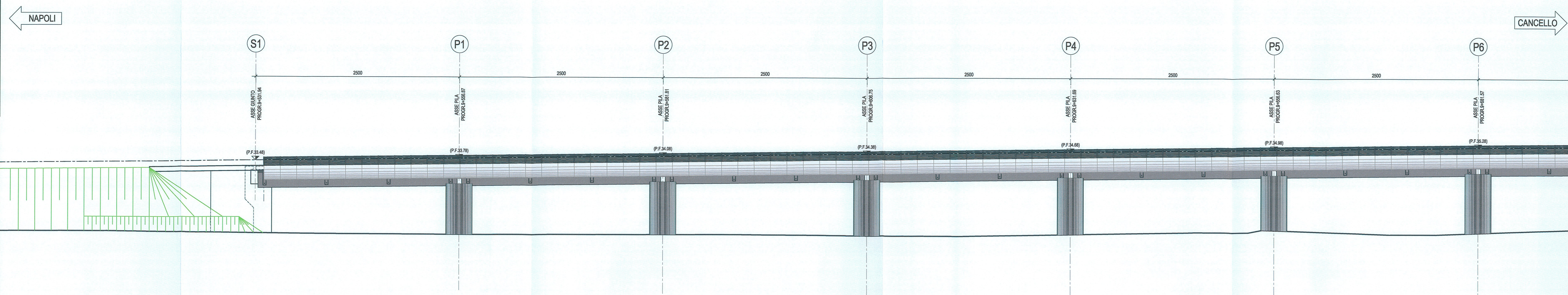
PIANTA IMPALCATO-Scala 1:200
