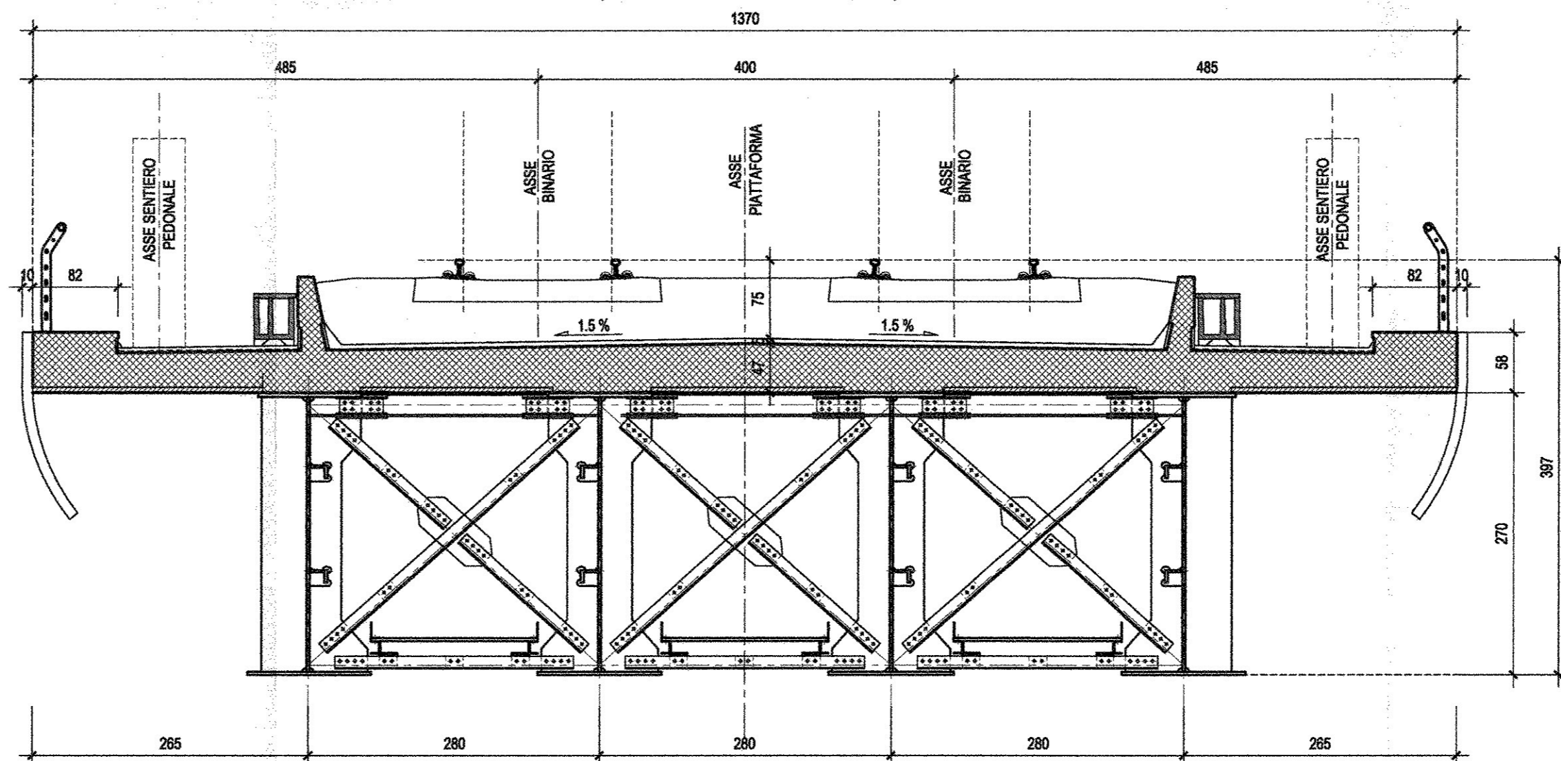
SEZIONE TIPO IN CAMPATA-Scala 1:50 (CAMPATA IN ACCIAIO PILE P8-P10)
