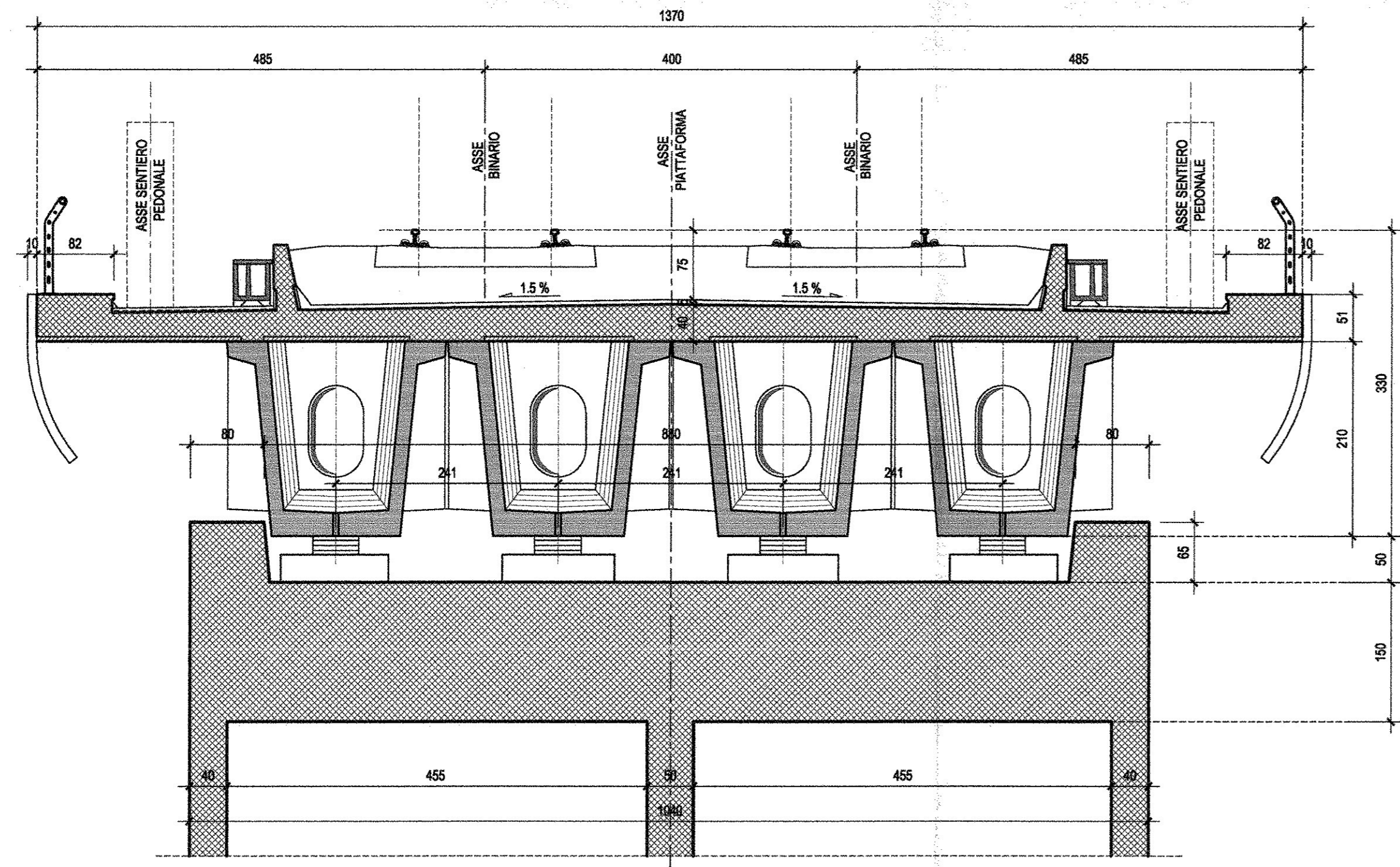
SEZIONE TIPO IN ASSE APPOGGIO-Scala 1:50
