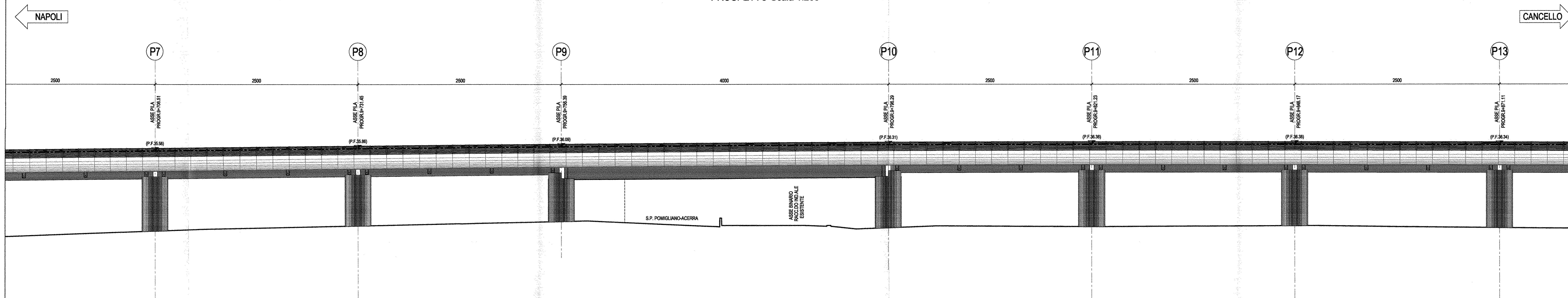
PIANTA IMPALCATO-Scala 1:200
