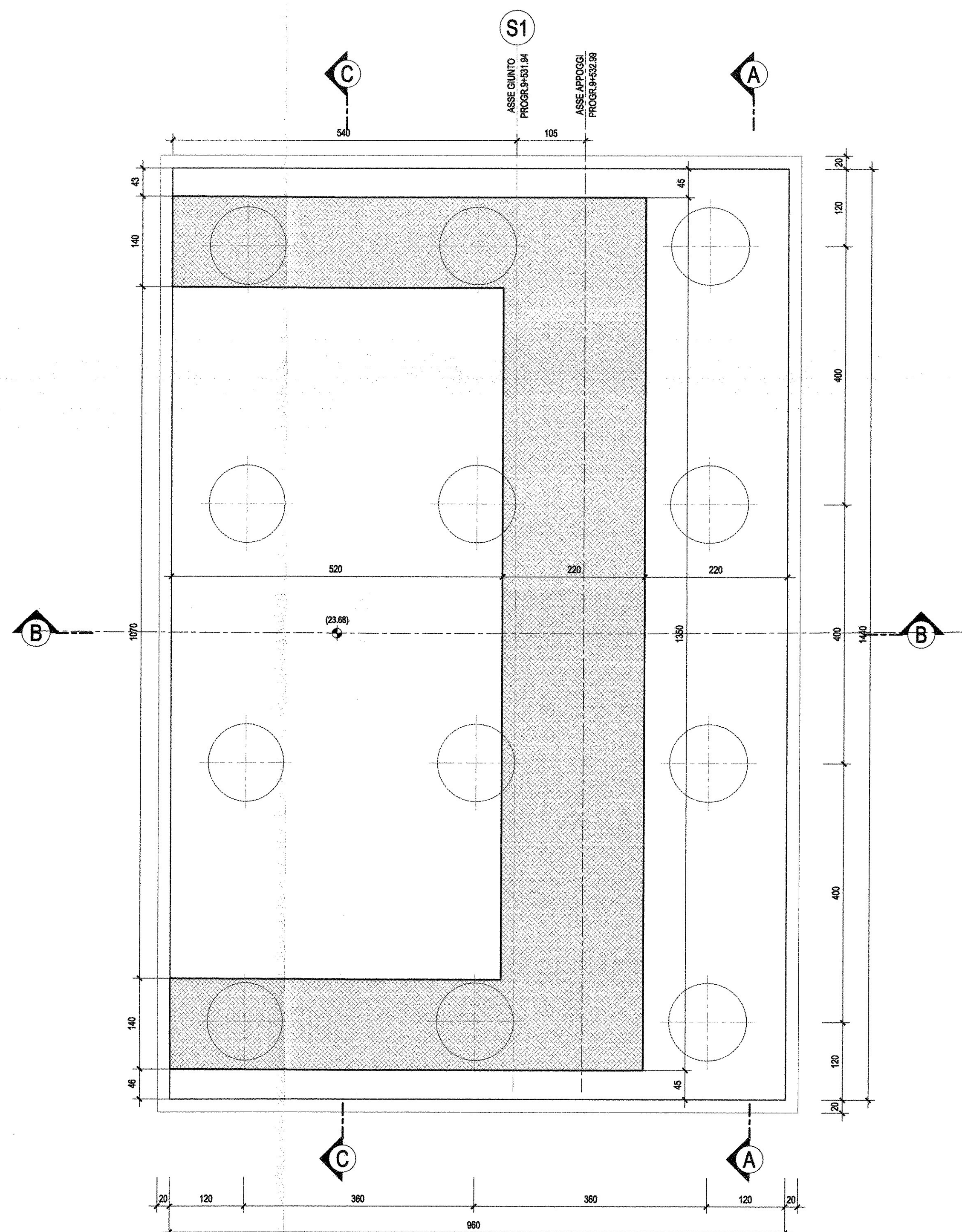
SEZIONE D-D-Scala 1:50
