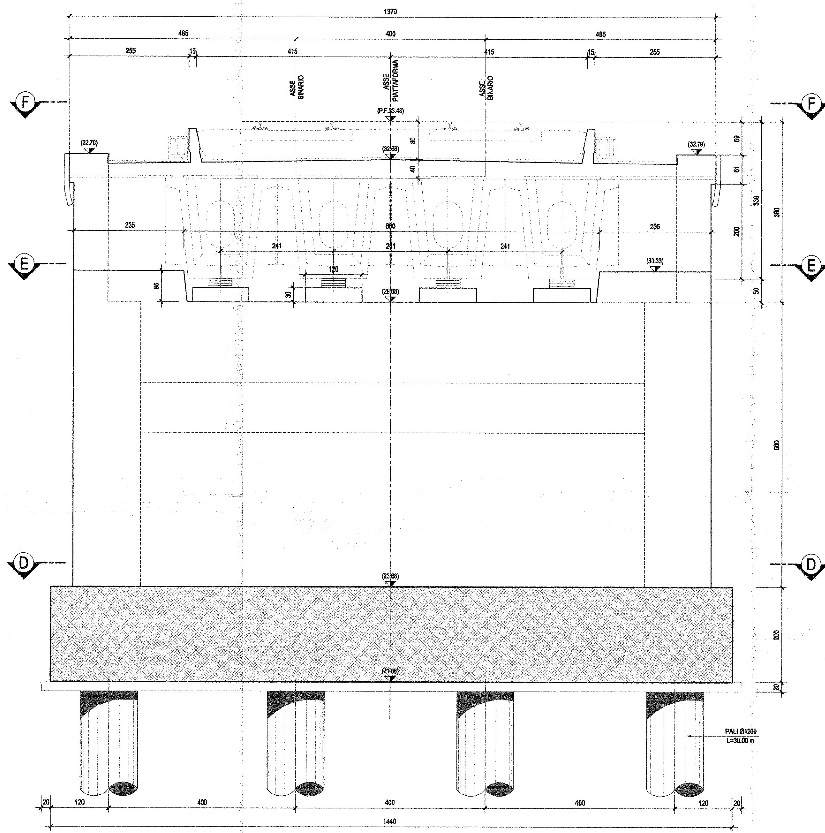
SEZIONE A-A-Scala 1:50
