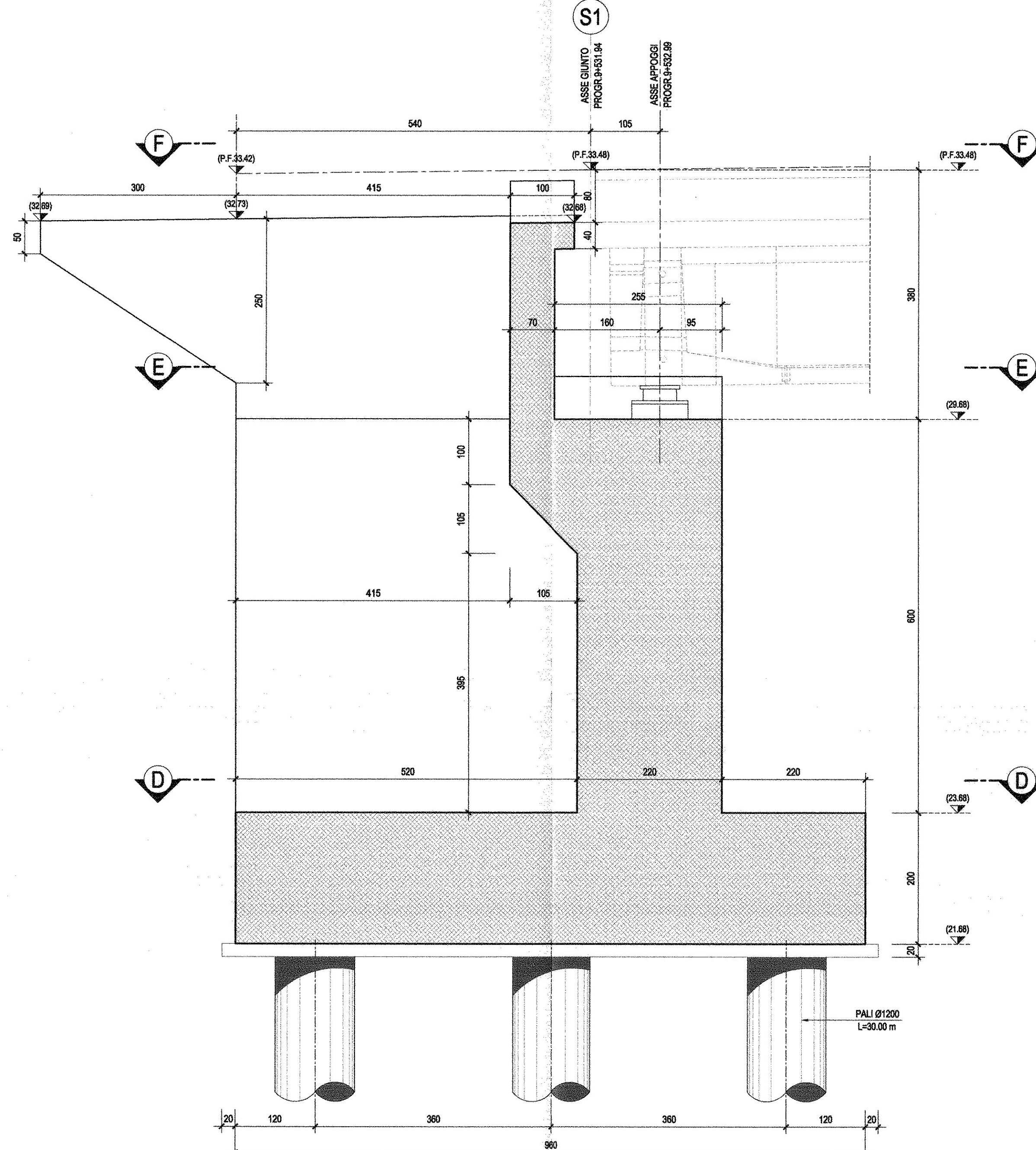
SEZIONE B-B-Scala 1:50
