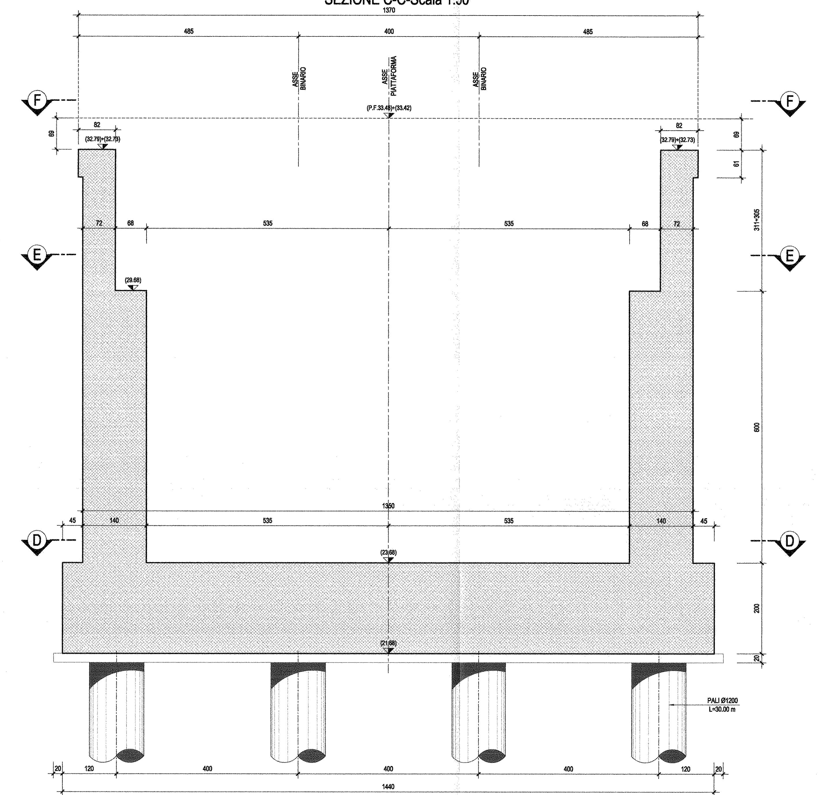
SEZIONE C-C-Scala 1:50
