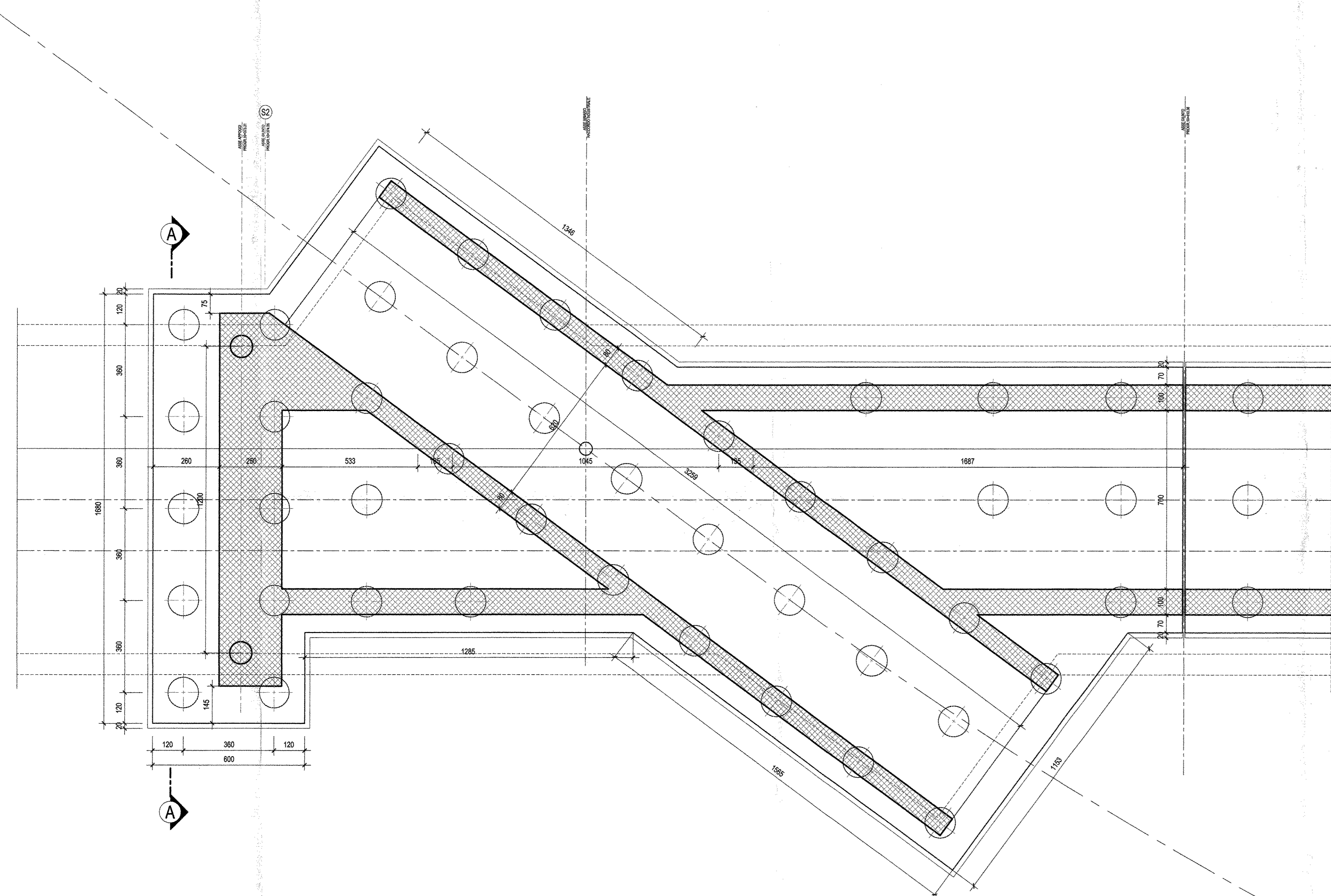
SEZIONE D-D-Scala 1:100
