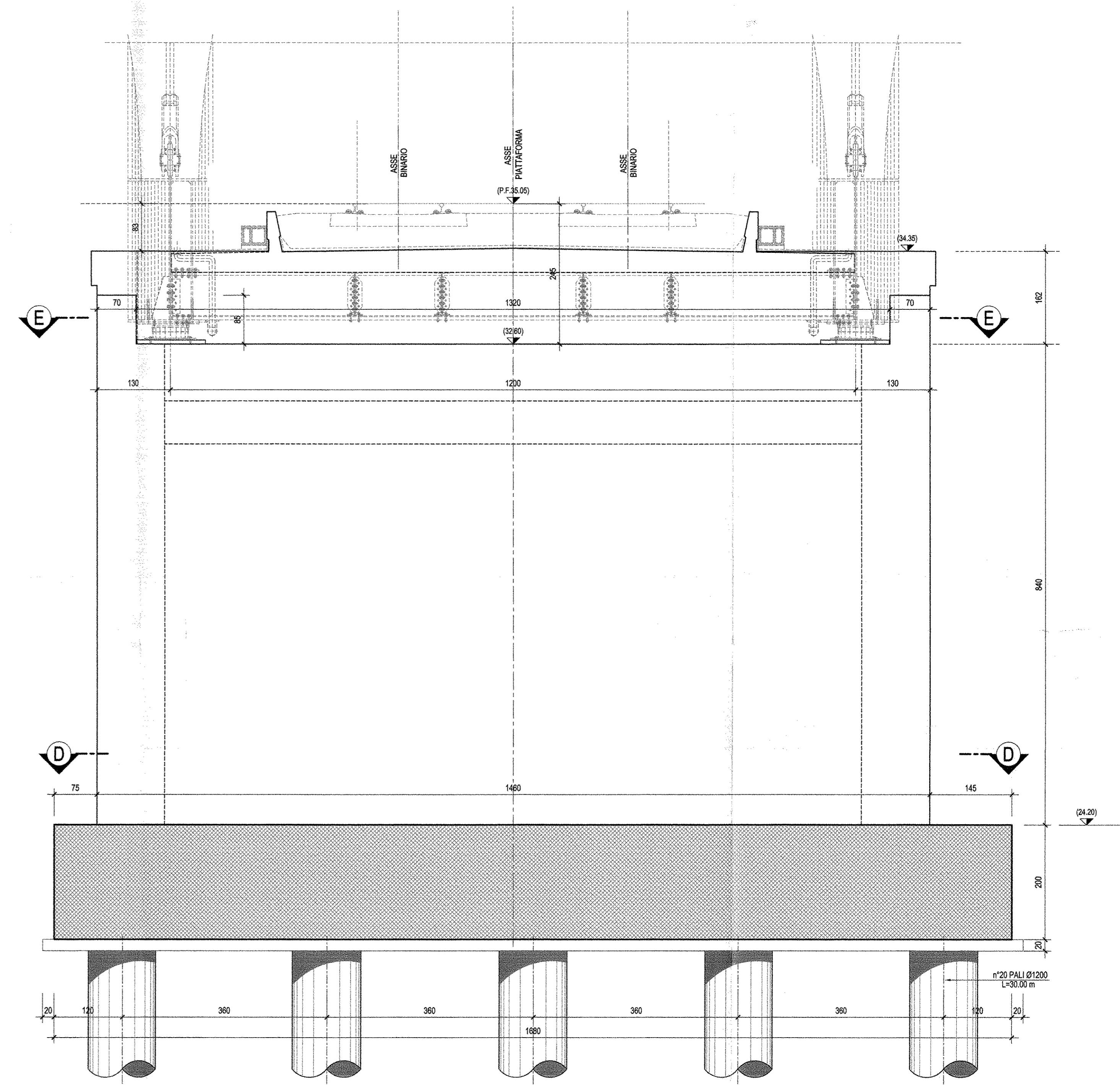
SEZIONE A-A-Scala 1:50
