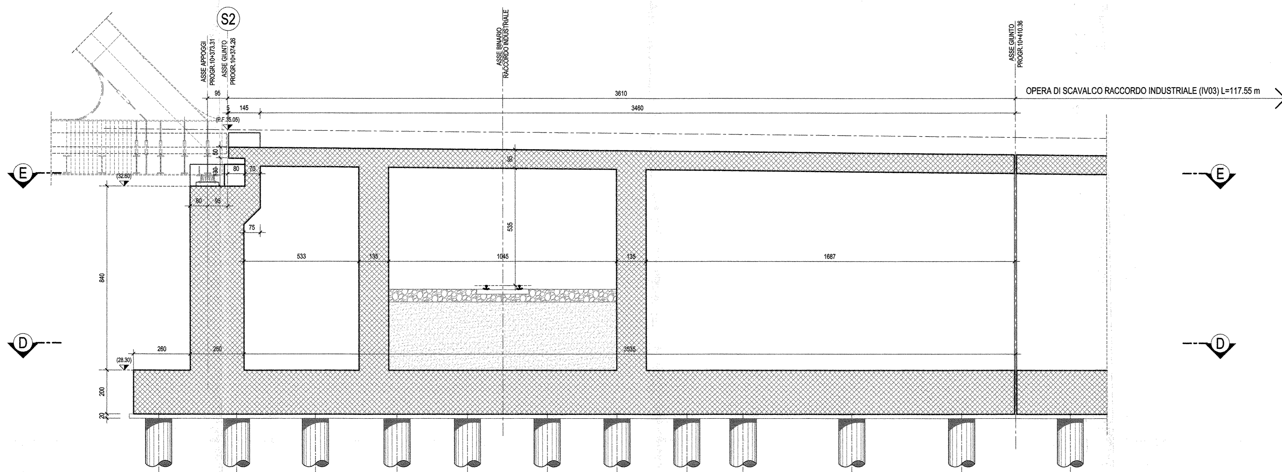
SEZIONE LONGITUDINALE-Scala 1:100
