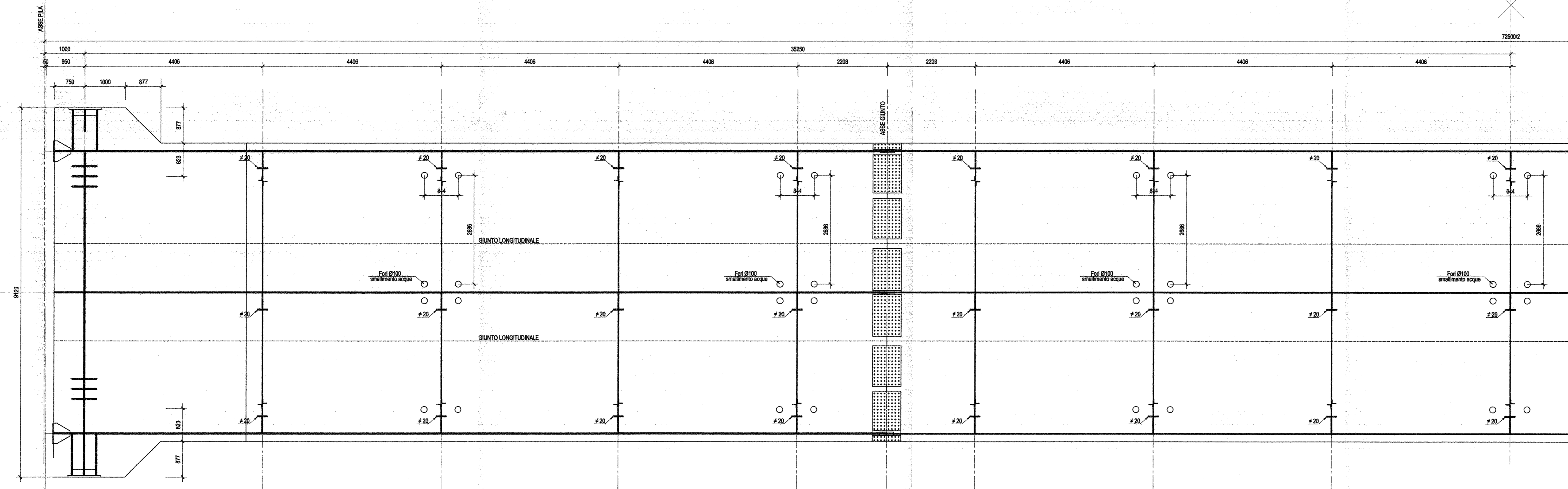
1/2 PIANTA PIATTABANDE INFERIORI TRAVE-Scala 1:50
