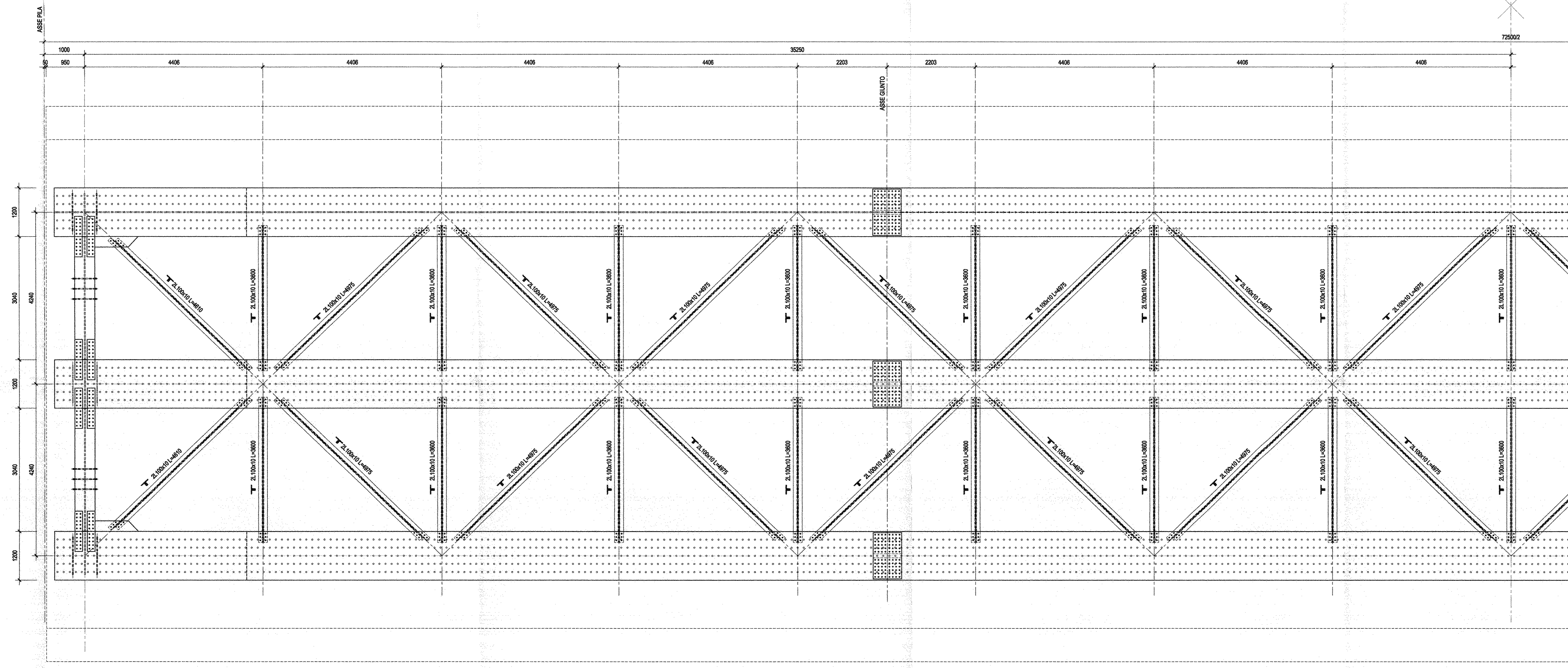
1/2 PIANTA PIATTABANDE SUPERIORI TRAVE-Scala 1:50
