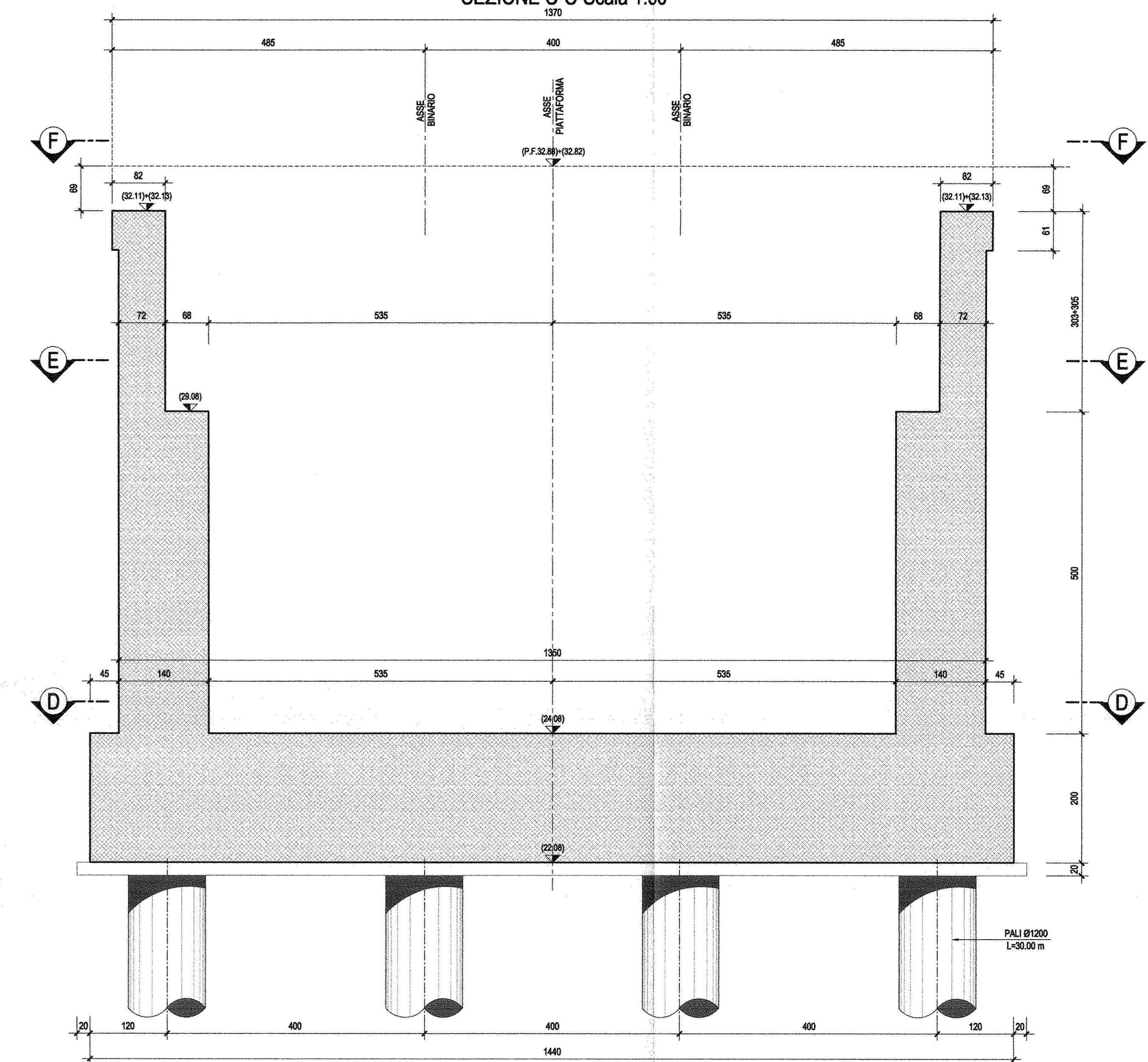
SEZIONE C-C-Scala 1:50
