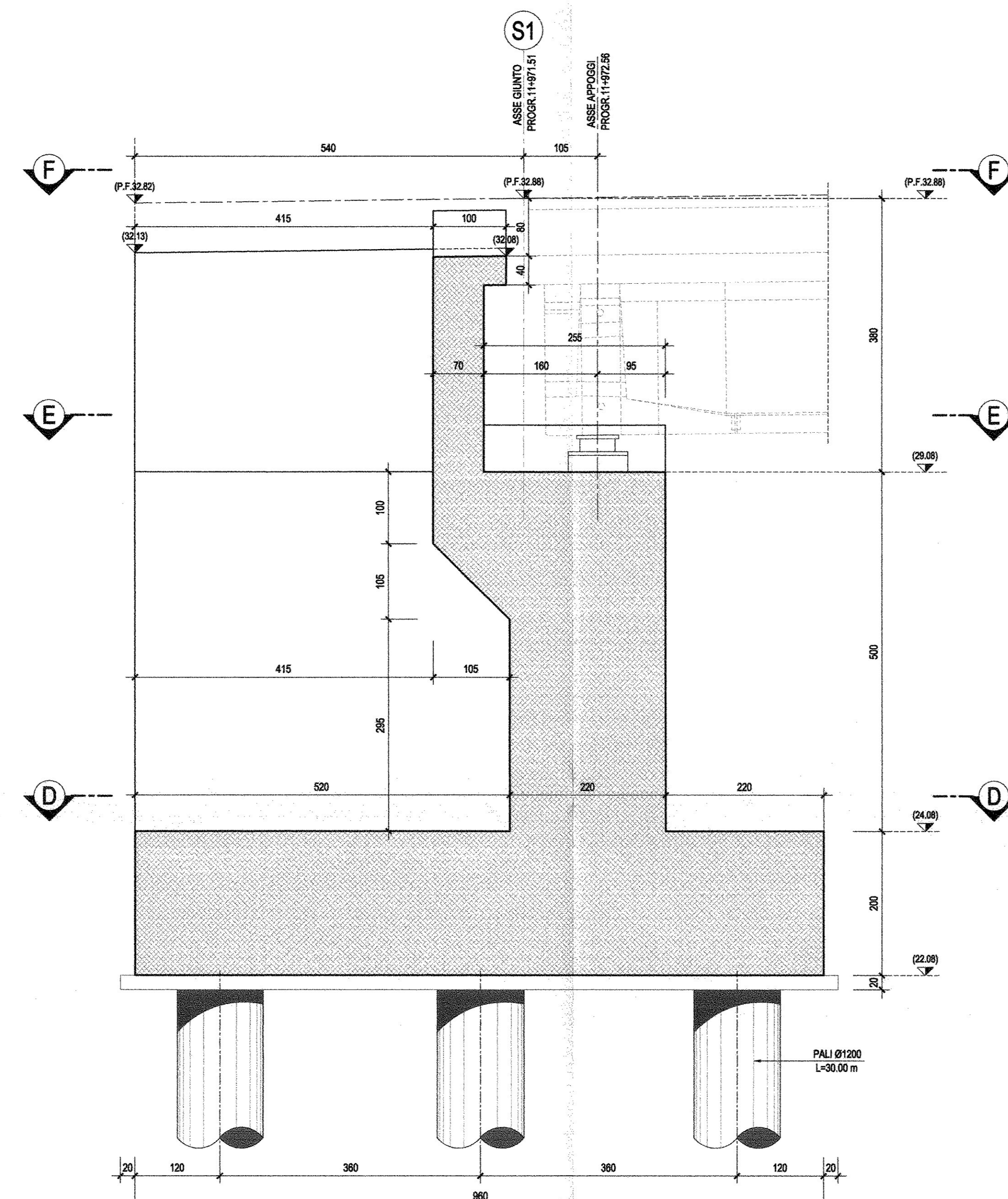
SEZIONE B-B-Scala 1:50
