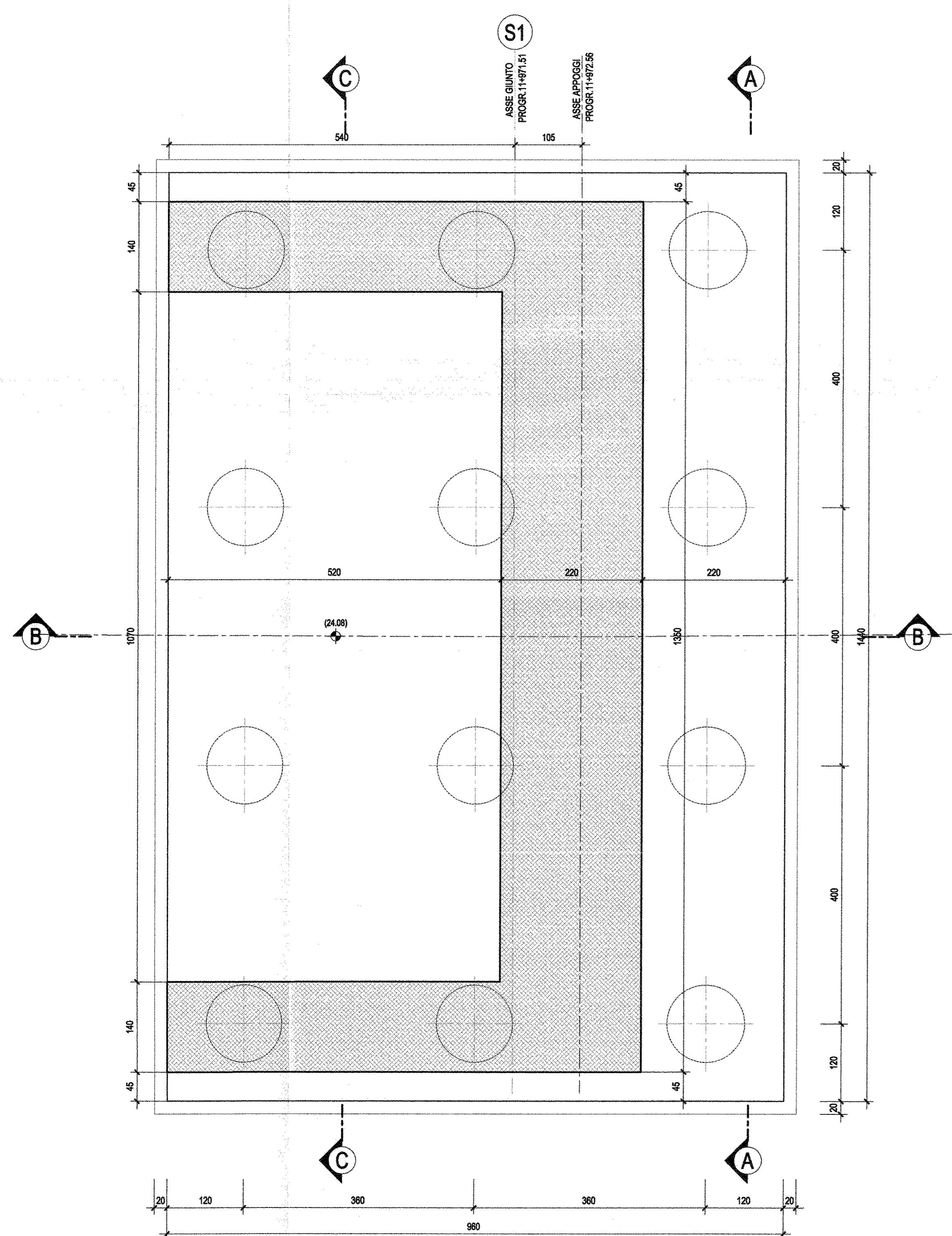
SEZIONE D-D-Scala 1:50
