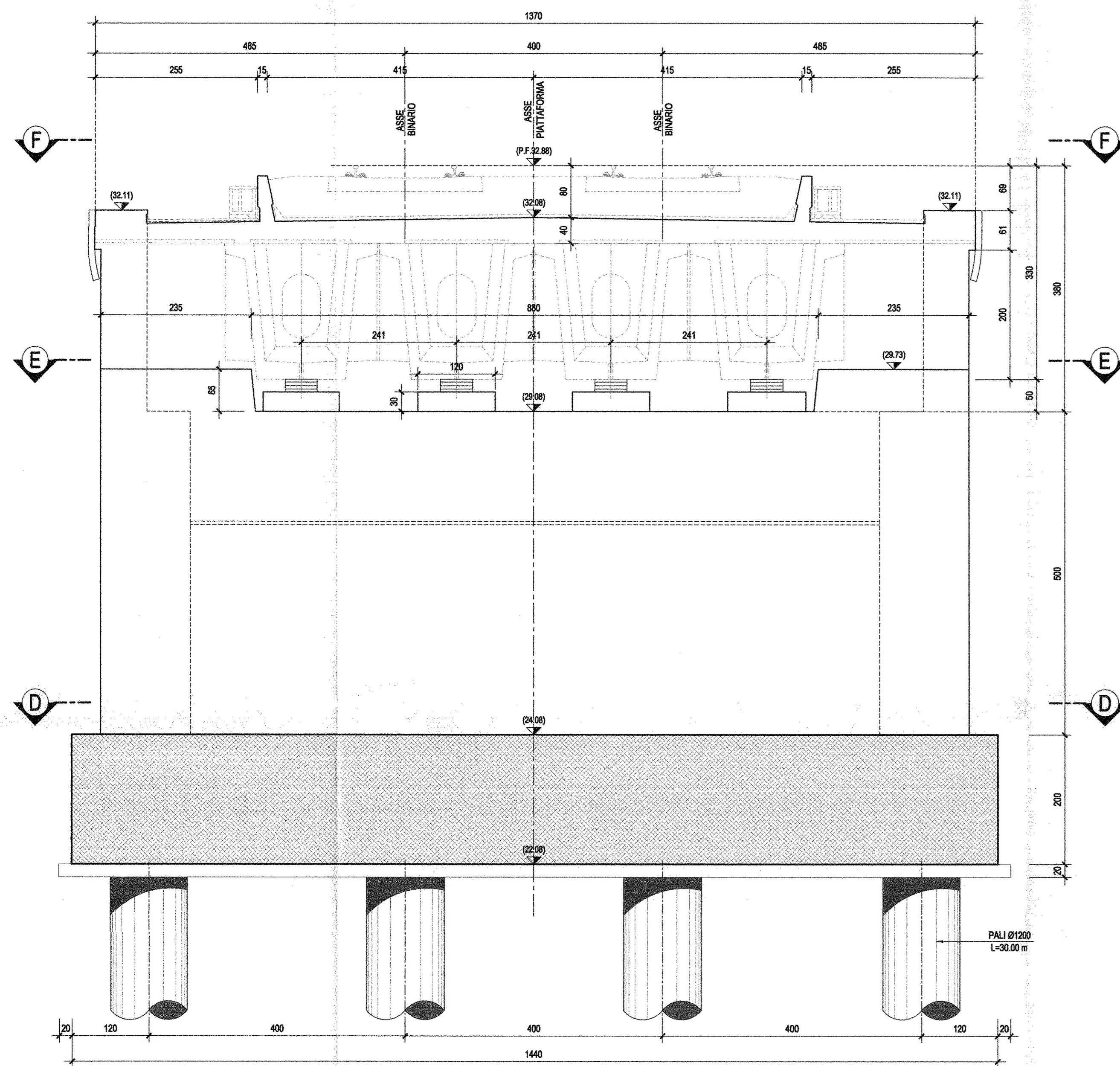
SEZIONE A-A-Scala 1:50
