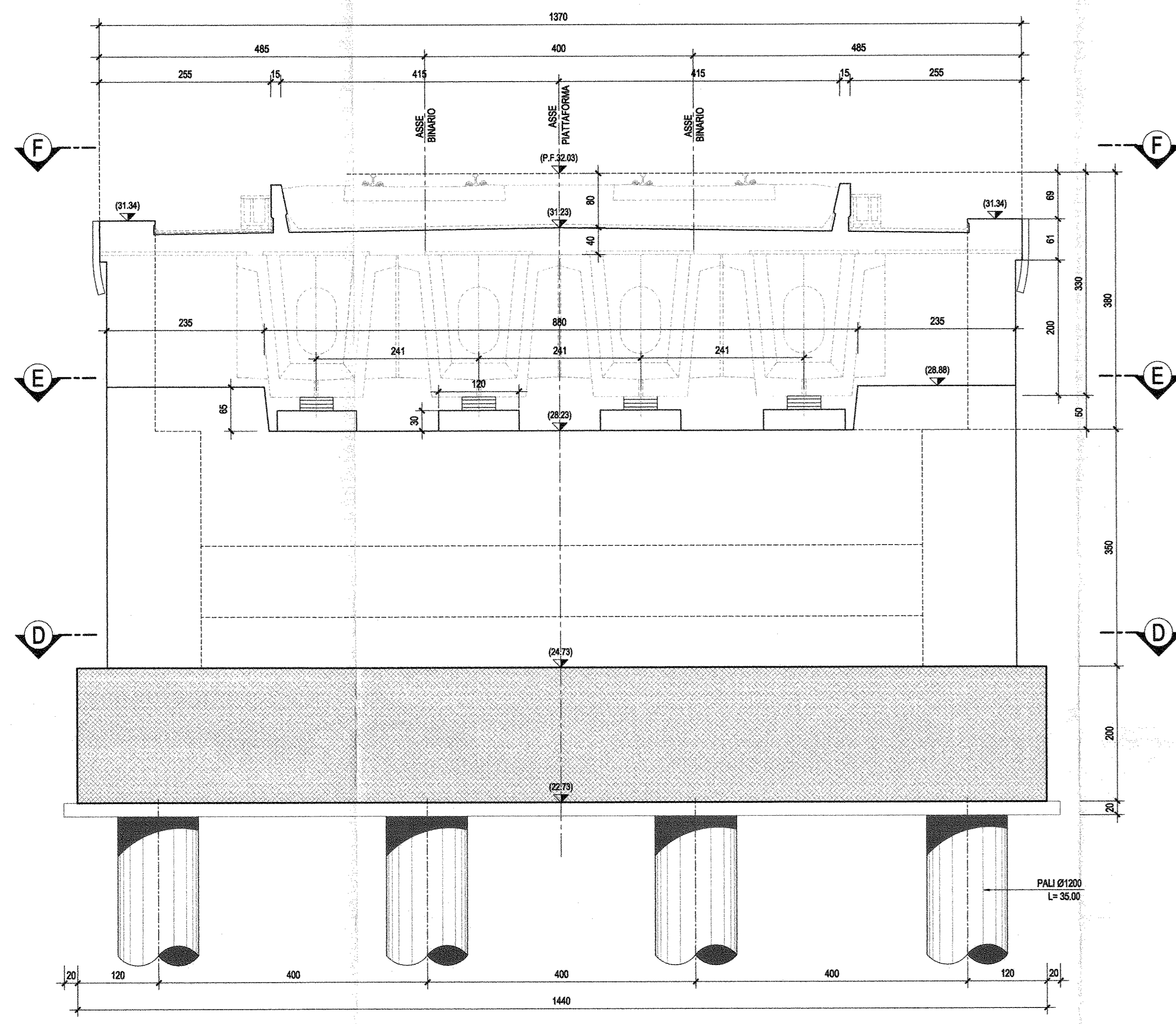
SEZIONE A-A-Scala 1:50
