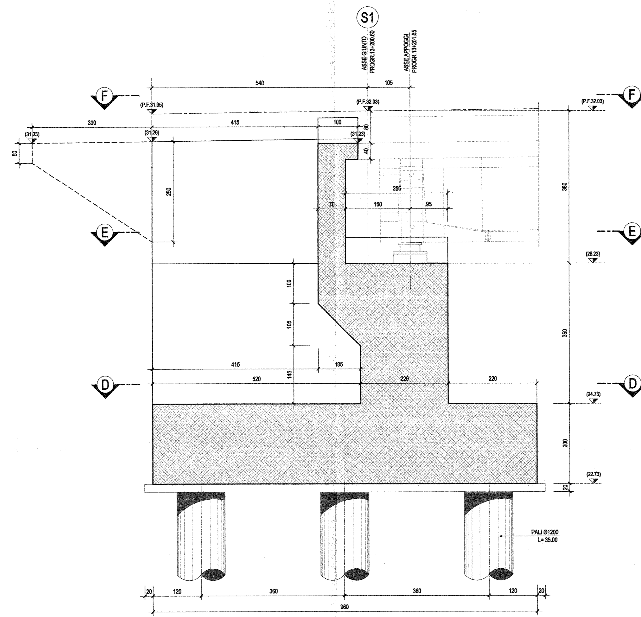
SEZIONE B-B-Scala 1:50
