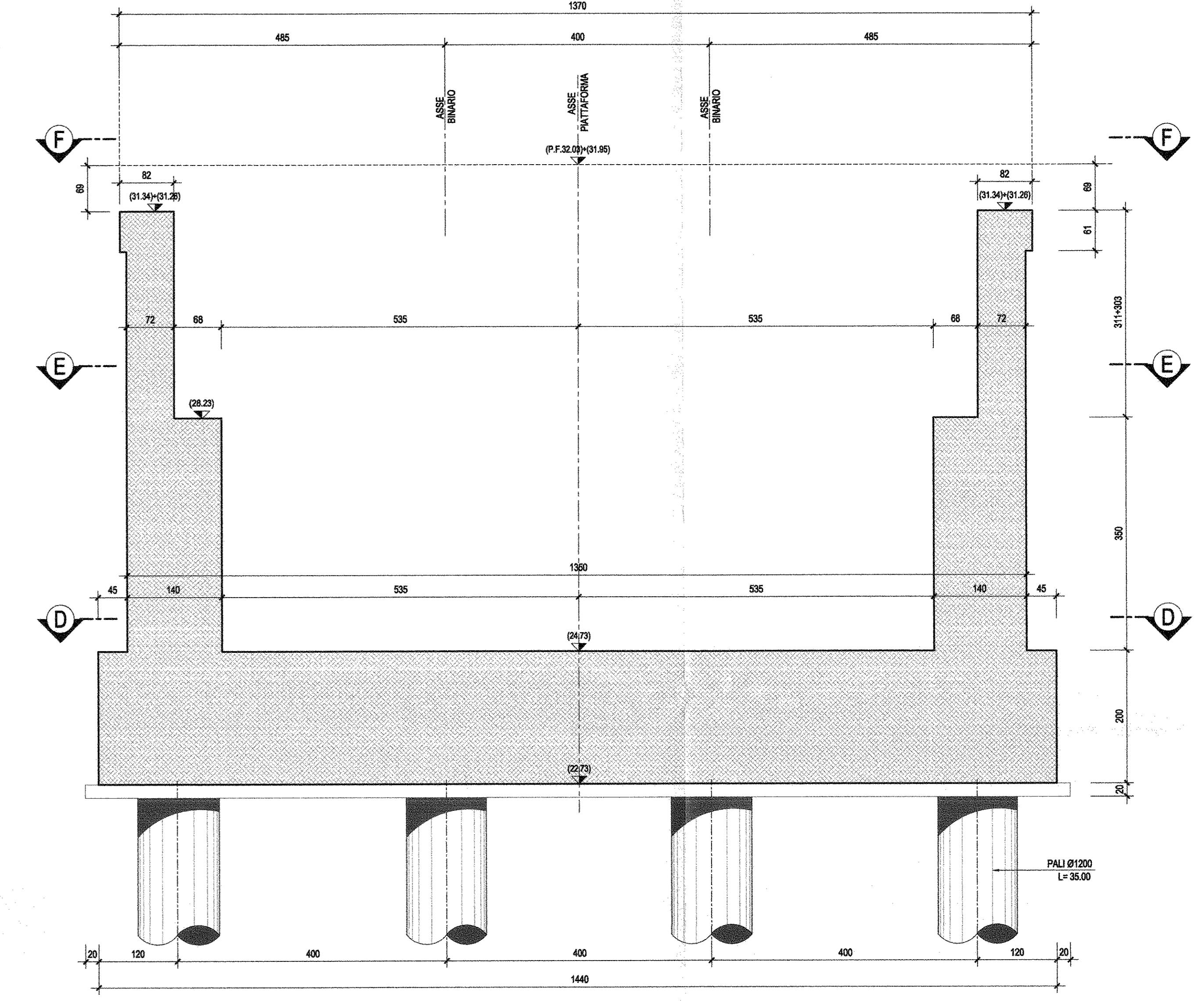
SEZIONE C-C-Scala 1:50
