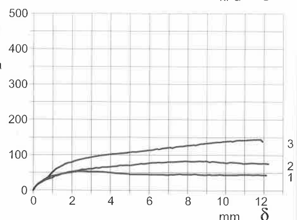
DIAGRAMMA Tensione - Deformaz. orizz.
