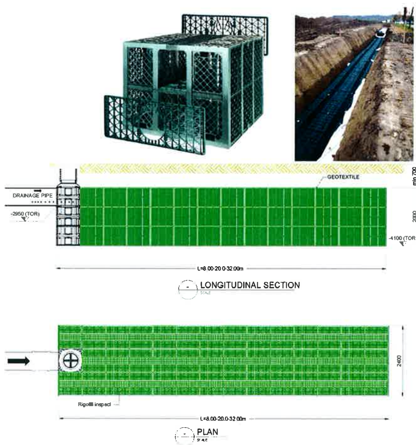
Figura 6 – Tipologico di trincea drenante con moduli in materiale plastico
