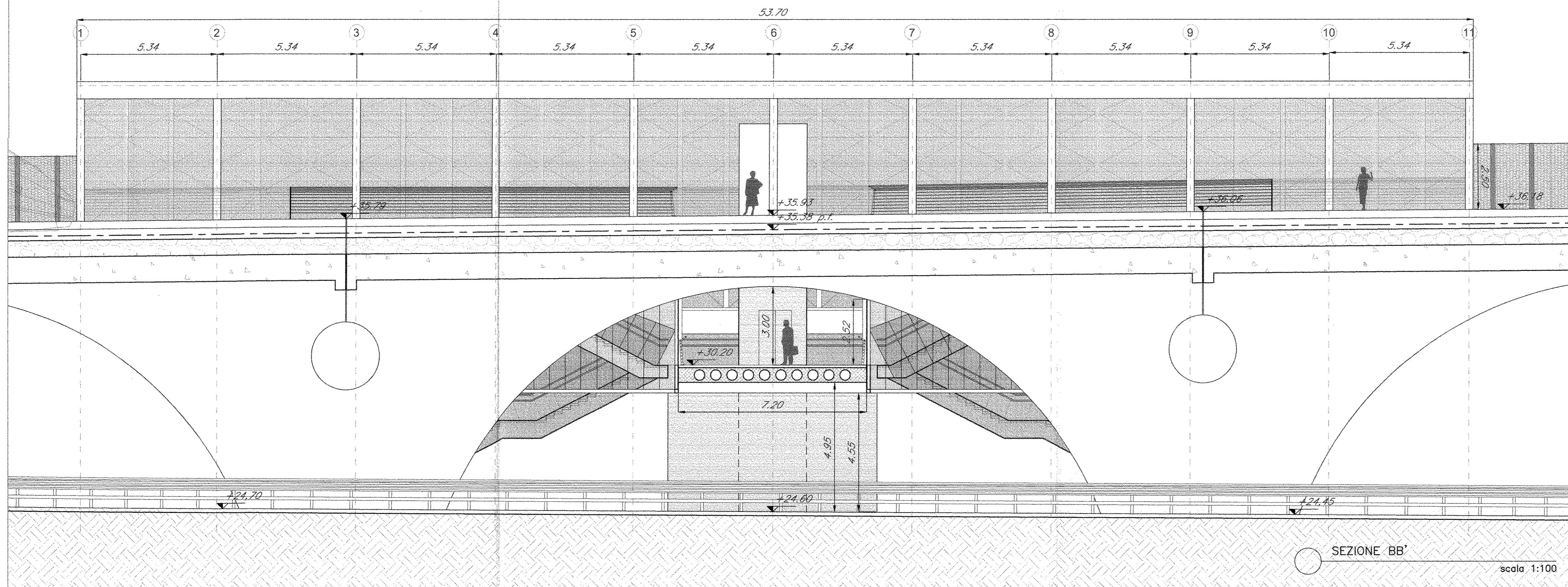
PIANTA QUOTA MEZZANINO scala 1:100
