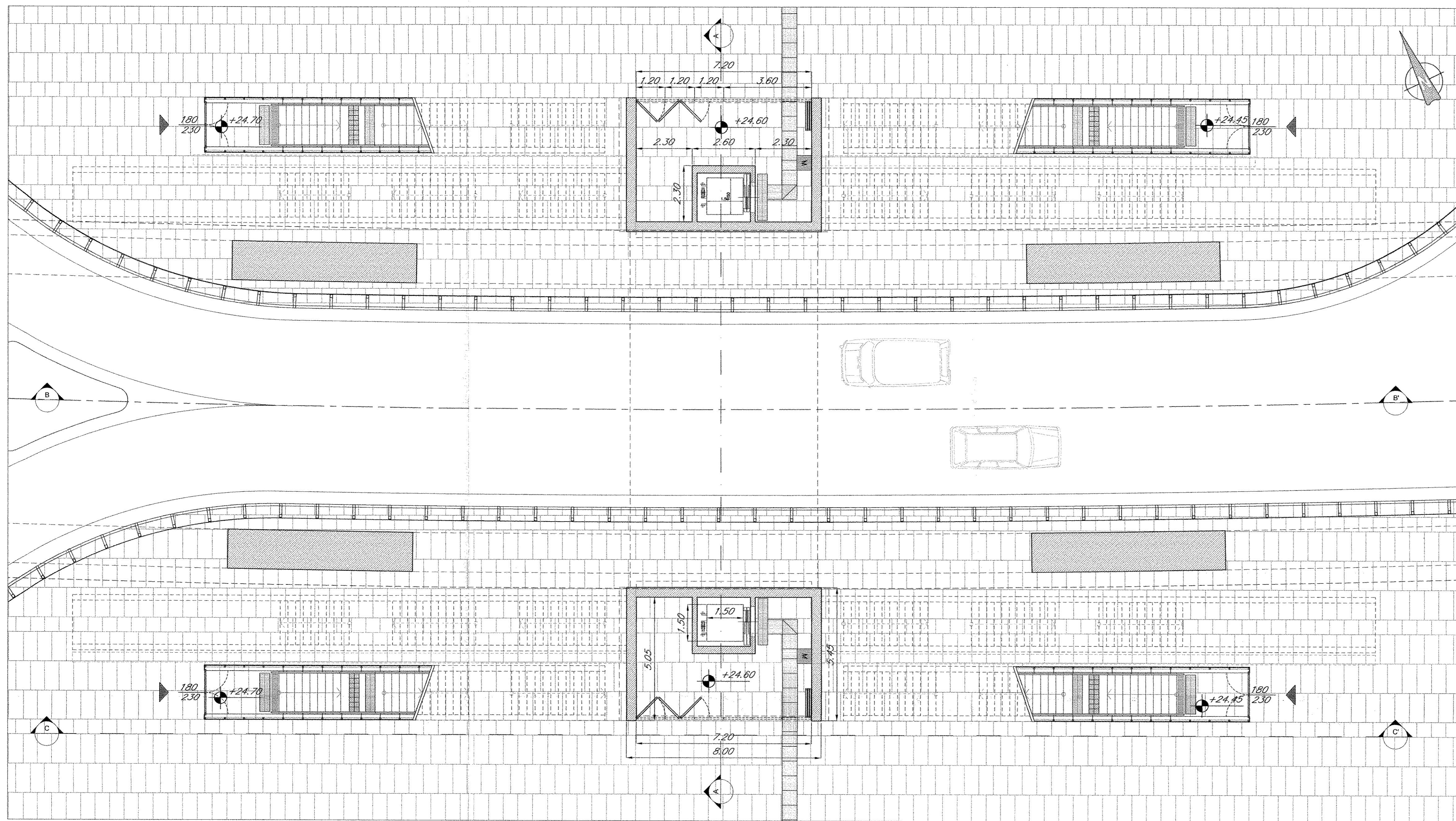
PIANTA QUOTA STRADA scala 1:100
