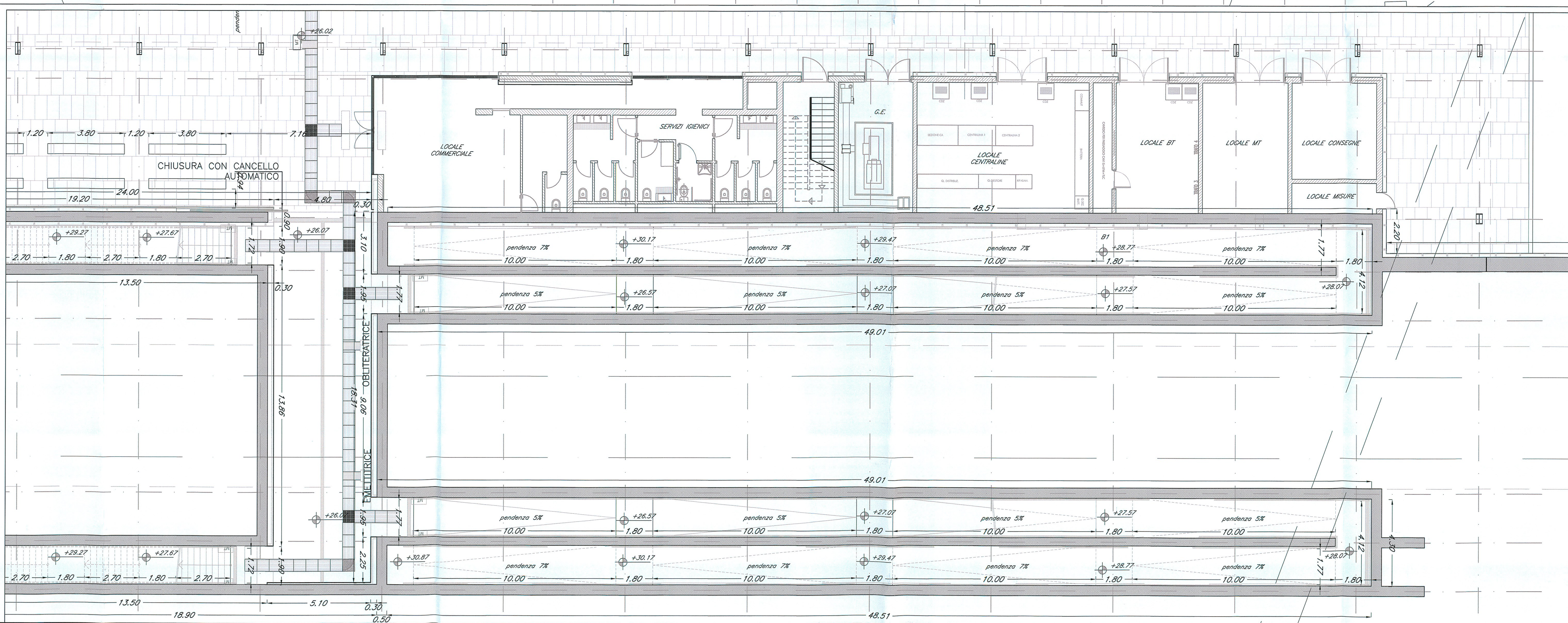
1 PIANTE SOTTOPASSO POST OPERAM scala 1:100
