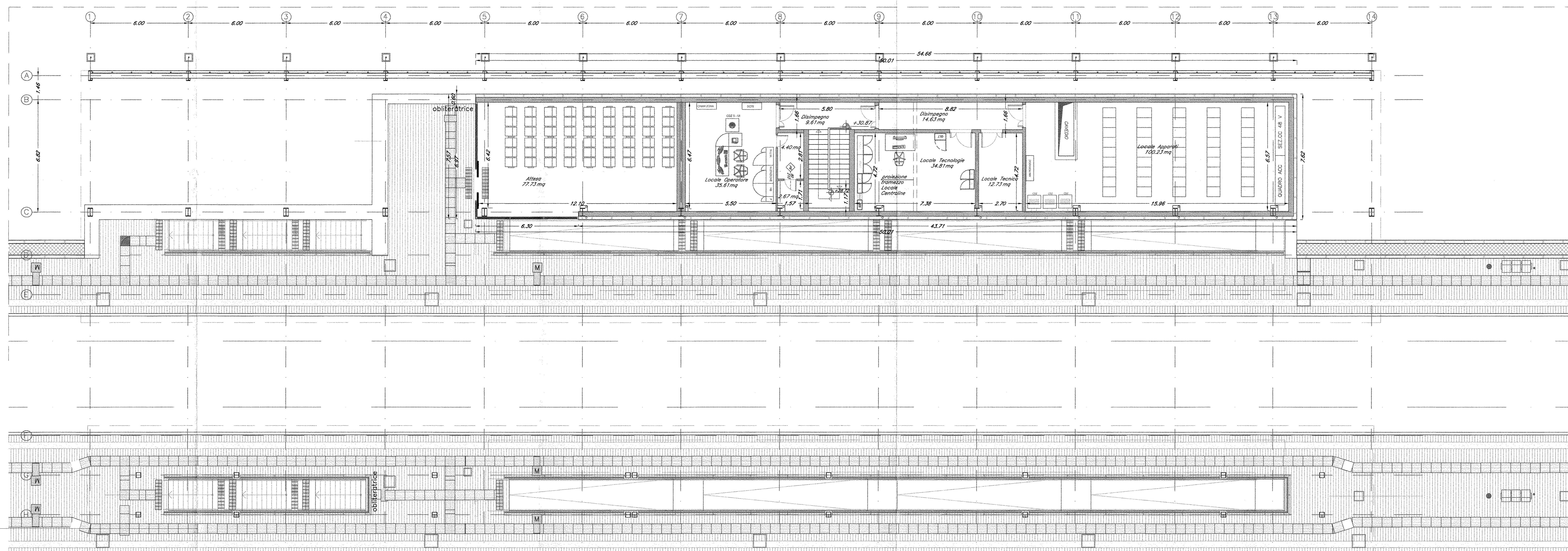
PIANTA FT QUOTA SOTTOPASSO POST OPERAM scala 1:100
