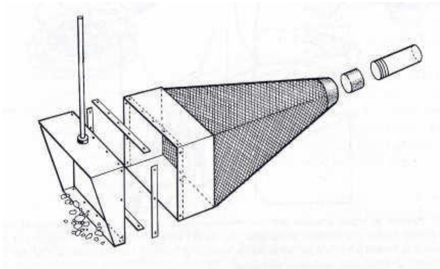
Figura 4.2.3. Schema del retino da campionamento.
