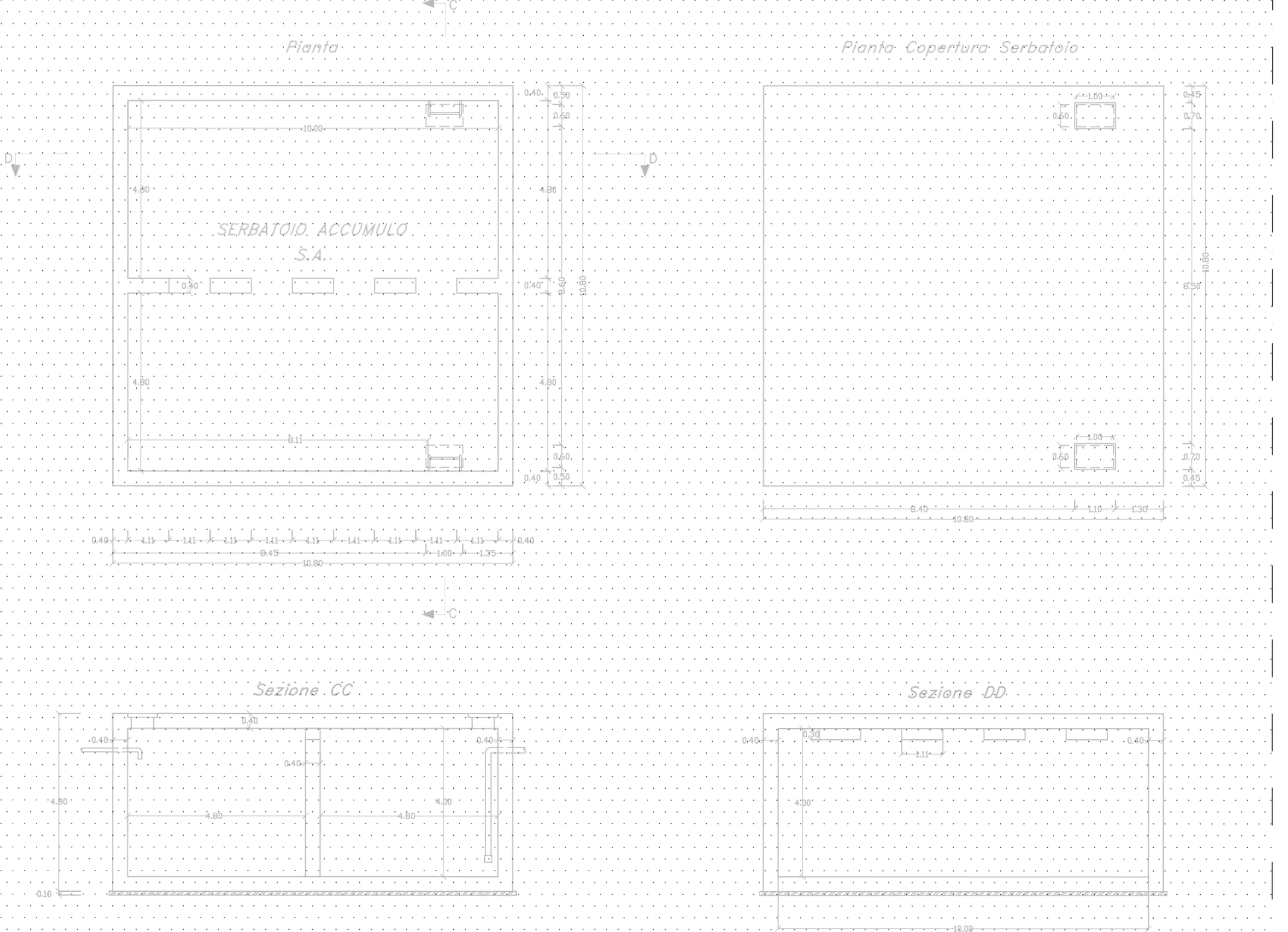
PARTIGOLARE ARCHITETTONICO DELLA VASCA DI ACCUMULO scala 1:100
