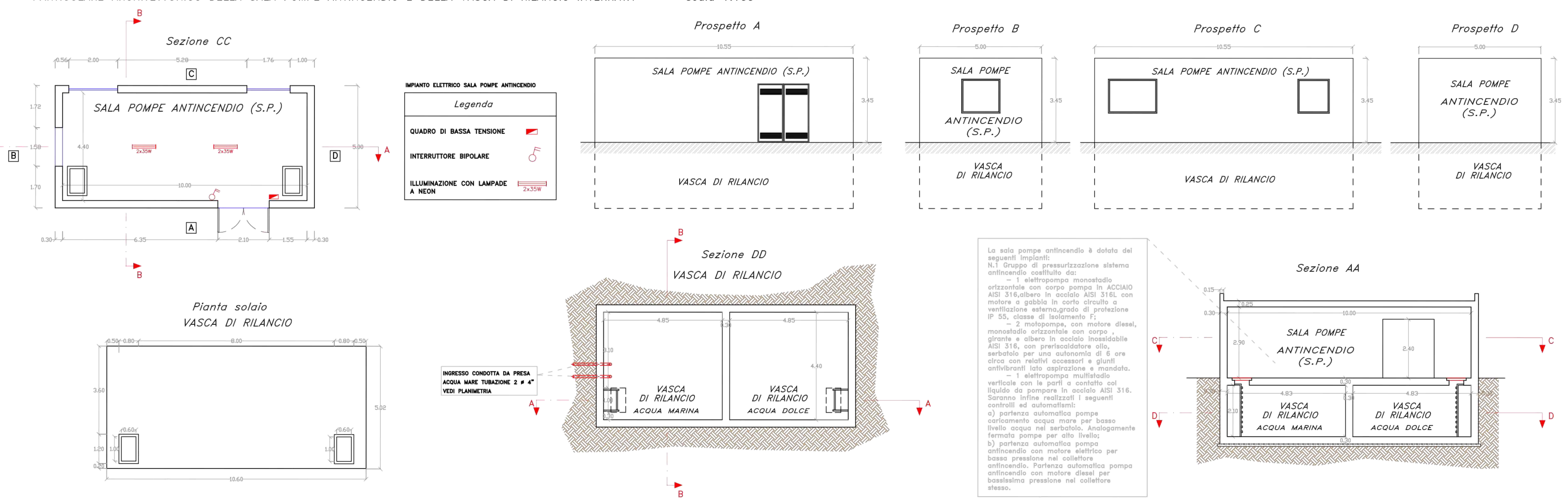
PARTIGOLARE ARCHITETTONICO DELLA SALA POMPE ANTINCENDIO E DELLA VASCA DI RILANCIO INTERRATA scala 1:100
