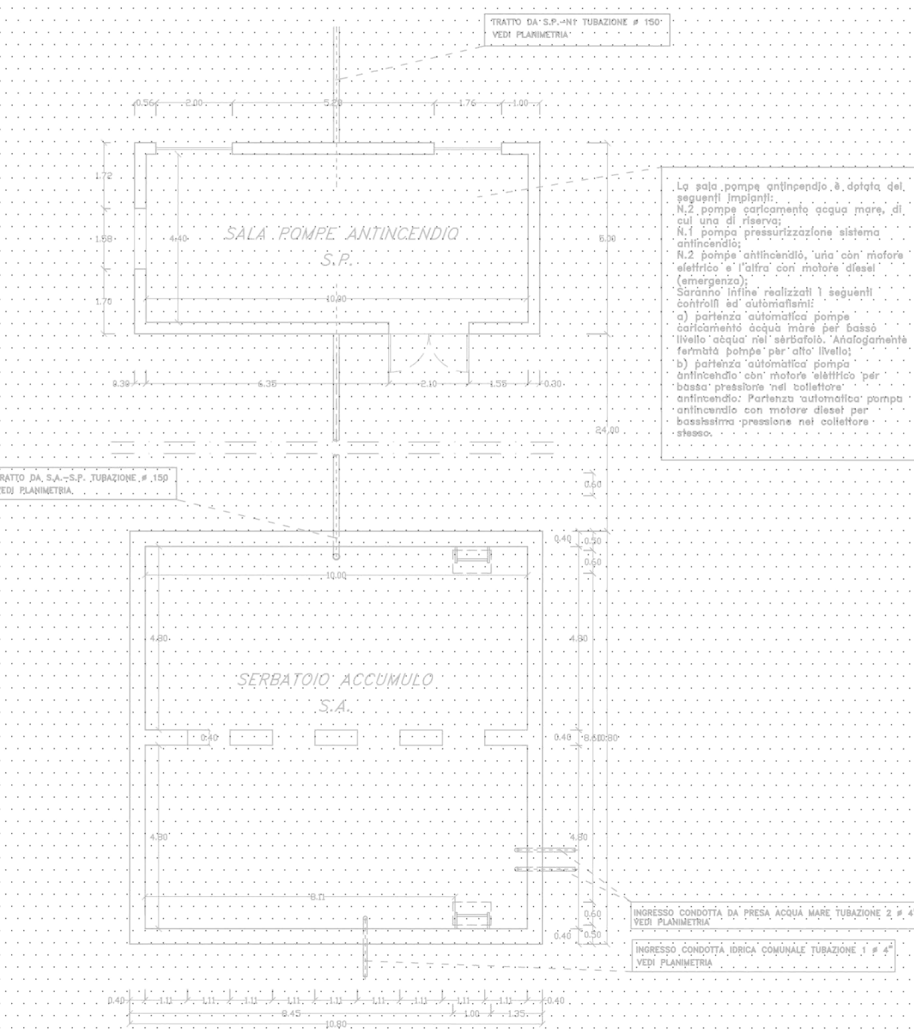
PARTIGOLARE ARCHITETTONICO DELLA SALA POMPE ANTINCENDIO E DELLA VASCA DI RILANCIO INTERRATA scala 1:100
