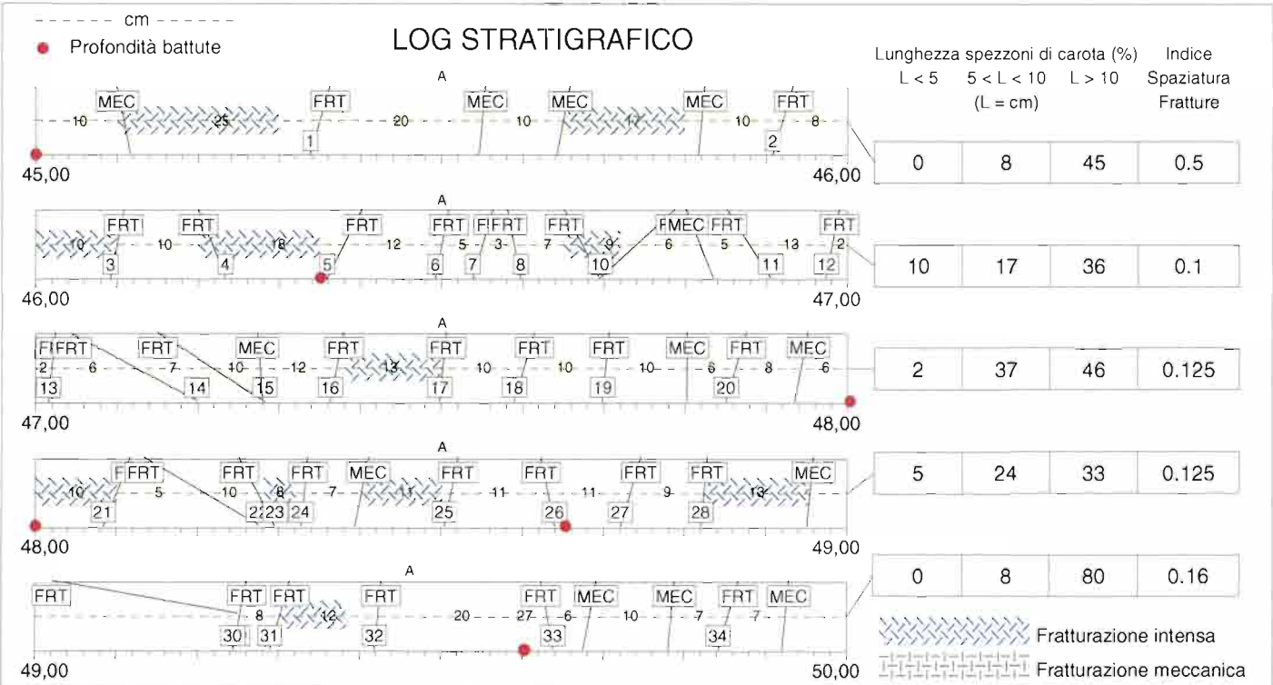
sondaggio CBV13 - cassetta n°10
