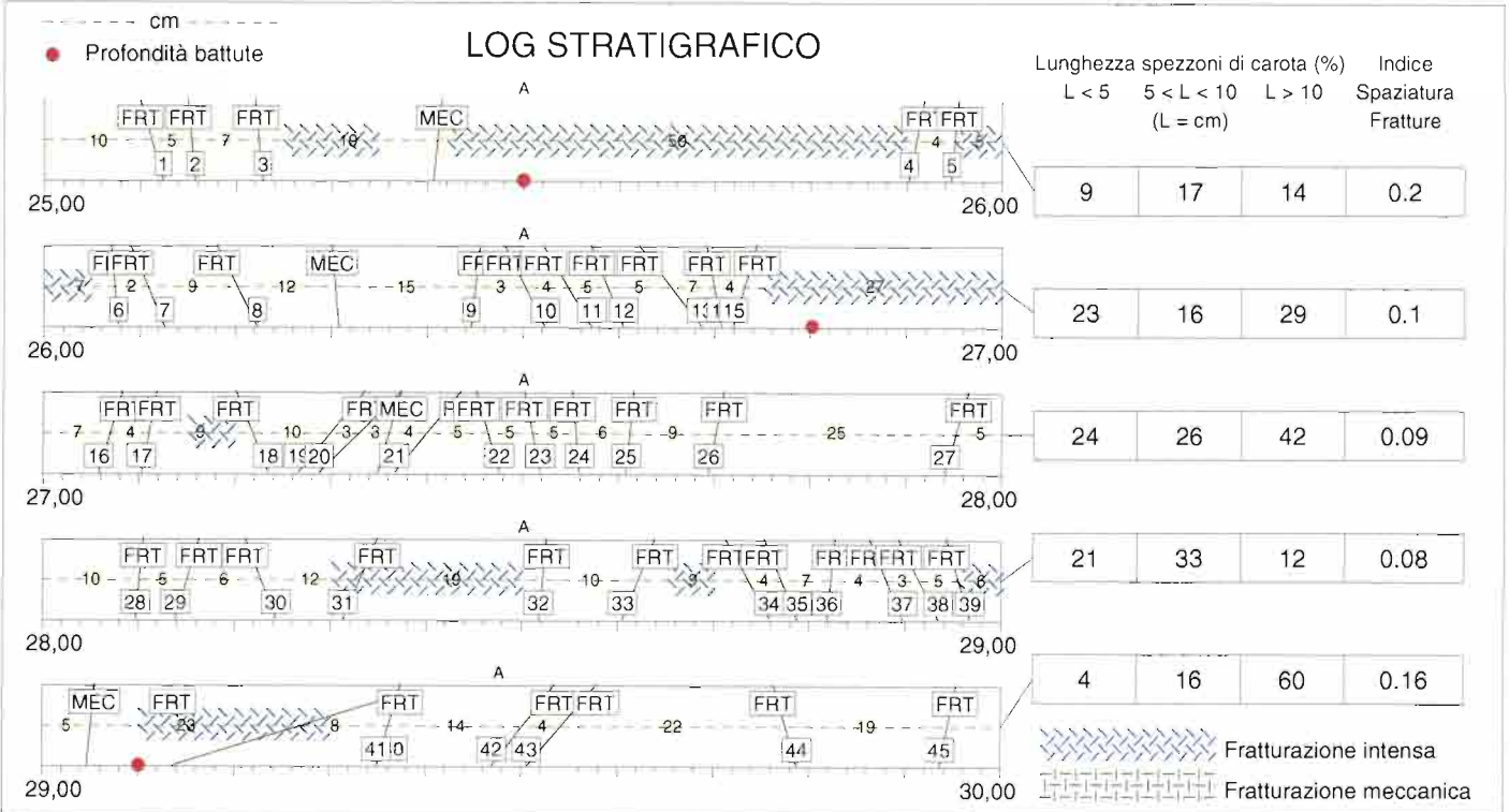
sondaggio C 27 - cassetta 6
