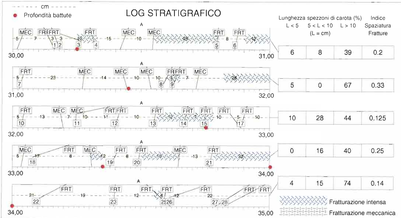
sondaggio CBV13 - cassetta n°7
