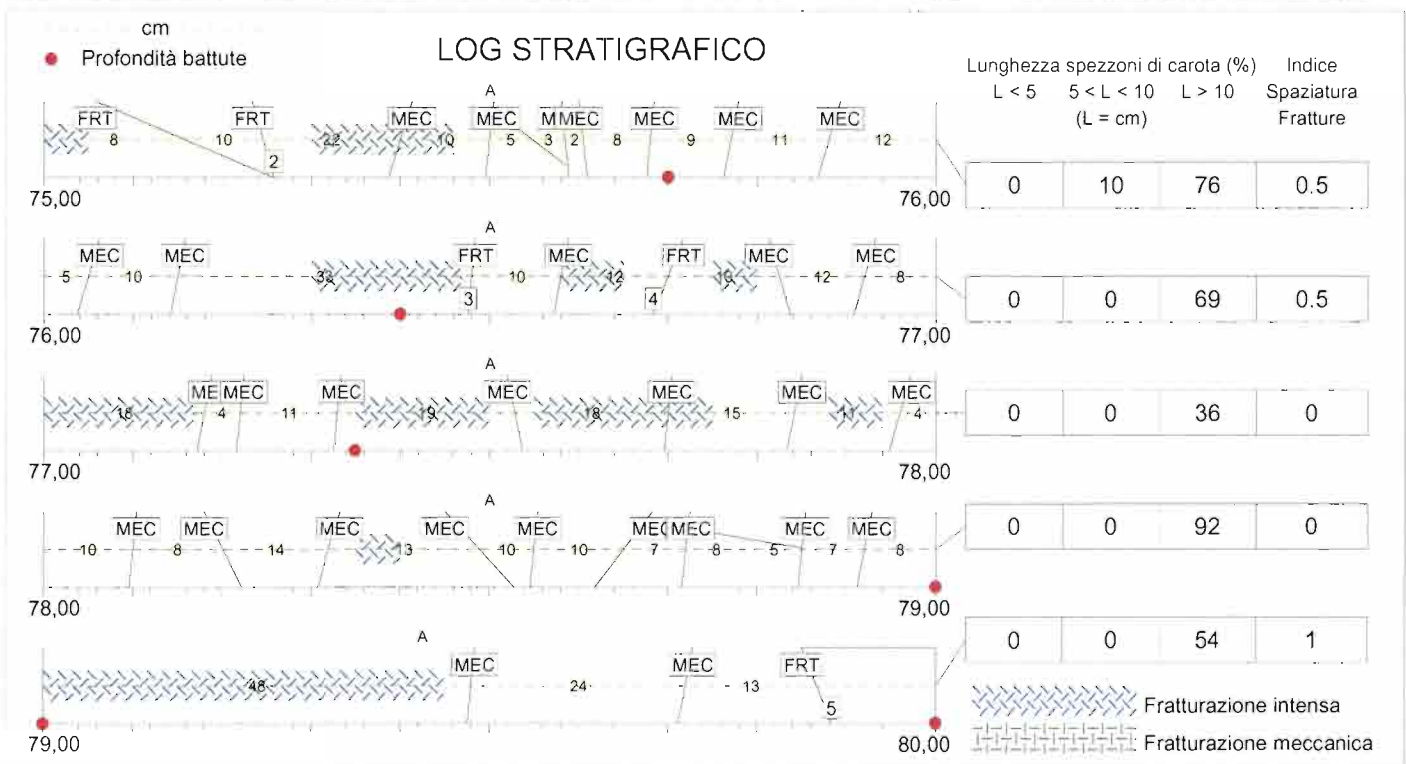
sondaggio CBV13 - cassetta n°16
