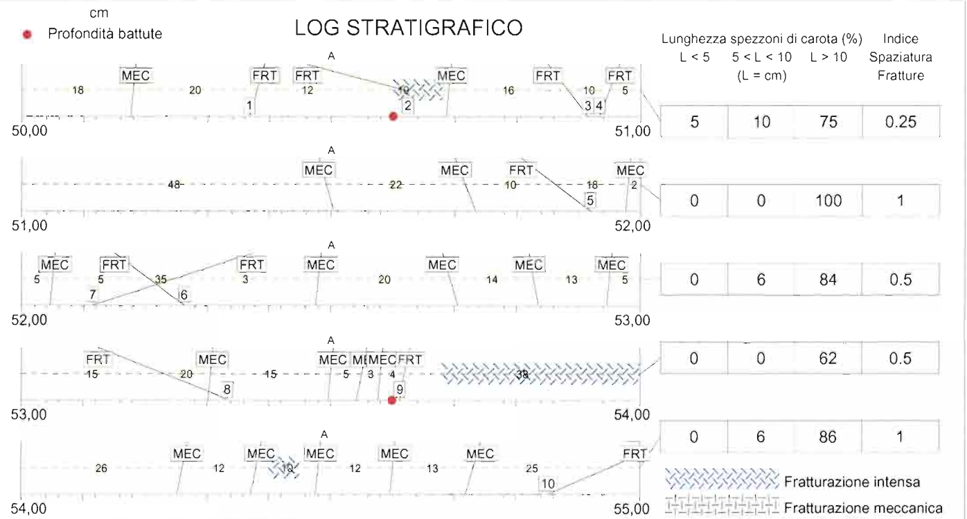
sondaggio CBV13 - cassetta n°11
