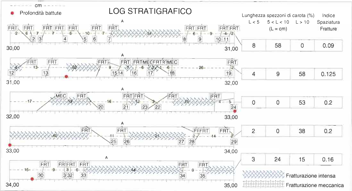
sondaggio C 27 - cassetta 7
