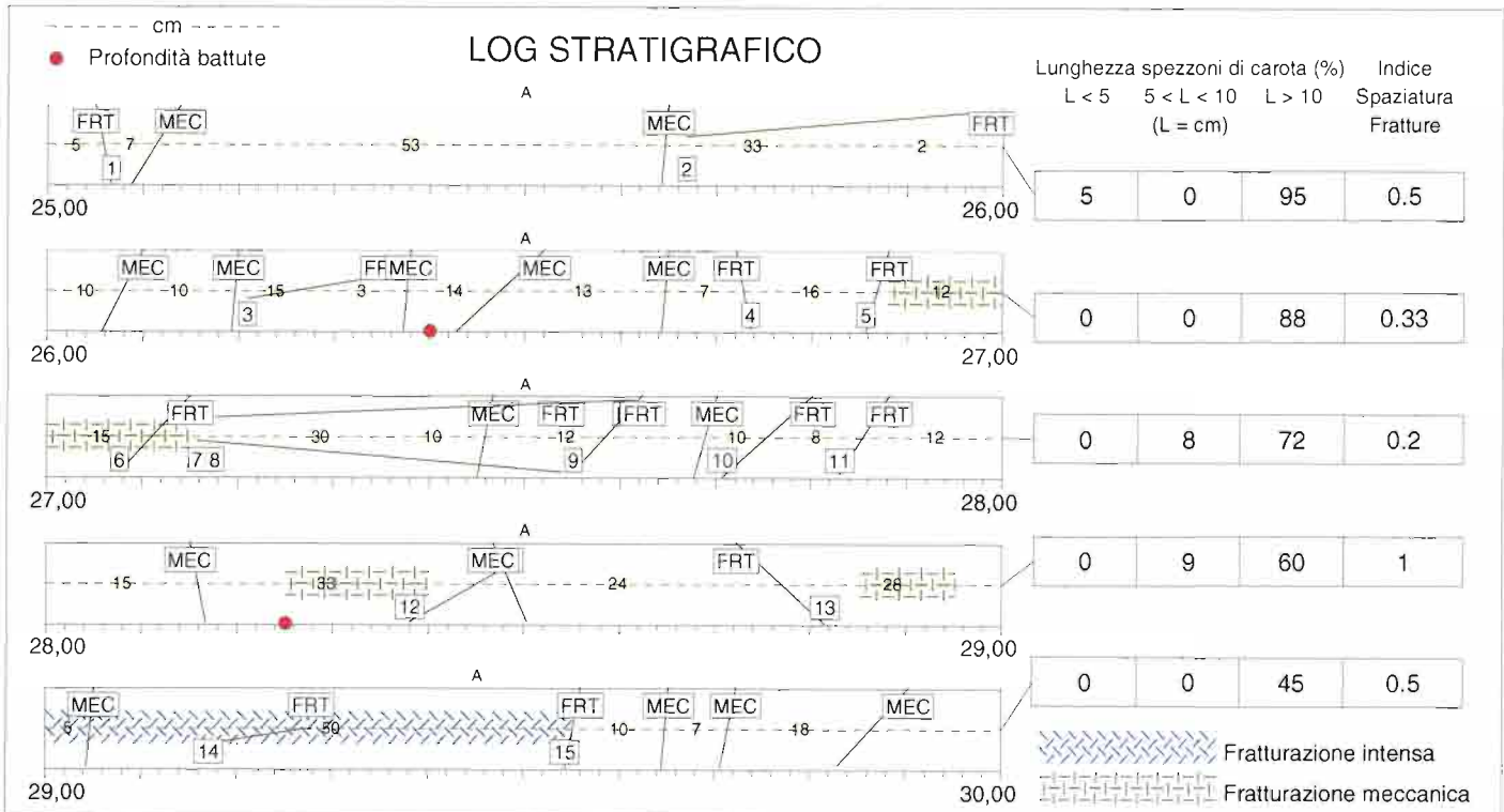
sondaggio CBV13 - cassetta n°6
