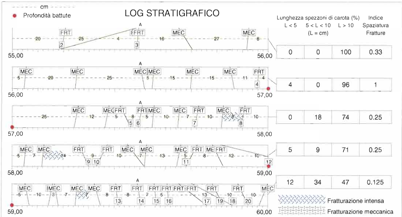
sondaggio CBV13 - cassetta n°12
