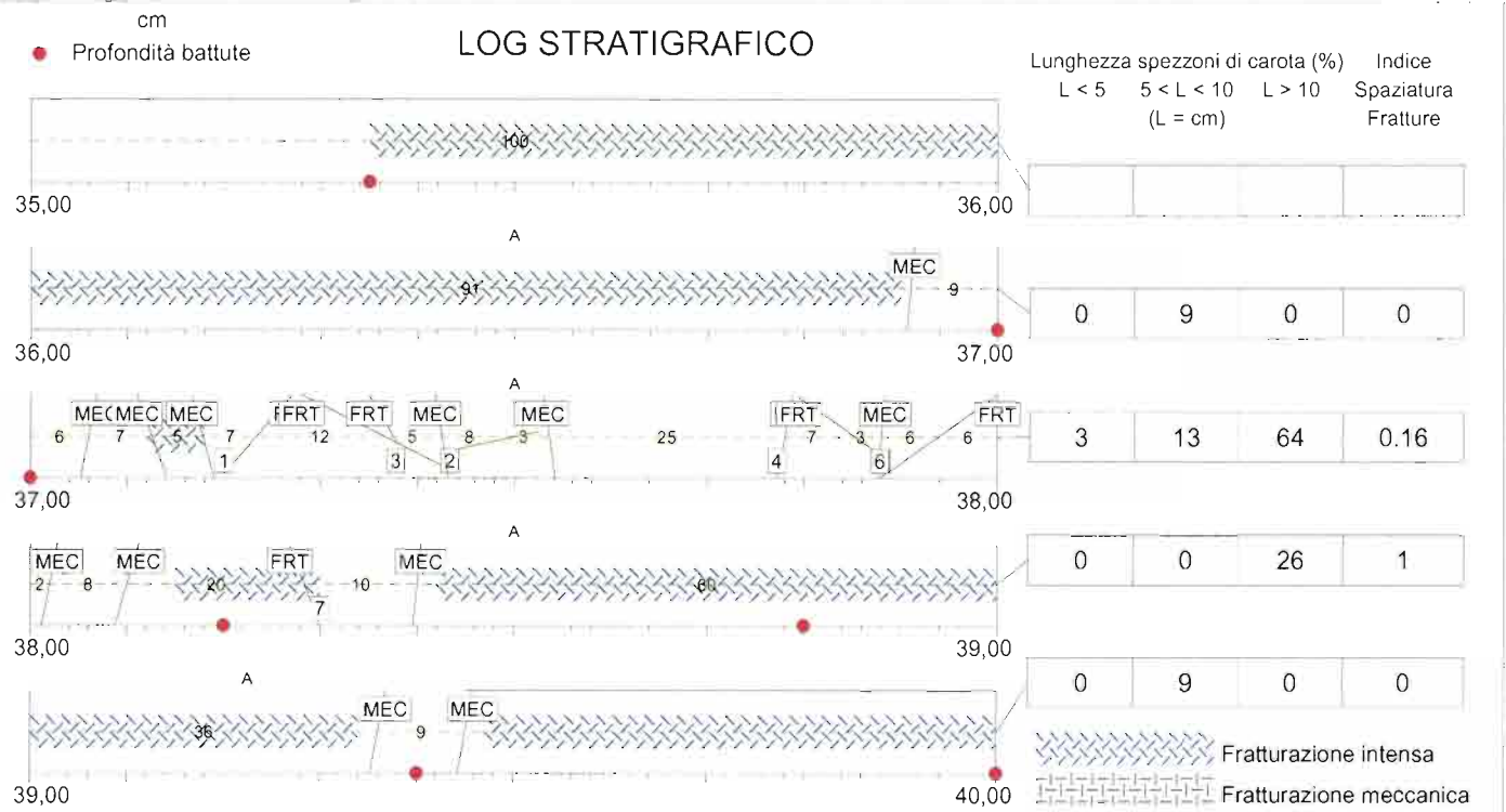
sondaggio C26 - cassetta 8
