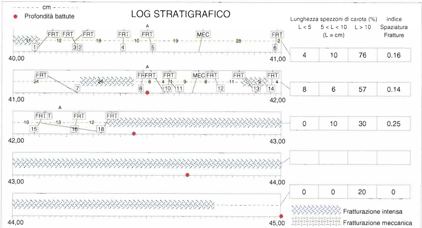
sondaggio C 27 - cassetta 9
