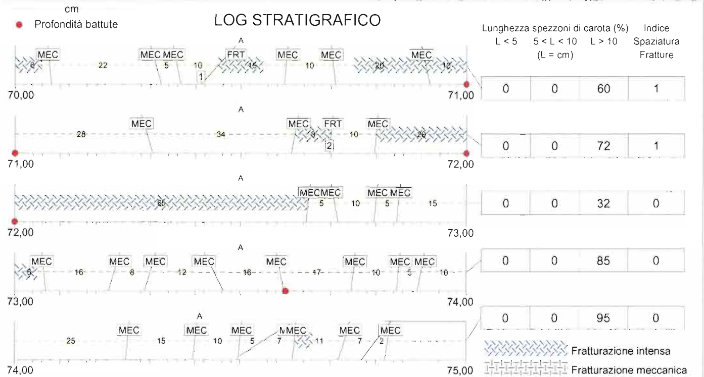
sondaggio CBV13 - cassetta n°15
