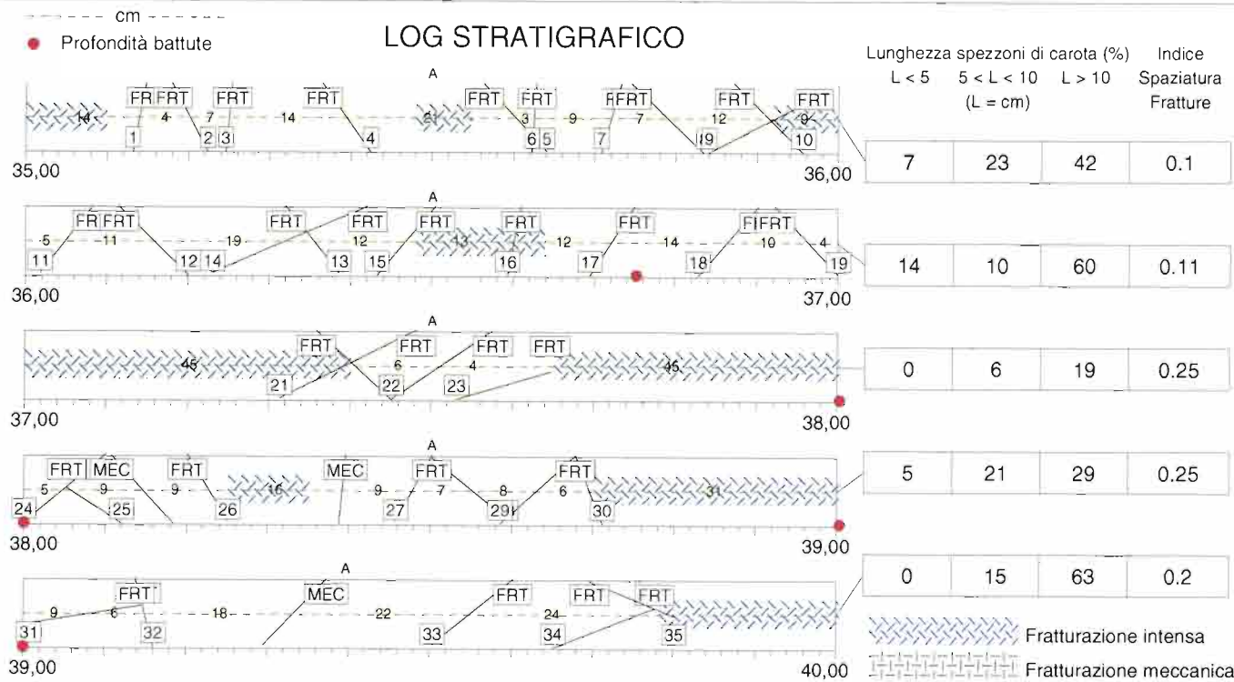
sondaggio C 27 - cassetta 8
