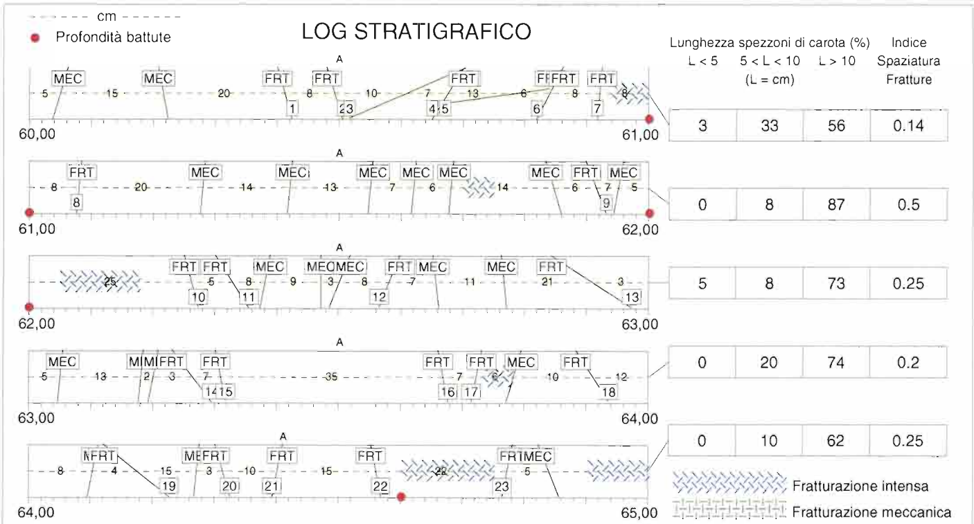
sondaggio CBV13 - cassetta n°13
