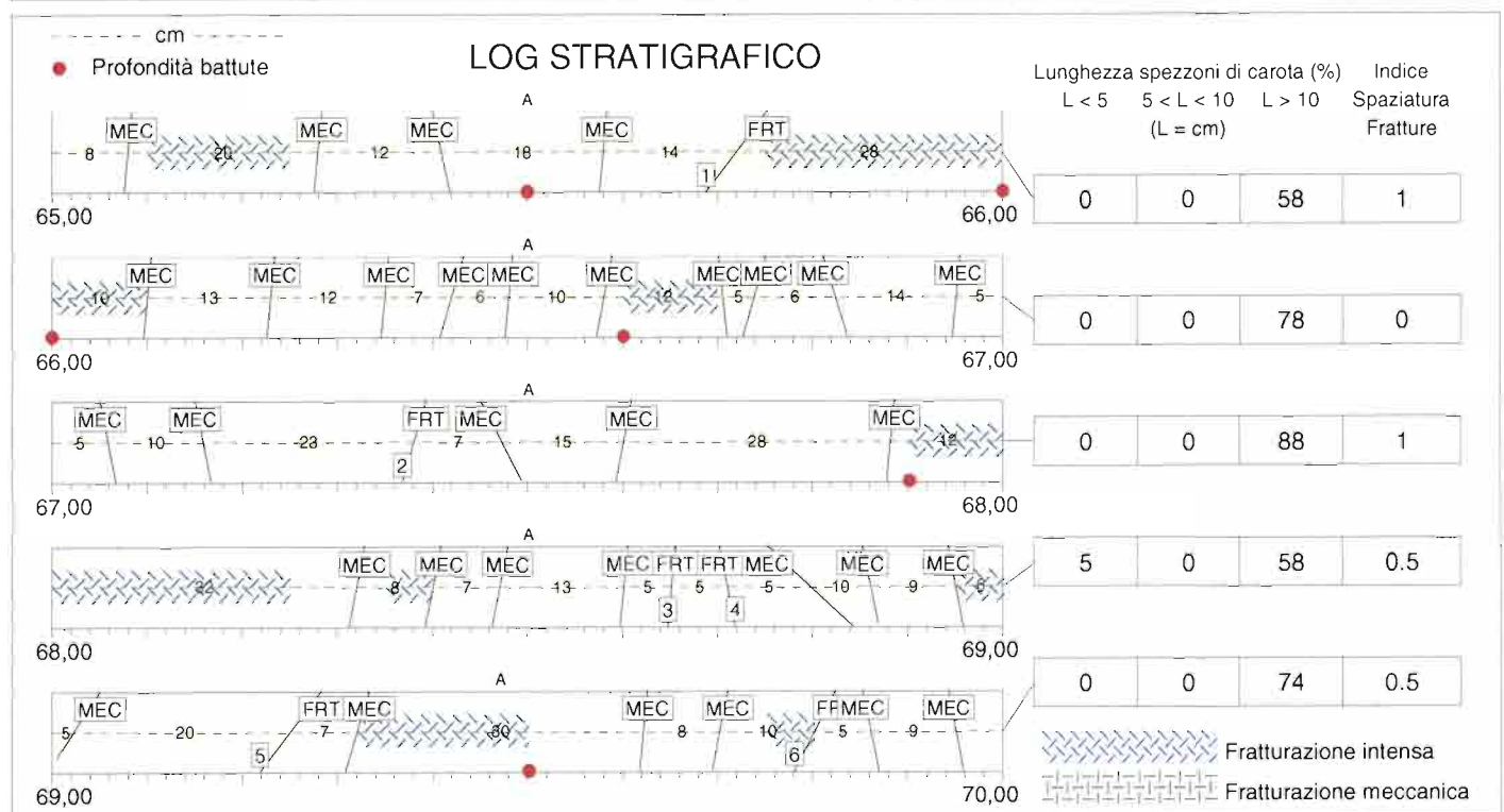
sondaggio CBV13 - cassetta n°14
