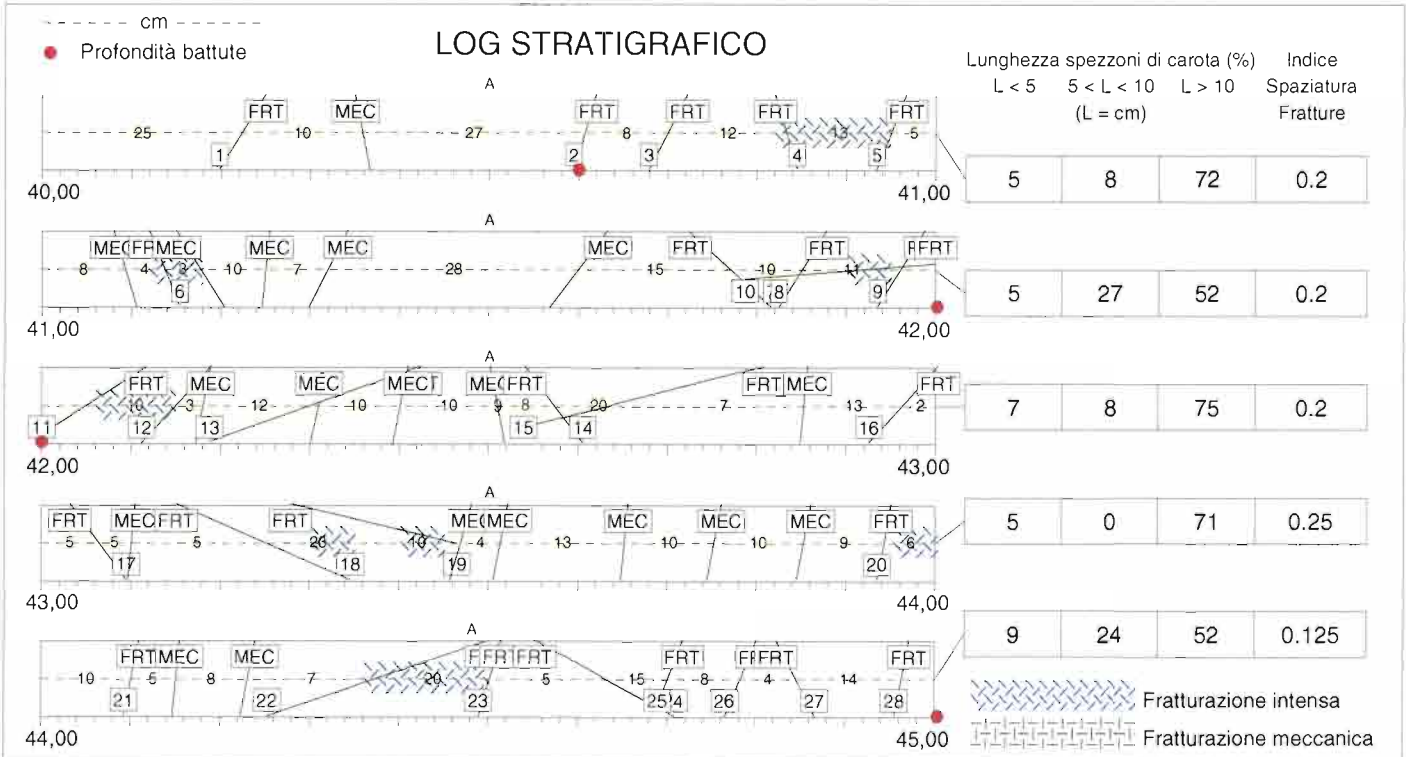
sondaggio CBV13 - cassetta n° 9
