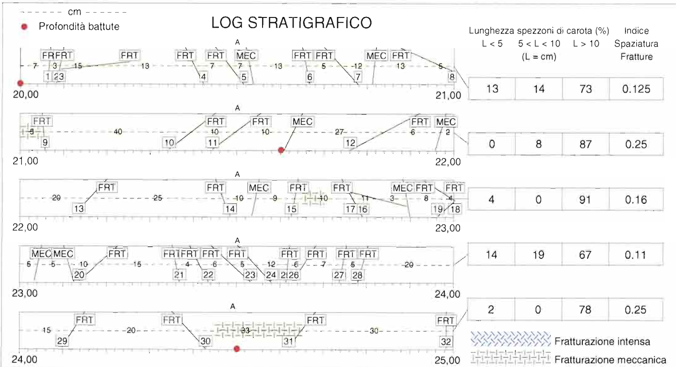
sondaggio CBV13 - cassetta n°5
