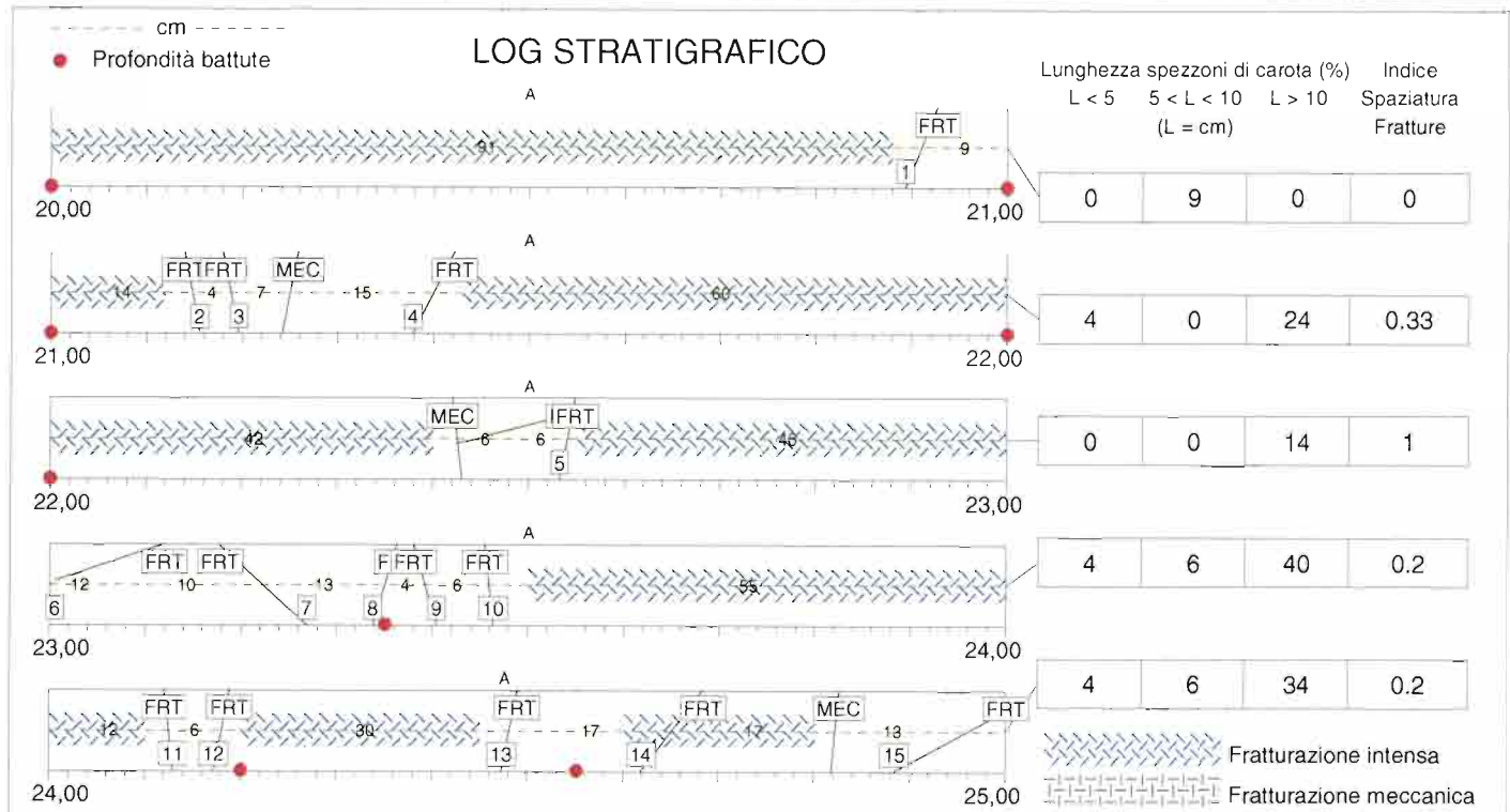
sondaggio C 27 - cassetta 5
