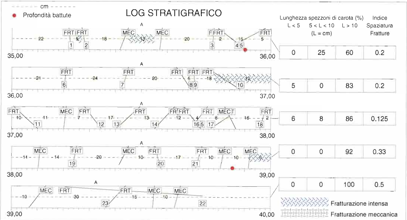
sondaggio CBV13 - cassetta n°8
