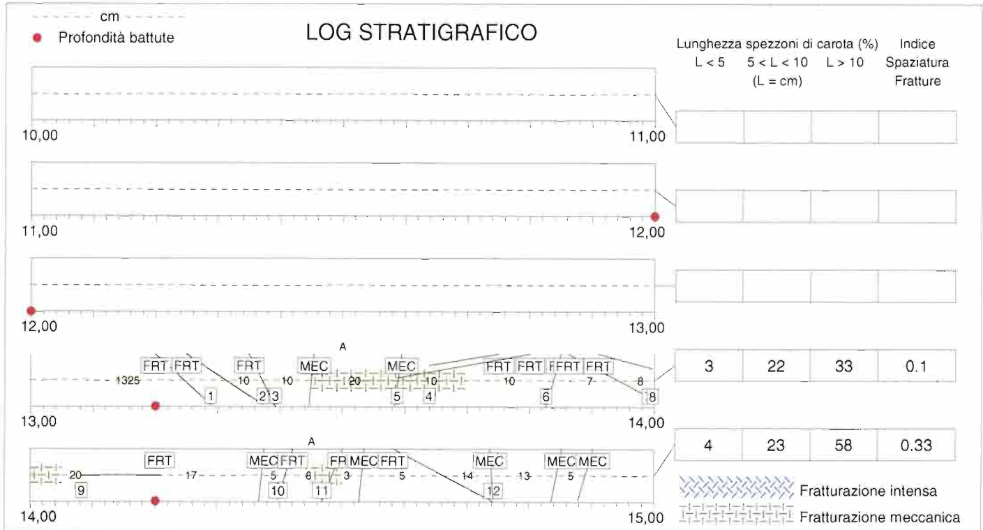
sondaggio CBV13 - cassetta n°3
