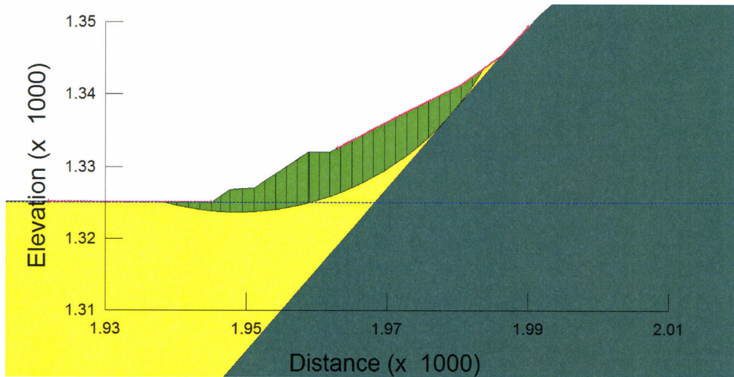
Figura 9: Deposito B (Fase di scavo)– analisi di stabilità globale in campo sismico – k_v > 0
