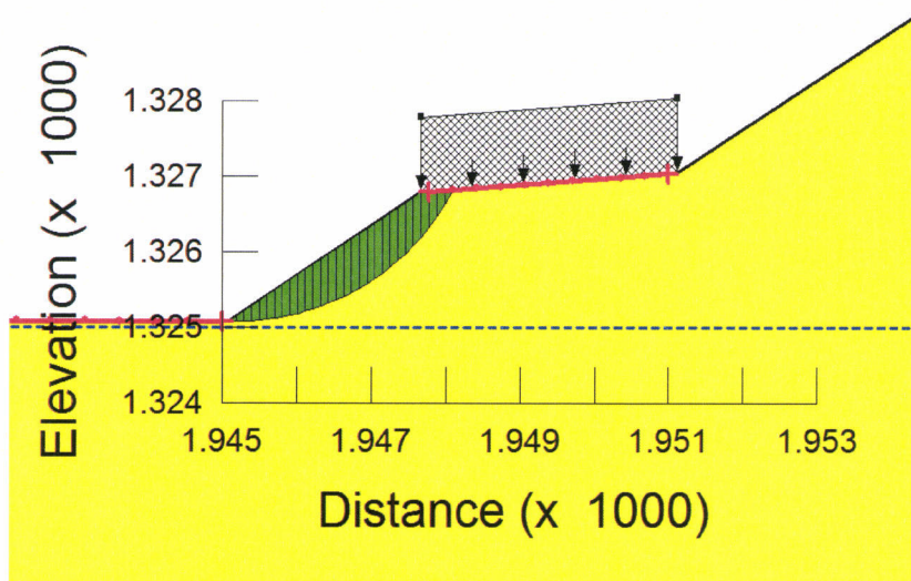
Figura 8: Deposito B (Fase di scavo) – analisi di stabilità locale in campo sismico – k_v < 0
