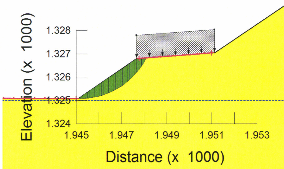
Figura 6: Deposito B (Fase di scavo) – analisi di stabilità locale in campo statico
