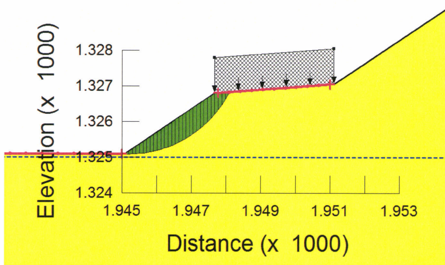
Figura 10: Deposito B (Fase di scavo)– analisi di stabilità locale in campo sismico – k_v > 0
