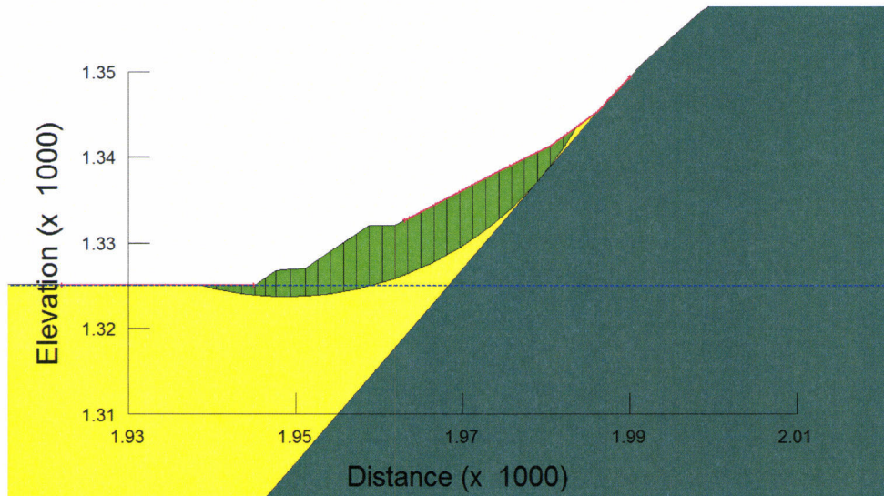
Figura 5: Deposito B (Fase di scavo) – analisi di stabilità globale in campo statico
