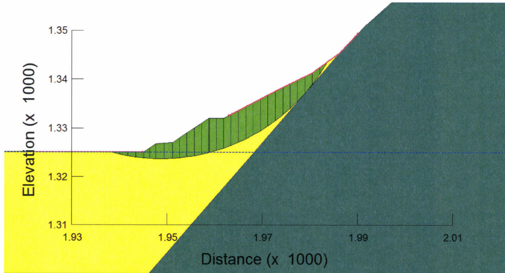
Figura 7: Deposito B (Fase di scavo) – analisi di stabilità globale in campo sismico – k_v < 0
