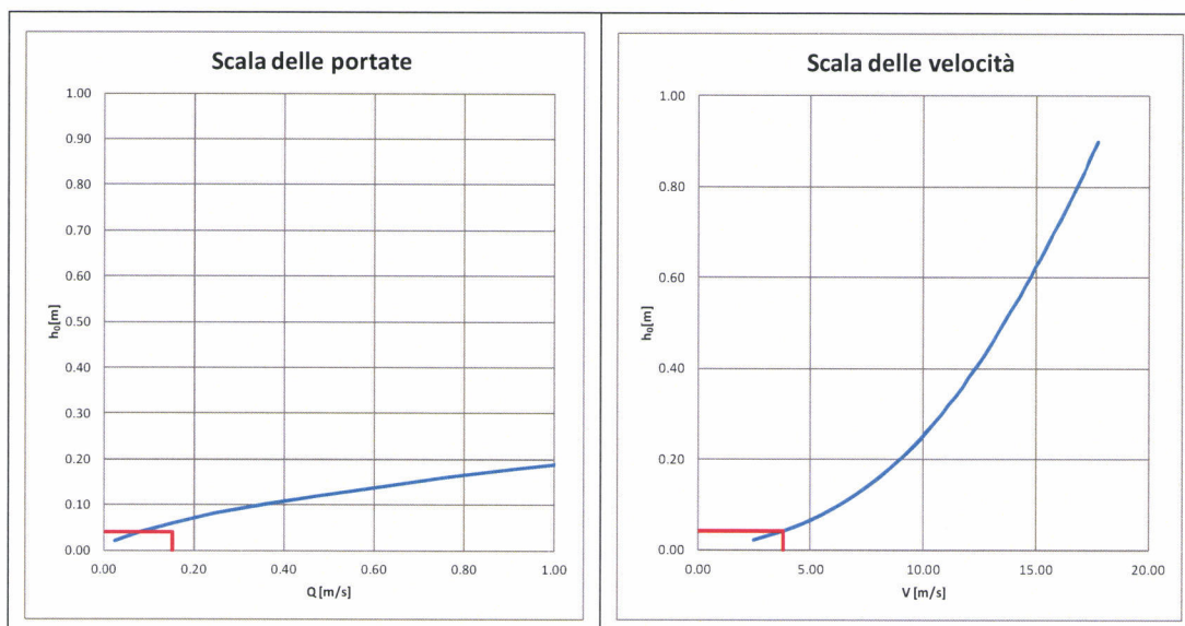
Figura 9: Canaletta in pietrame – Pendenza 50% - Scala delle portate e scala delle velocità
