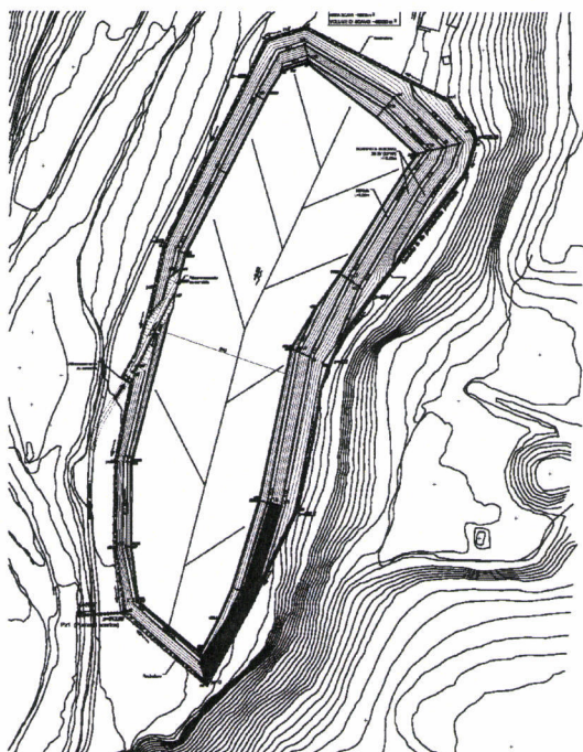
Figura 1: Individuazione sottobacini – configurazione di scavo
