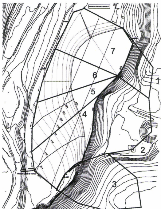
Figura 2: Individuazione sottobacini – configurazione finale di progetto
