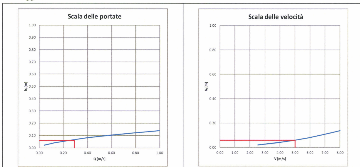
Figura 7: Canaletta in pietrame – Pendenza >50% - Scala delle portate e scala delle velocità
