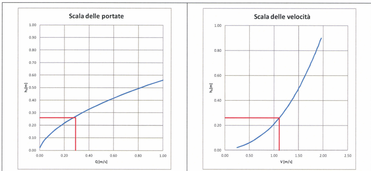
Figura 6: Canaletta in pietrame – Pendenza 0.5% - Scala delle portate e scala delle velocità
