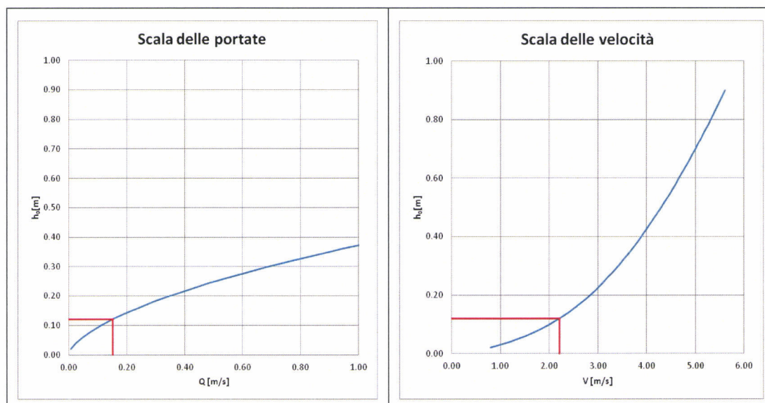
Figura 8: Canaletta in pietrame – Pendenza 0.5% - Scala delle portate e scala delle velocità
