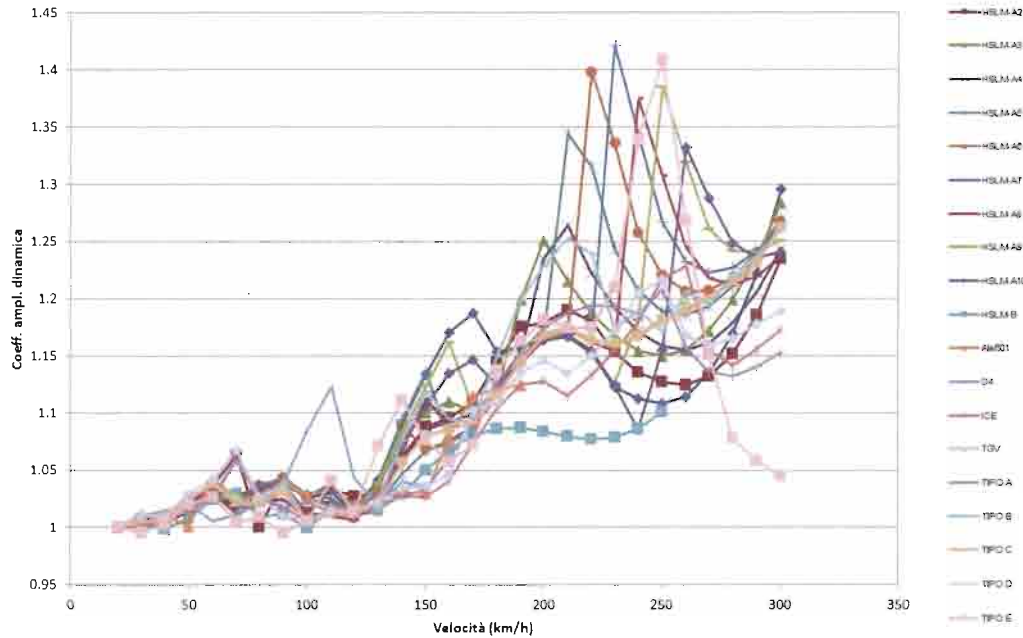
Coefficiente di amplificazione dinamica - ISARCO_23.04
