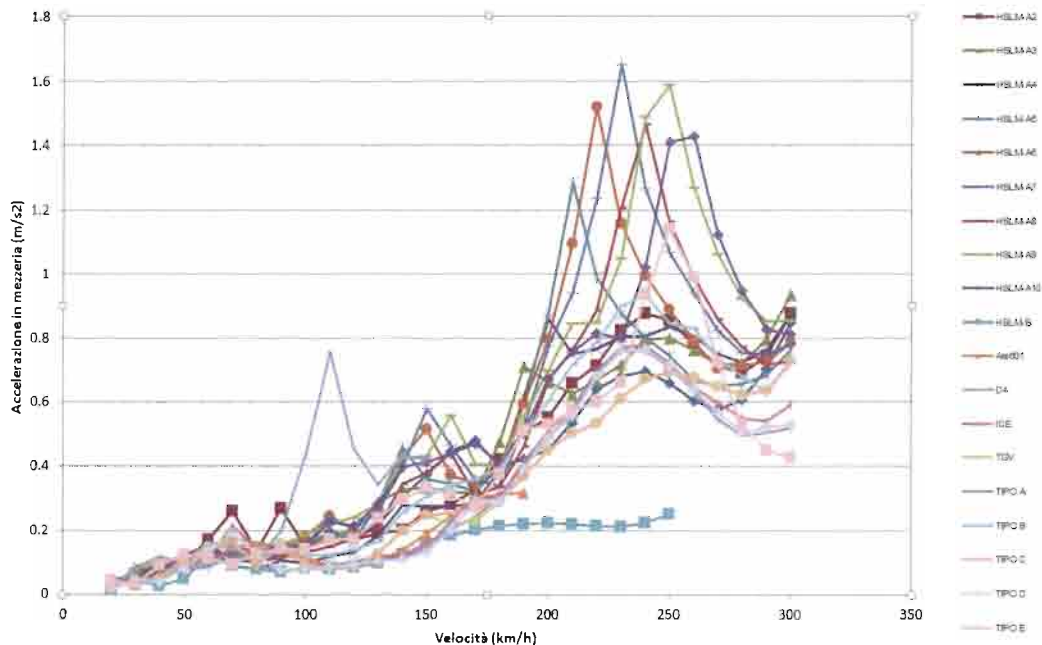
Accelerazione in mezzeria - ISARCO_23.04
