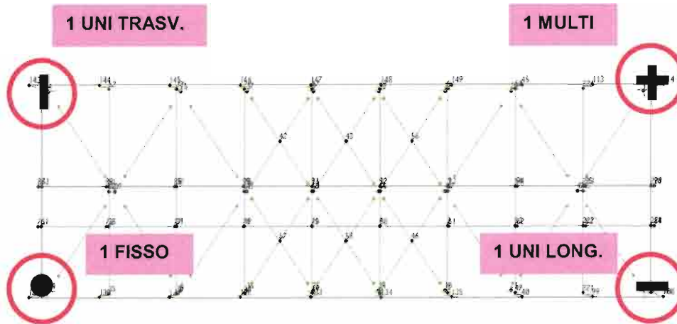
Figura 3 - Sistema di vincolo impalcato
