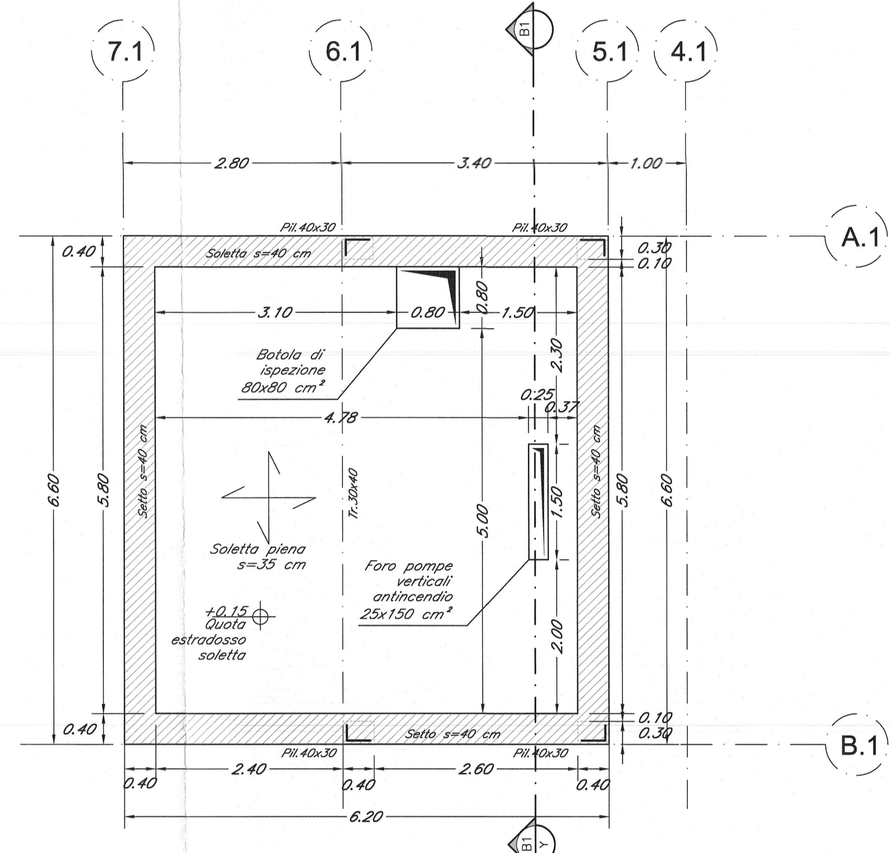
CARPENTERIA FONDAZIONI scala 1:50
