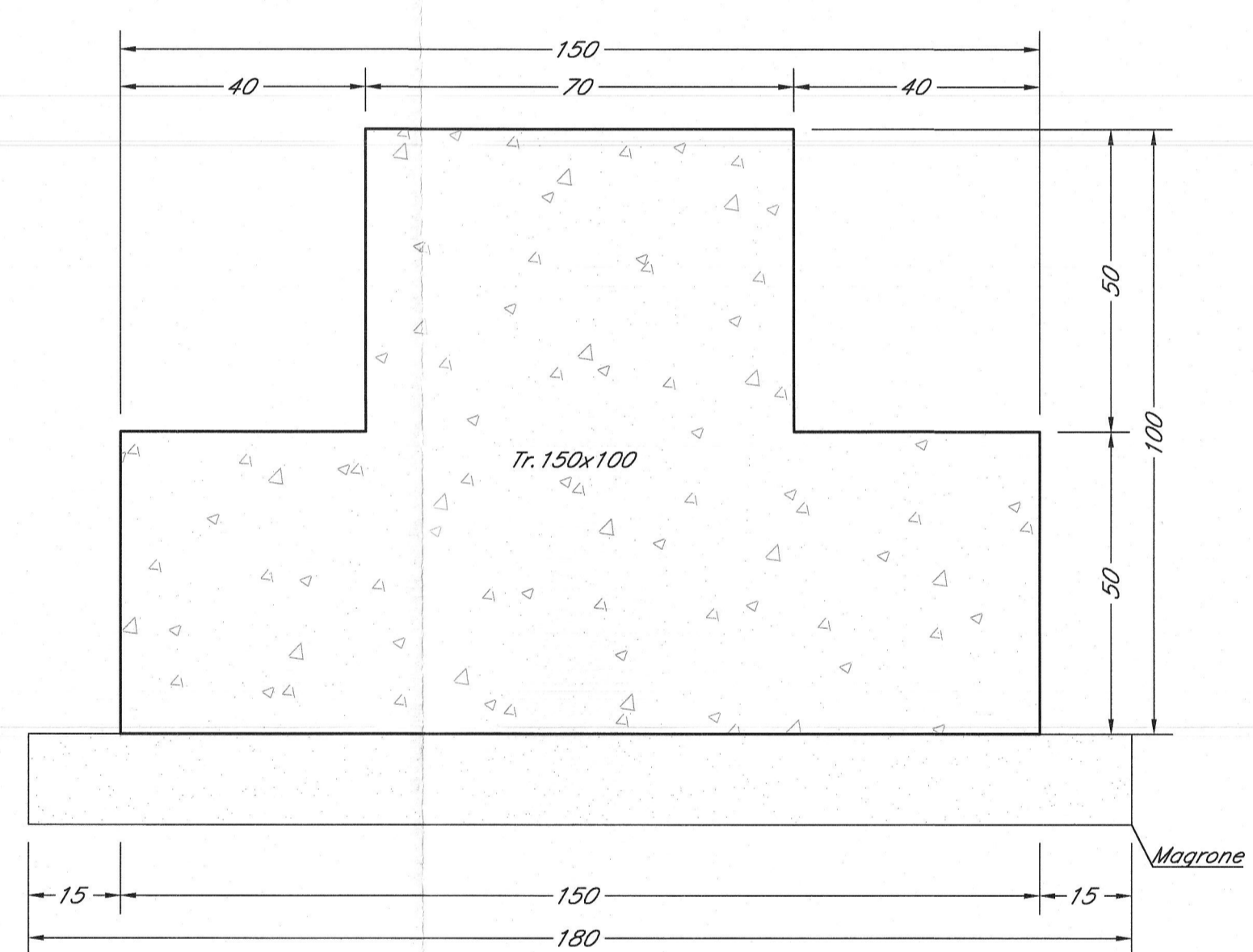
SEZIONE 1-1 scala 1:10
