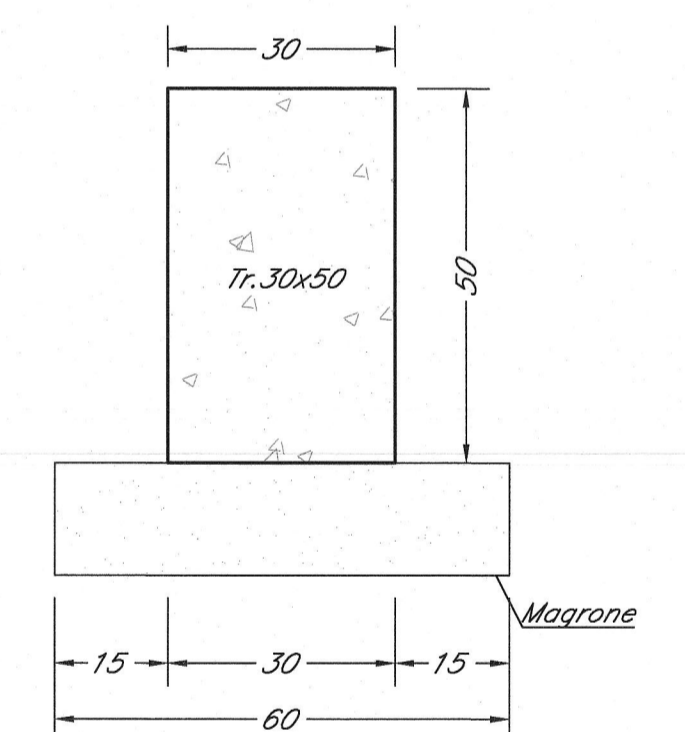
SEZIONE 2-2 scala 1:10
