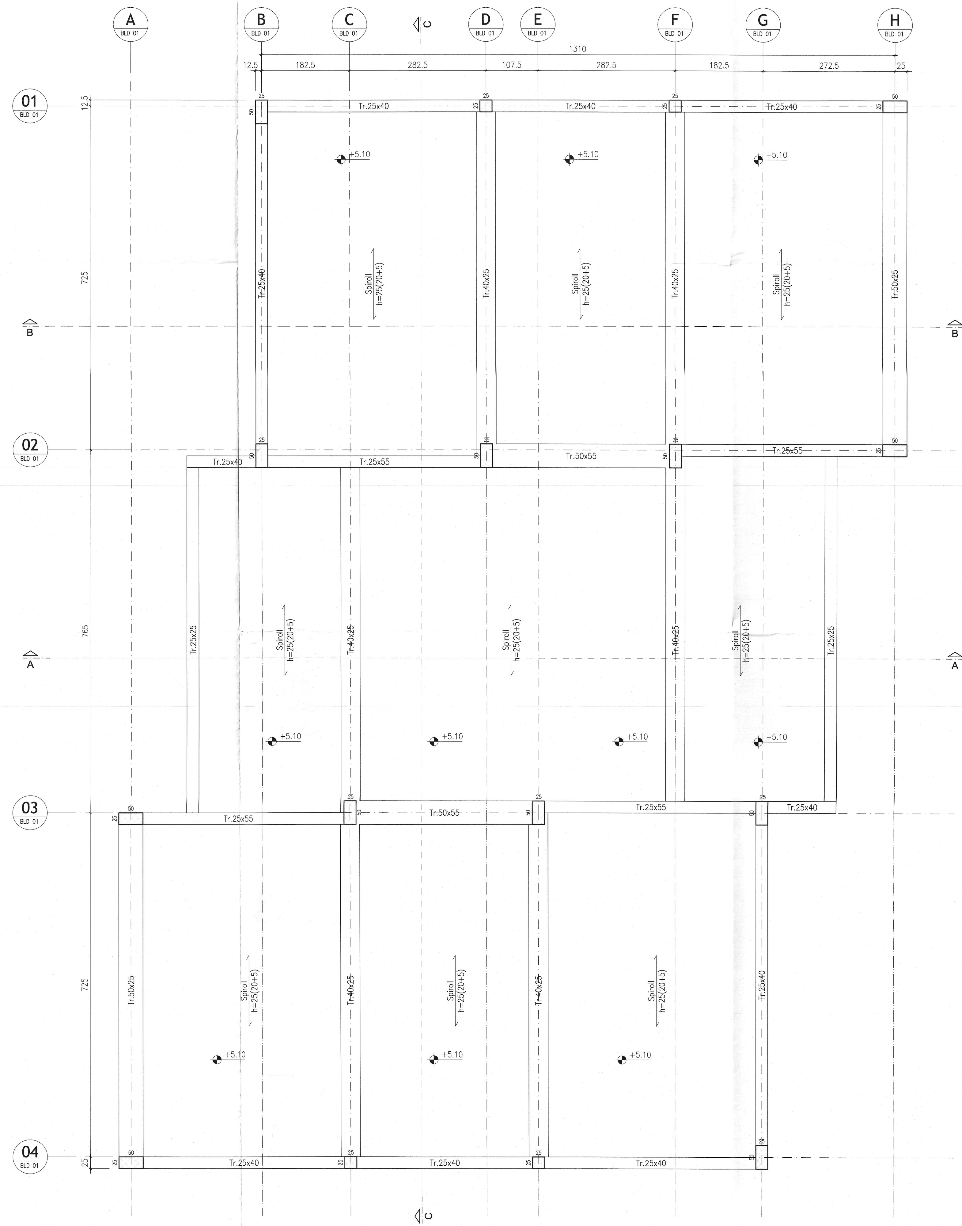
Carpenteria copertura Scala 1:50
