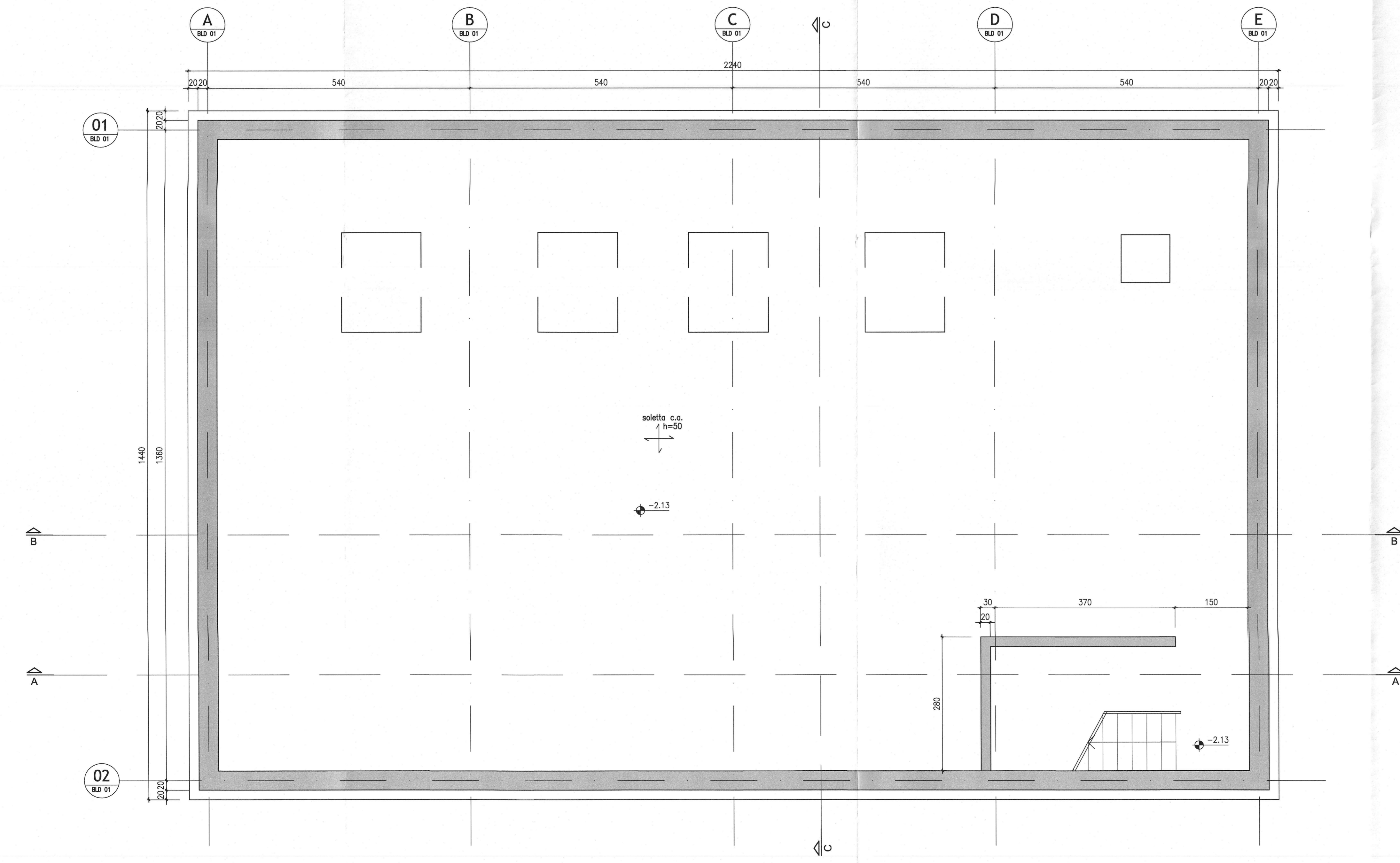
Pianta fondazioni Q.ta -1.97 Scala 1:50
