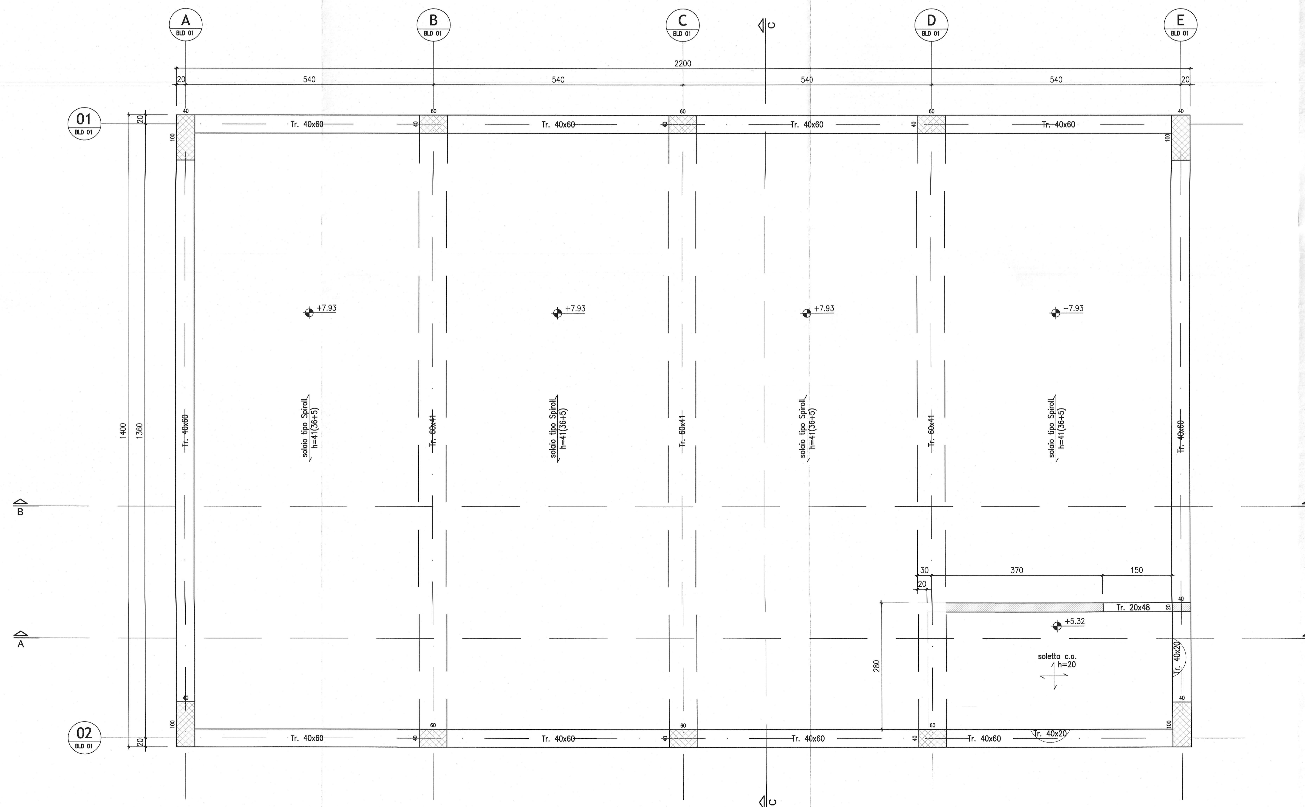
Carpenteria piano copertura Q.ta +7.93 Scala 1:50
