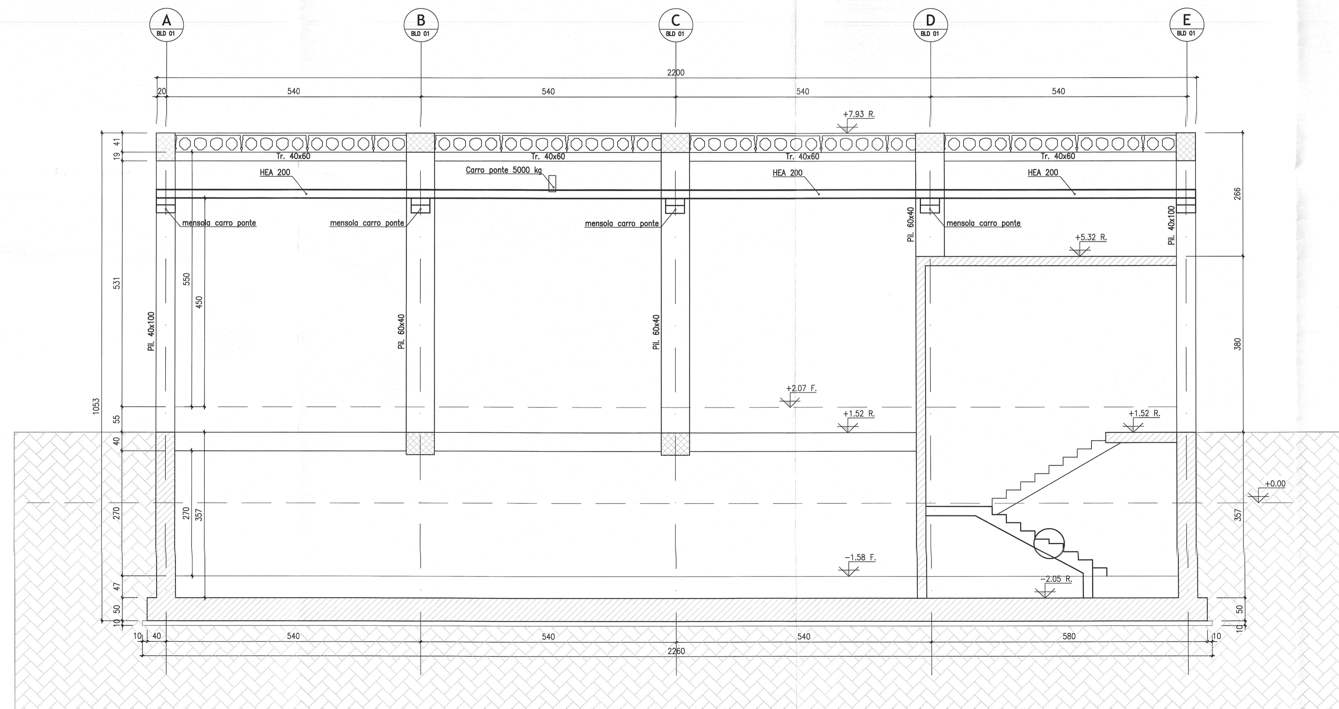
SEZIONE B-B
