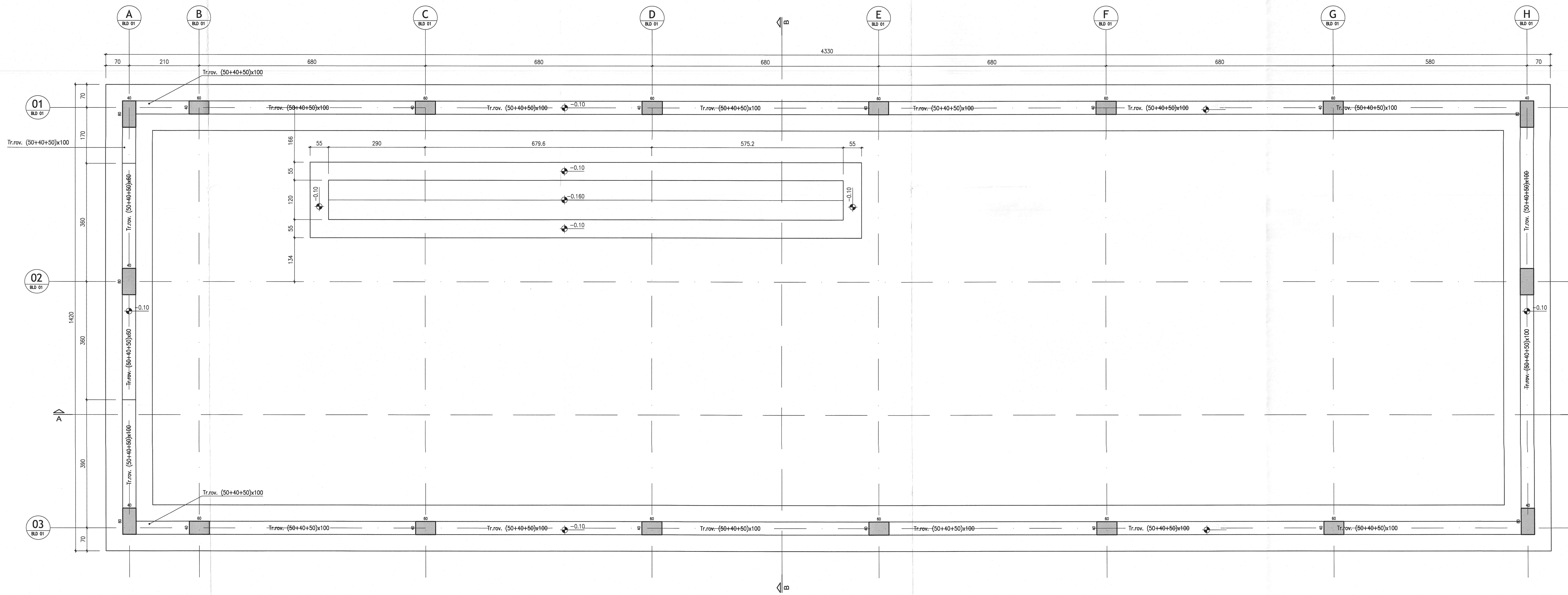
Pianta fondazioni Q.ta -0.10 Scala 1:50
