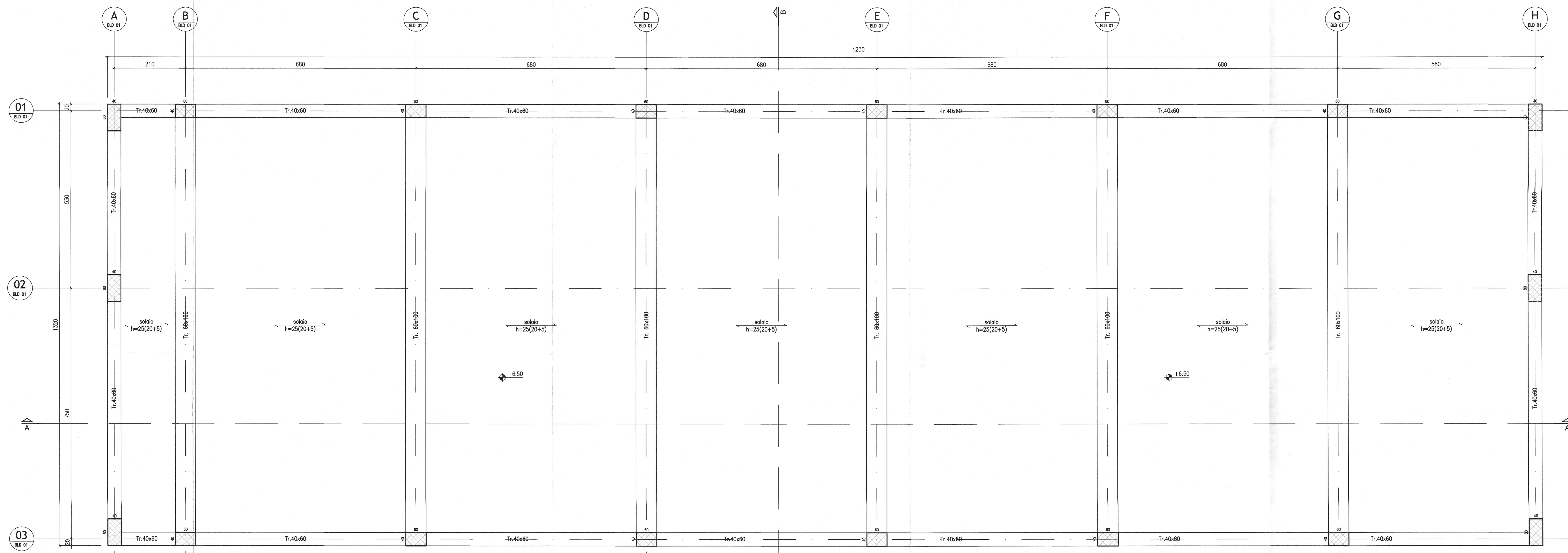
Carpenteria copertura Q.ta -0.10 Scala 1:50
