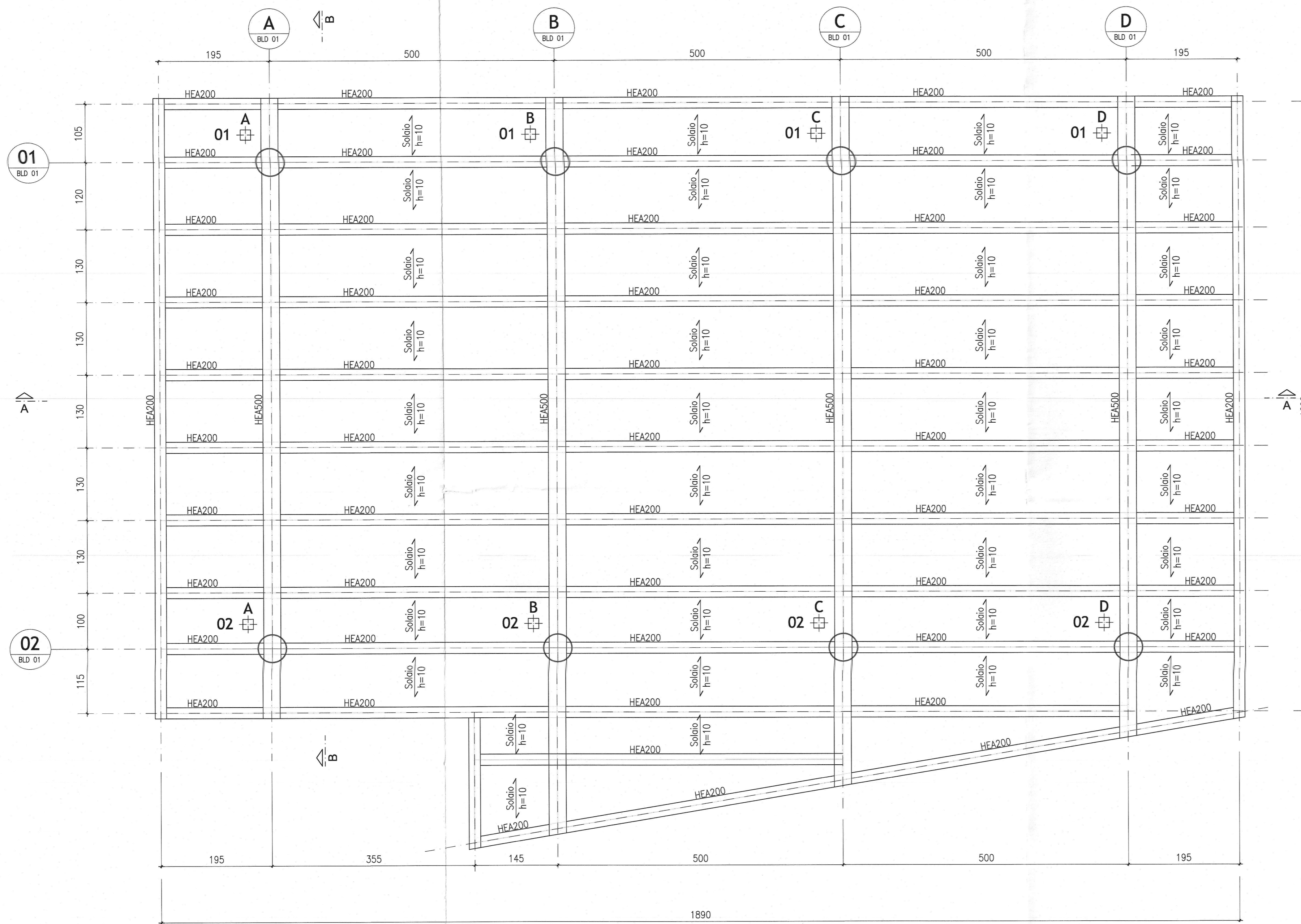
CARPENTERIA PIANO PRIMO Q.ta +6.20 Scala 1:50
