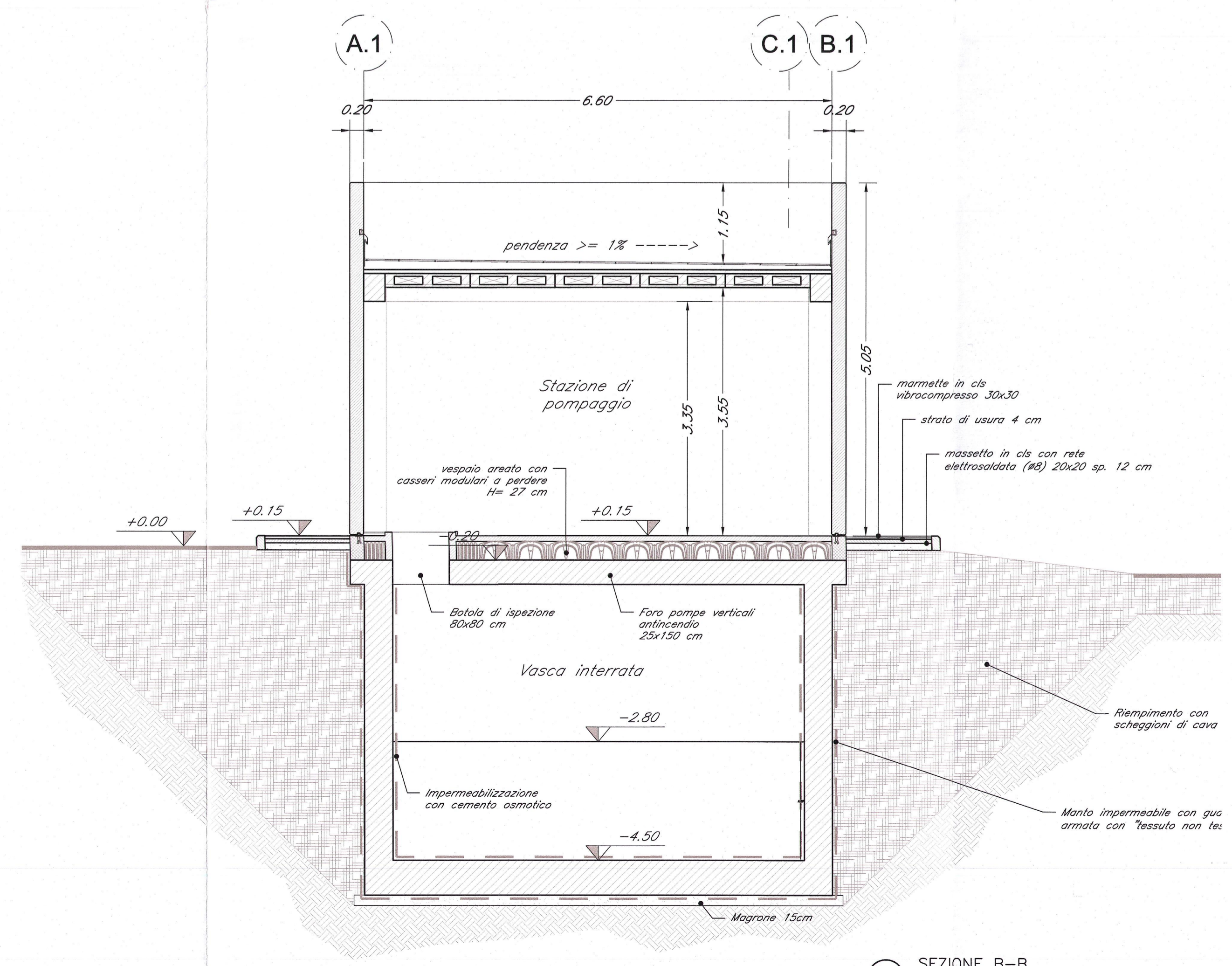
SEZIONE B-B scala 1:50
