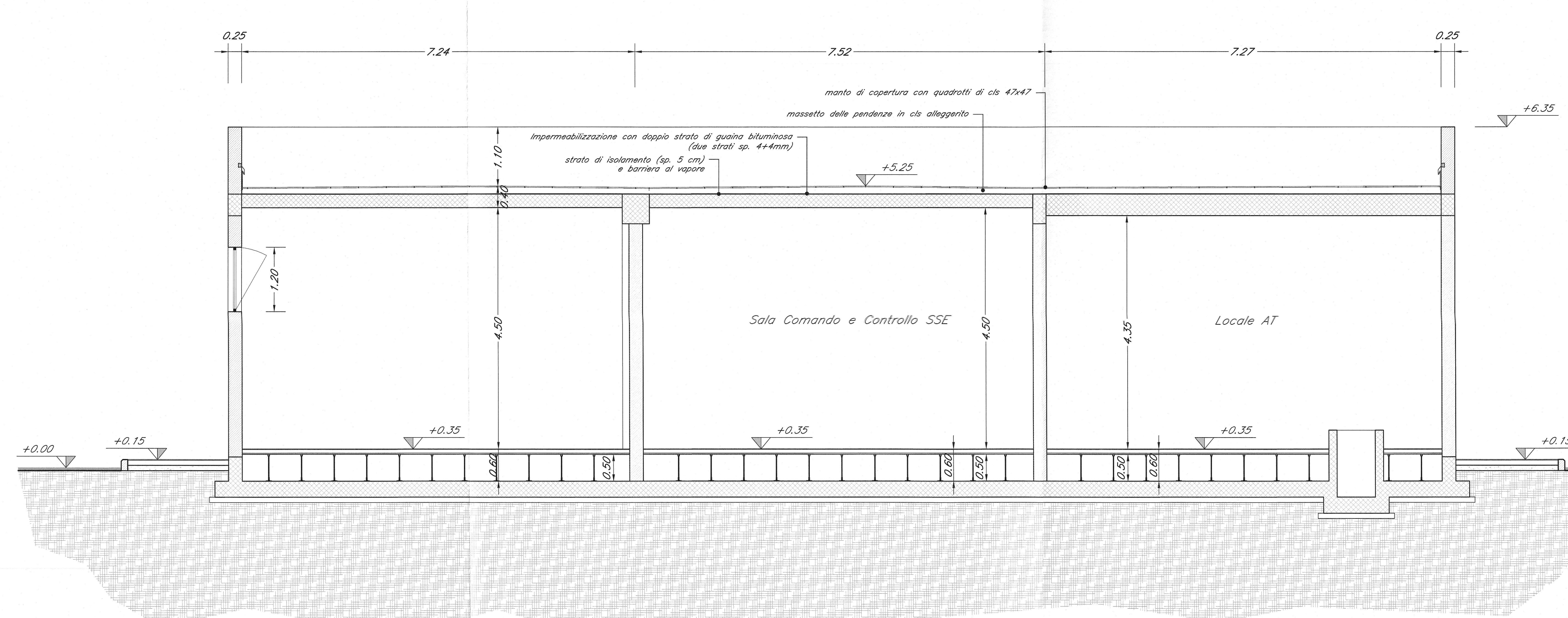
BB SEZIONE BB scala 1:50
