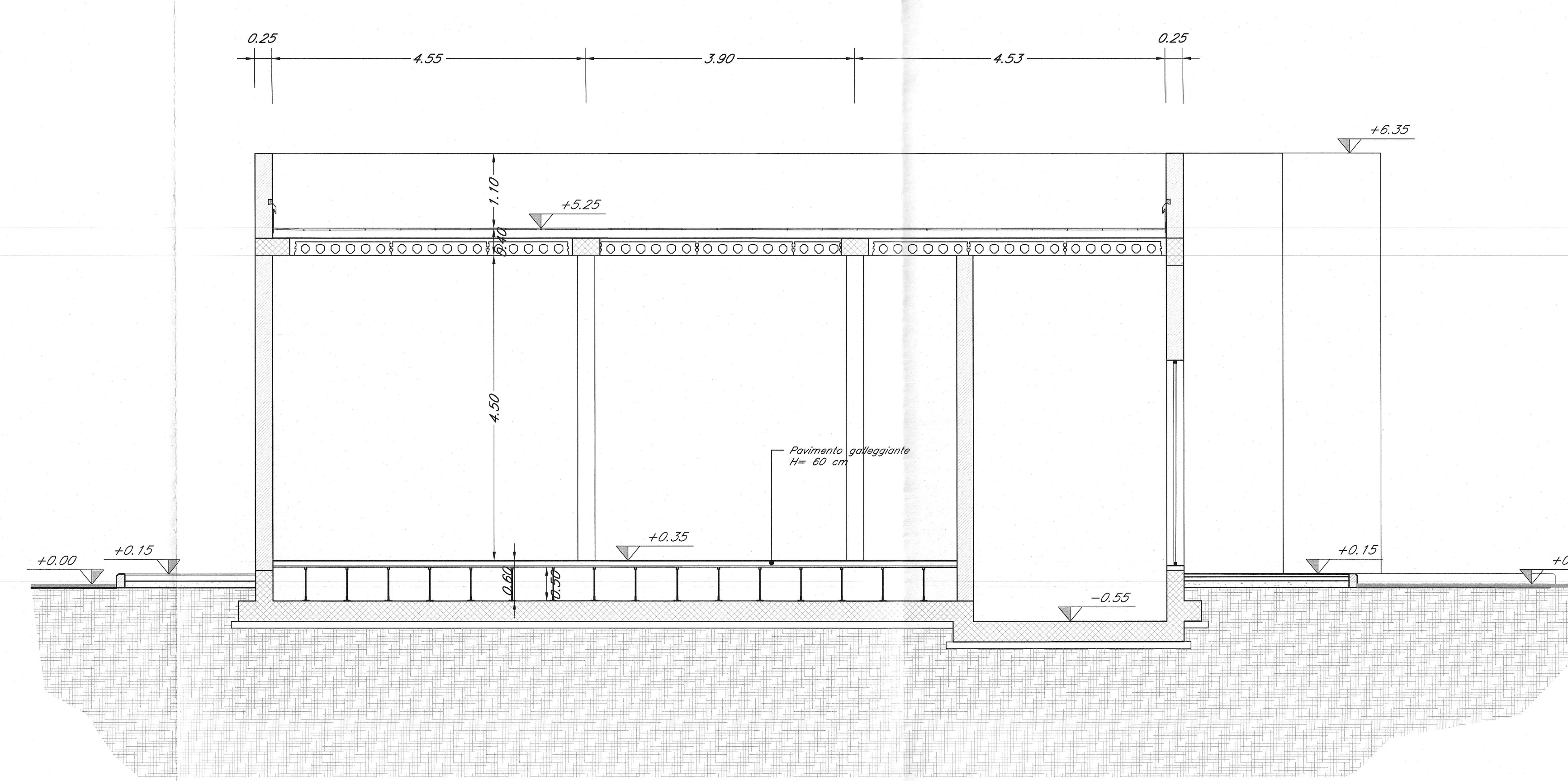
CC SEZIONE CC scala 1:50
