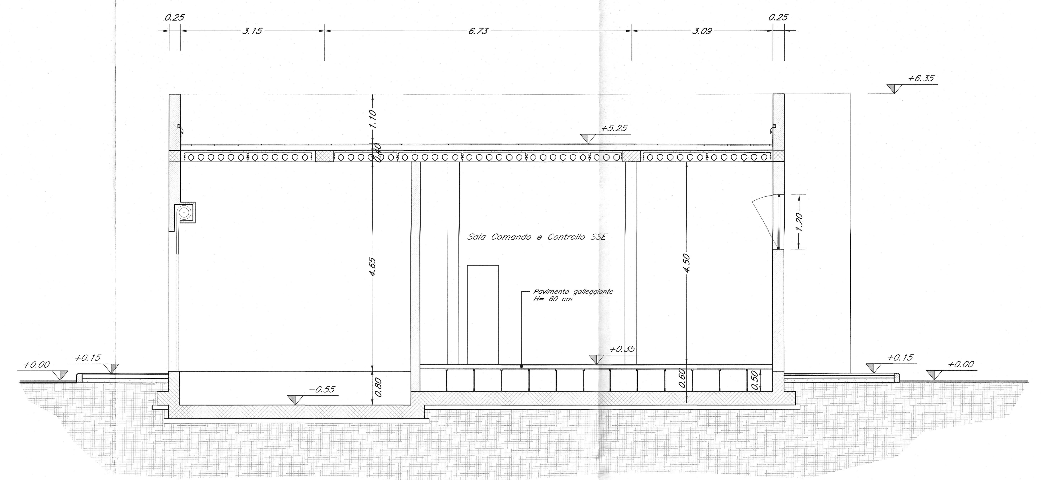
AA SEZIONE AA scala 1:50
