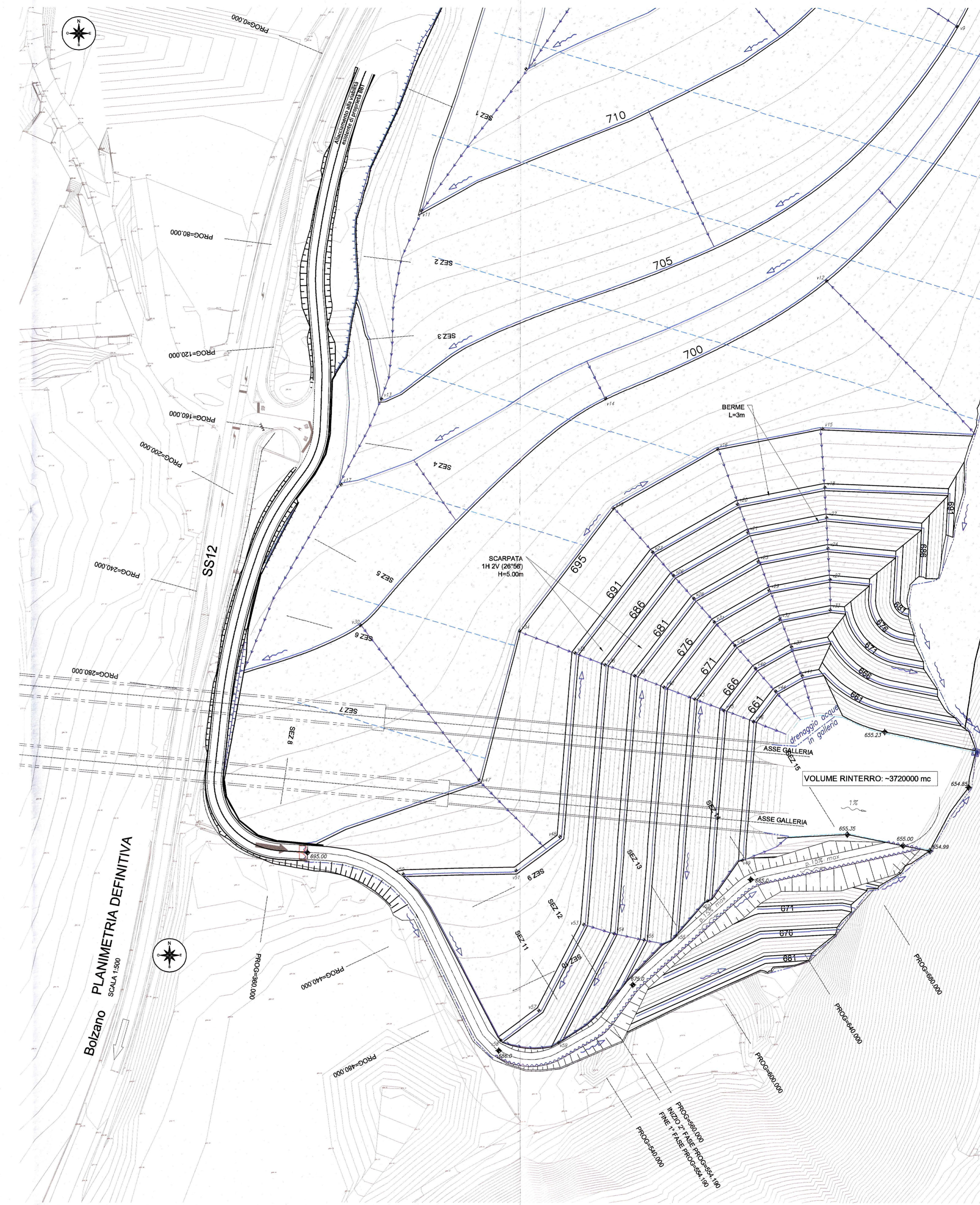
PLANIMETRIA SCALA 1:1000
