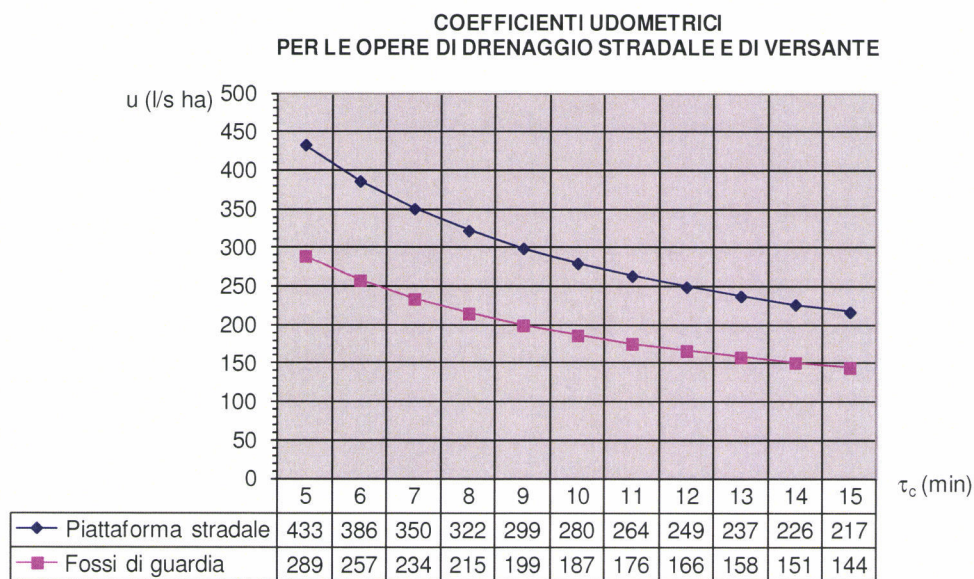
Fig. 2-2 – Coefficienti udometrici in funzione del tempo di corrivazione per il dimensionamento delle opere di drenaggio stradale e dei fossi di guardia – Stazione Chiuse
