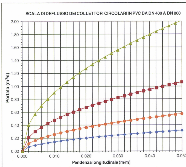
Fig. 2-8 - Scala di deflusso dei collettori circolari in PVC con diametro nominale variabile da DN400 a DN800 mm
