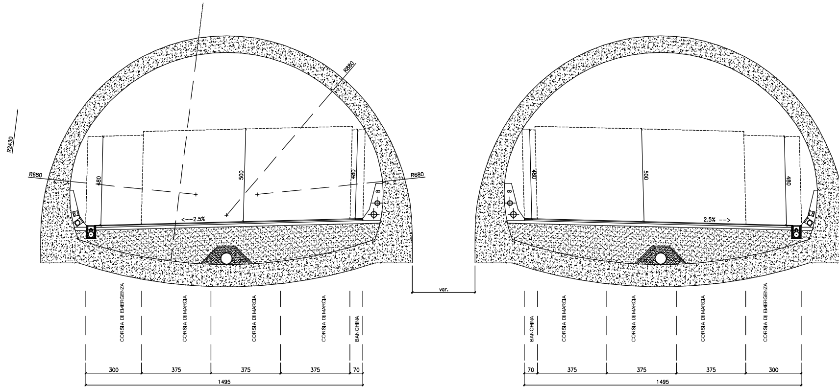
SEZIONE TIPO IN GALLERIA NATURALE TRATTO 1
