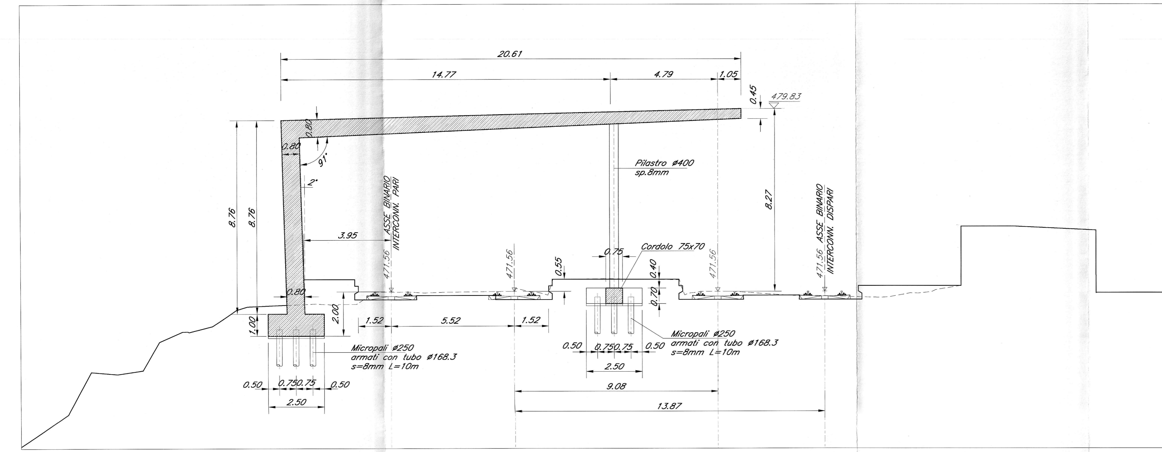
SEZIONE 85 - PK 2+987.65
