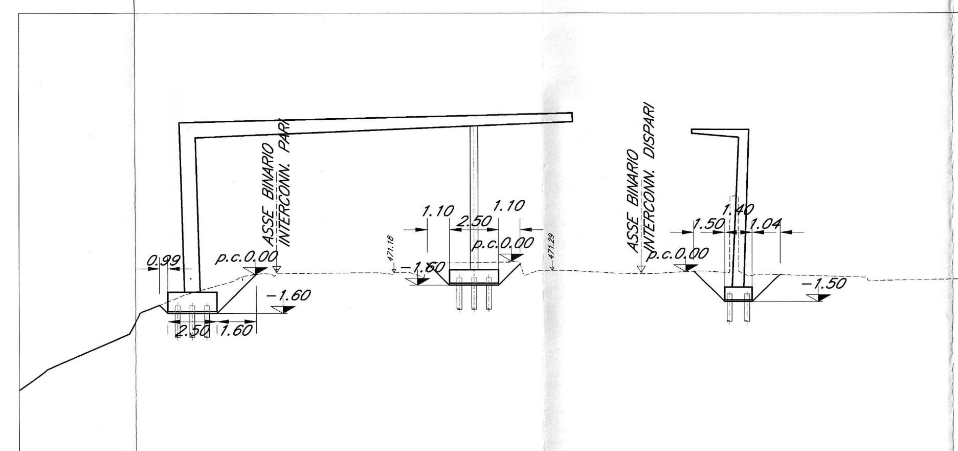
SEZIONE 61 Scala 1:200
