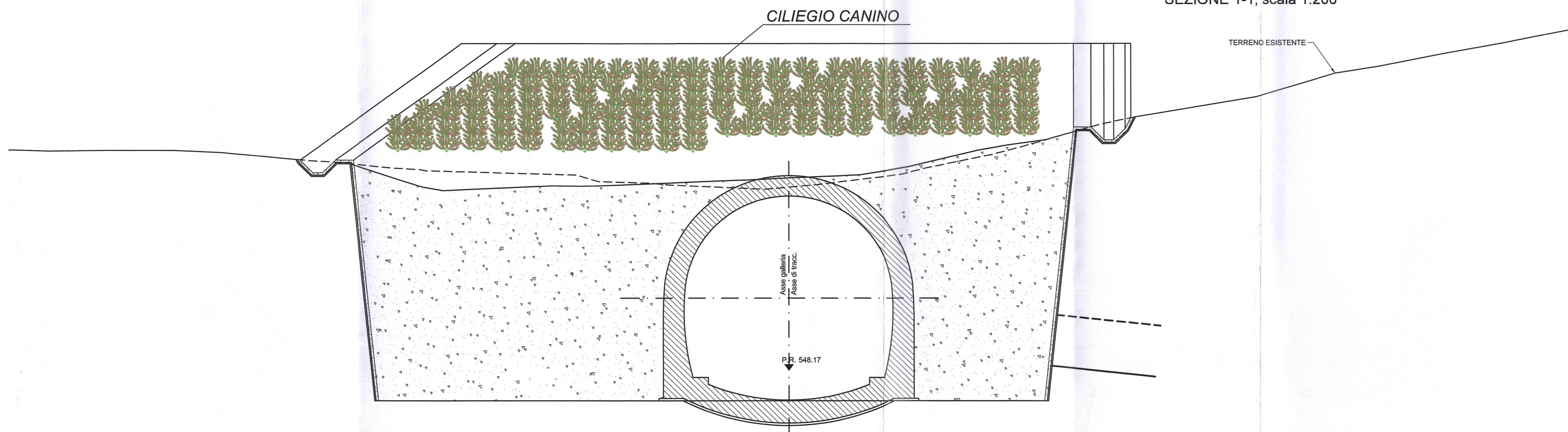
SEZIONE 1-1, scala 1:200
