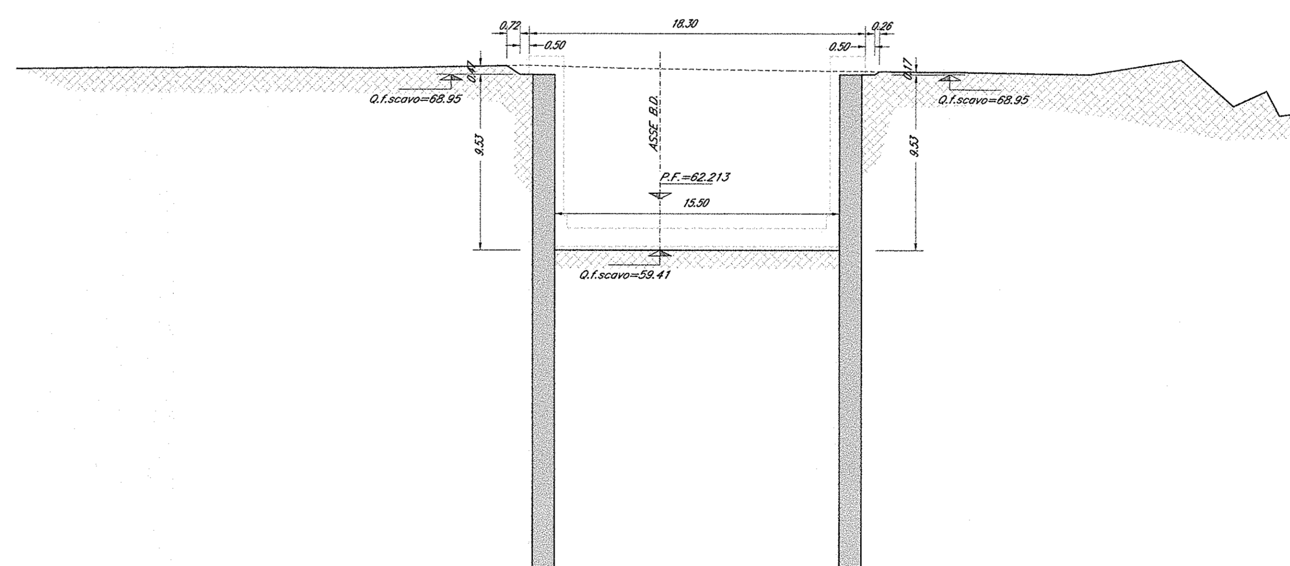
SEZIONE 9: Prog. 2+730.00 Scala 1:200
