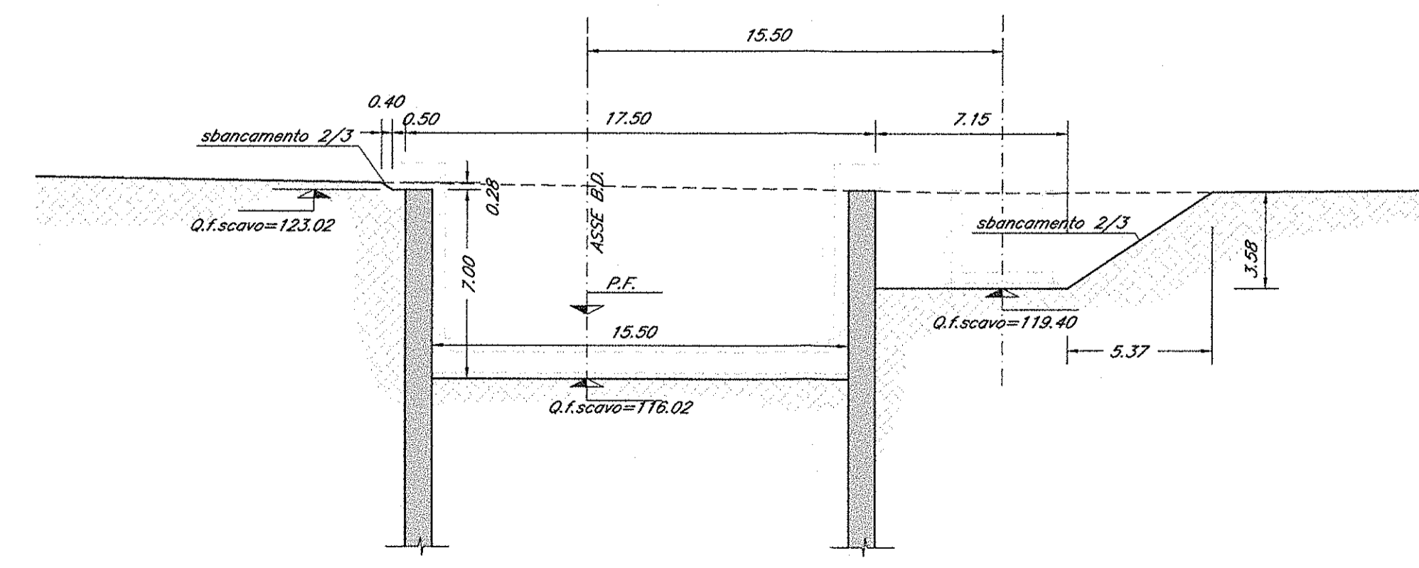
SEZIONE 6: Prog. 7+150.00
