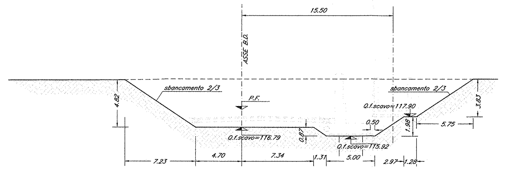
SEZIONE 7: Prog. 7+200.00
