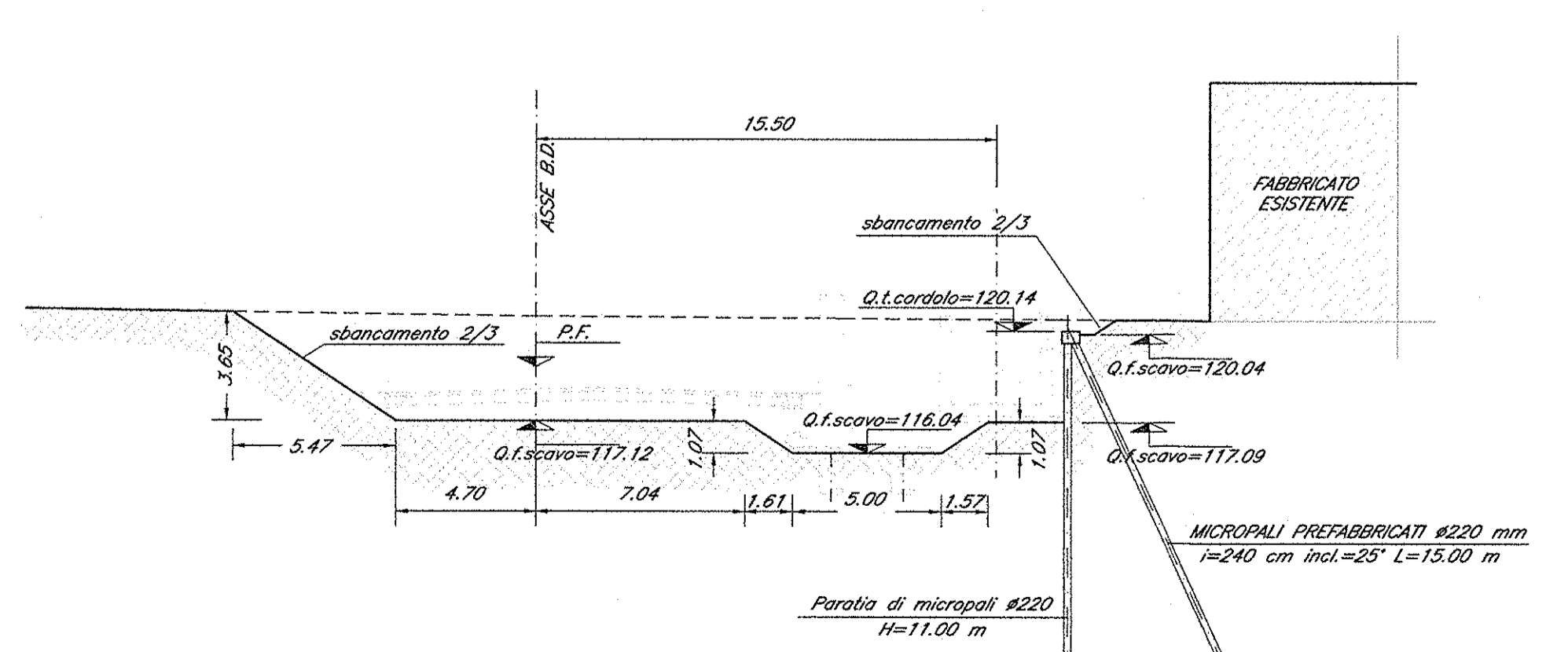
SEZIONE 9: Prog. 7+281.00 Scala 1:200
