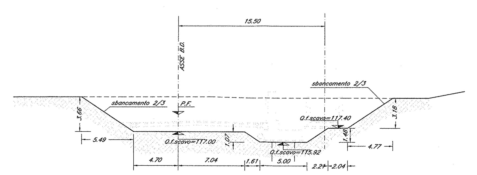
SEZIONE 8: Prog. 7+250.00 Scala 1:200
