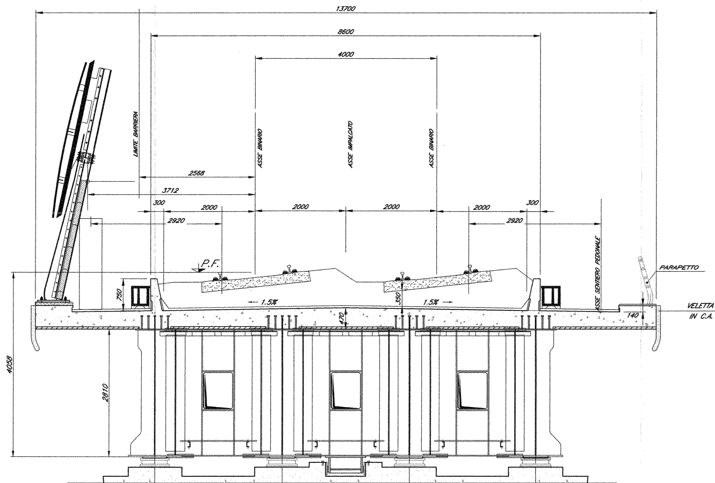
SEZIONE DI TESTATA
