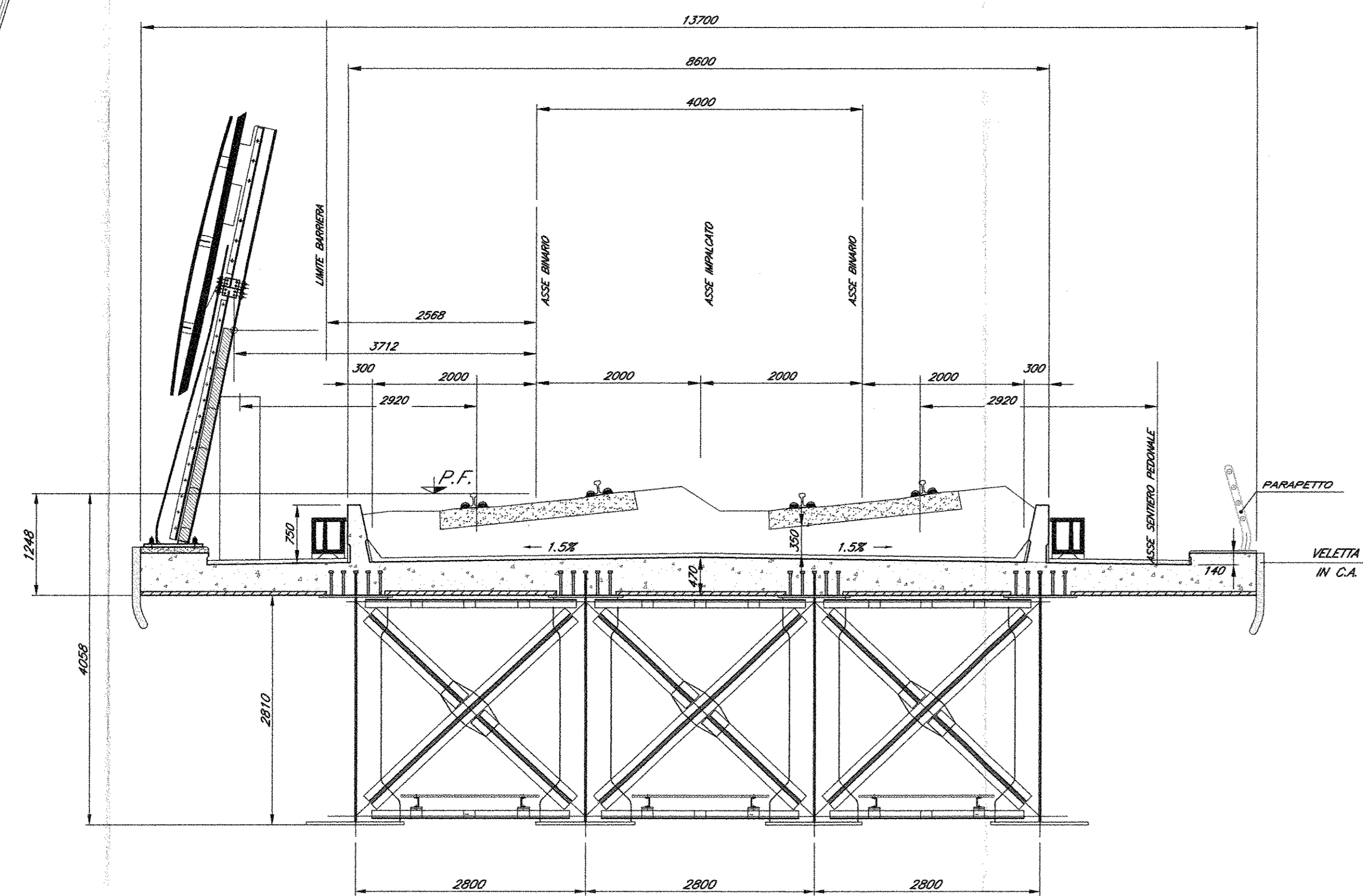
SEZIONE SU DIAFRAMMA
