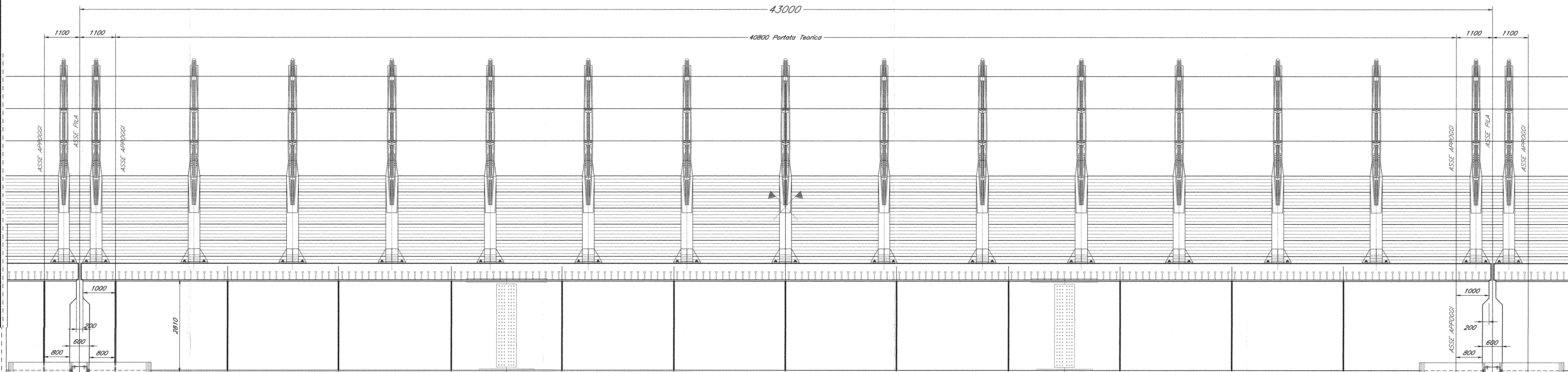
PROSPETTO CAMPATA
