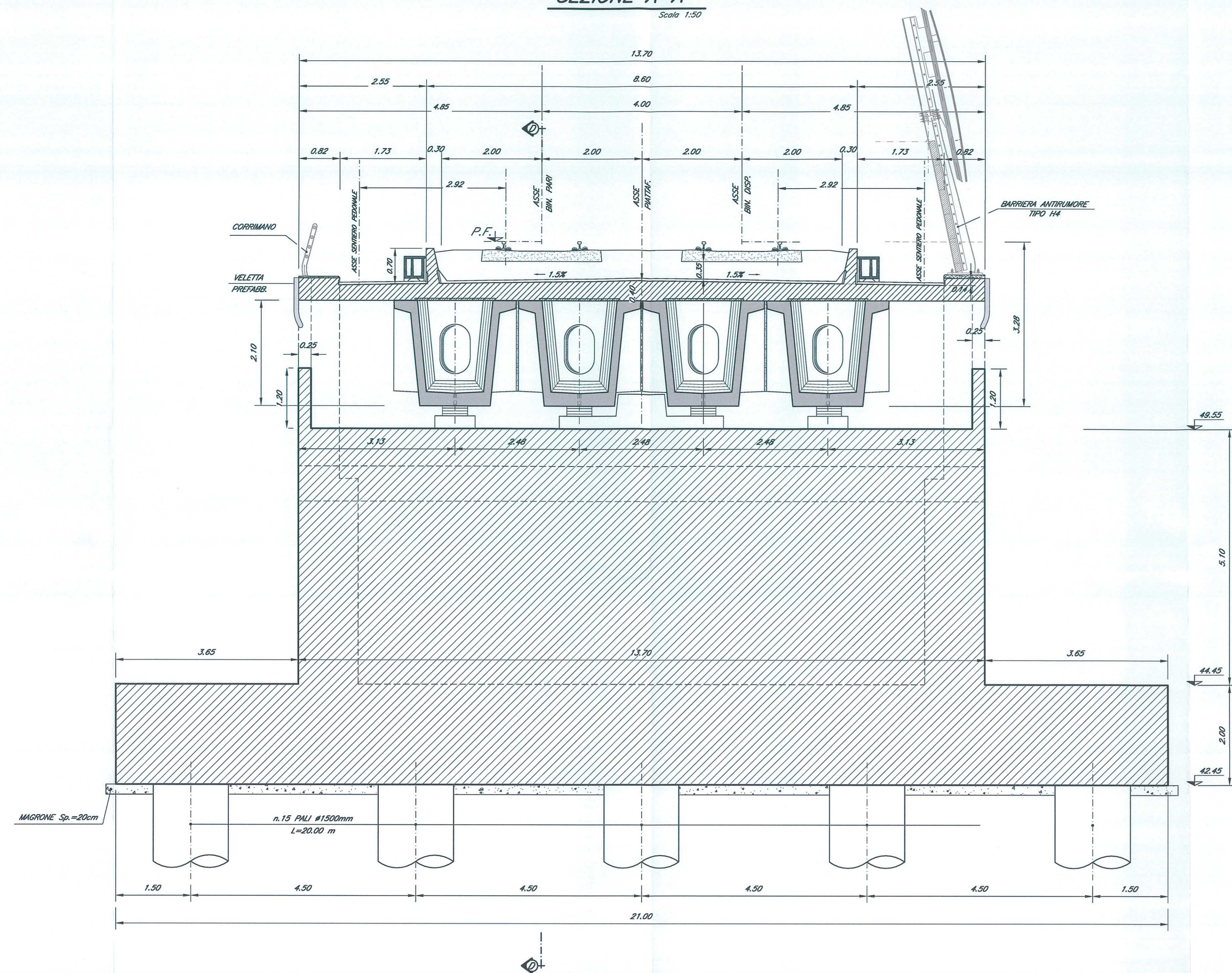
SEZIONE A-A Scala 1:30
