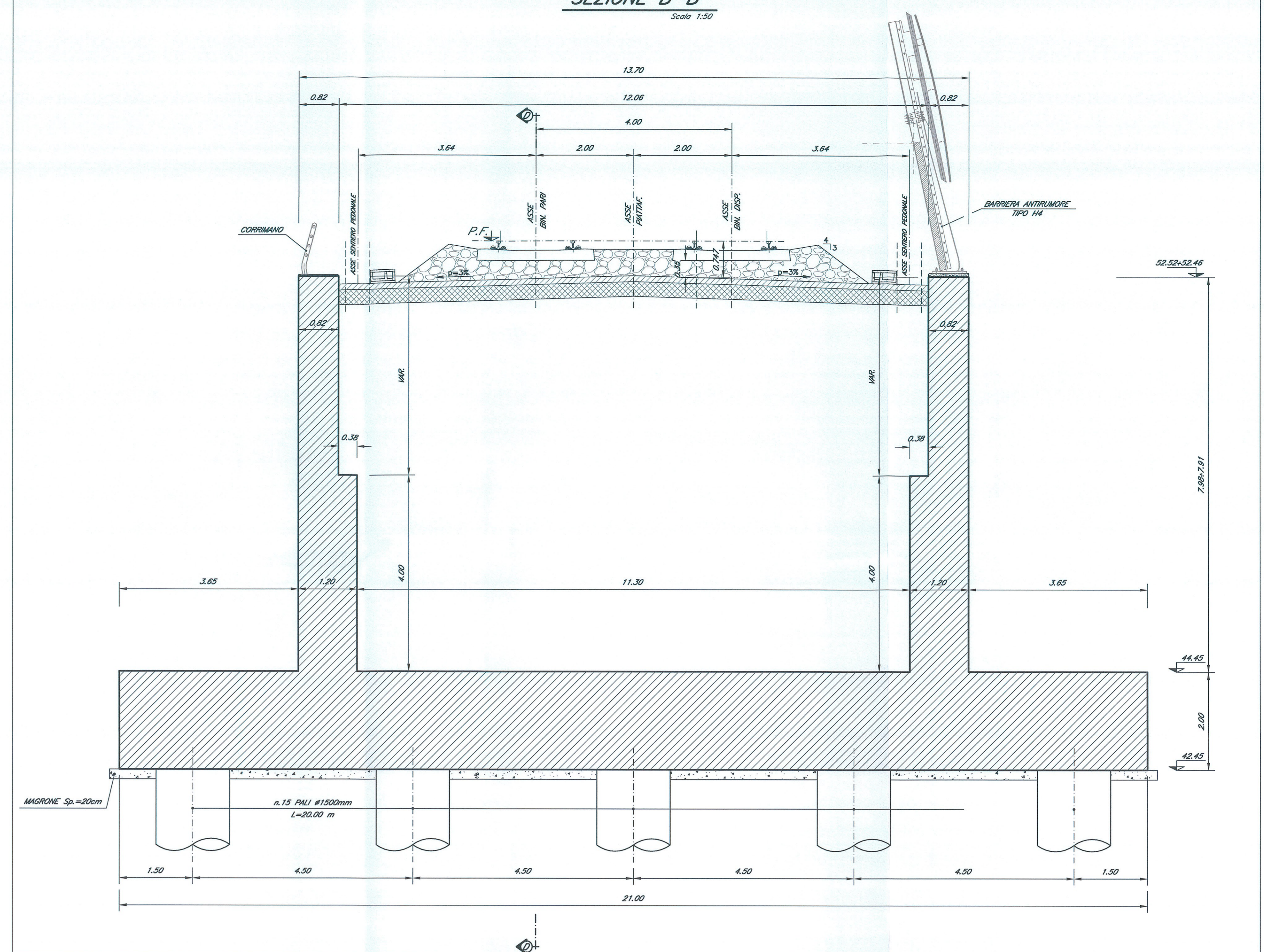
SEZIONE B-B Scala 1:30
