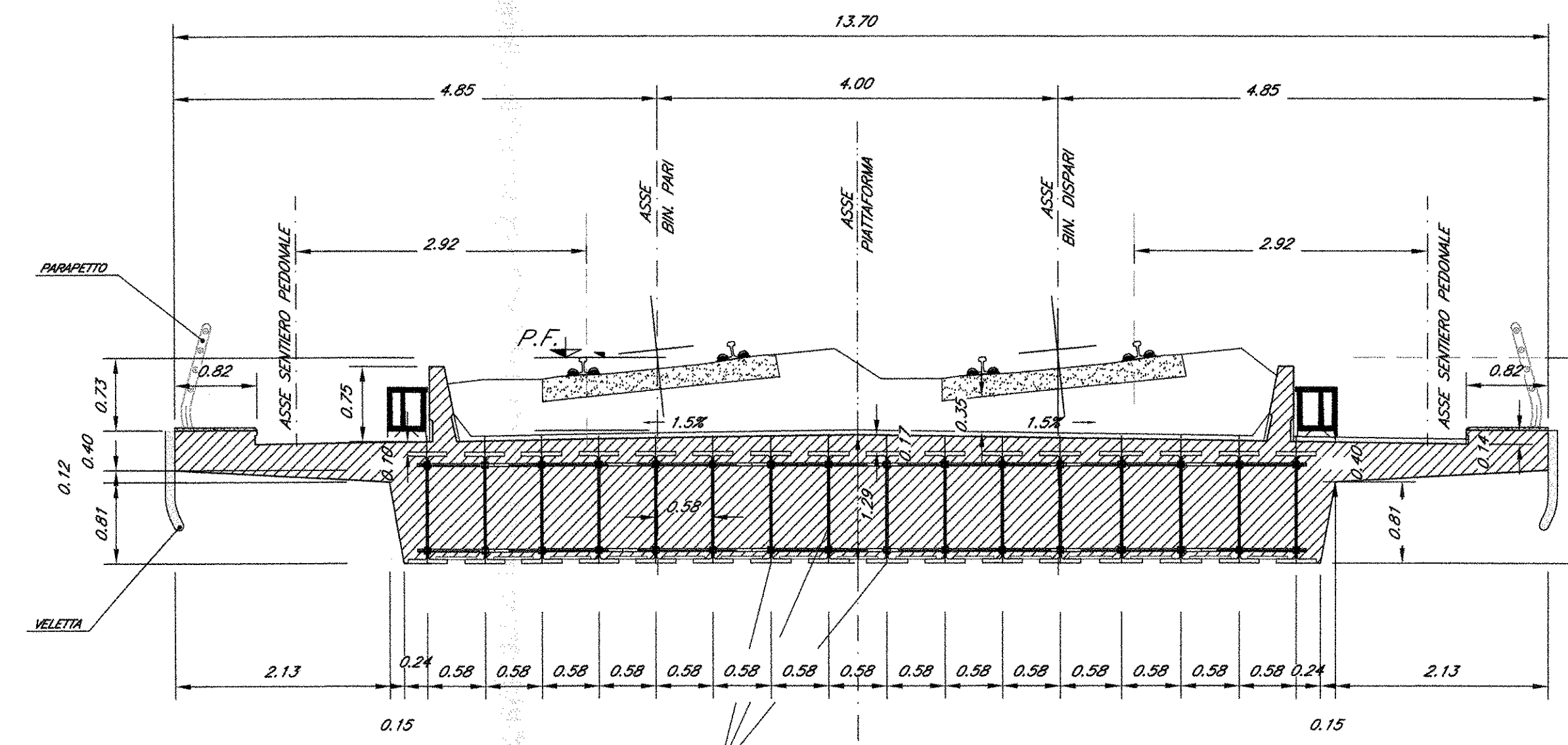
SEZIONE TRASVERSALE Scale 1:50
