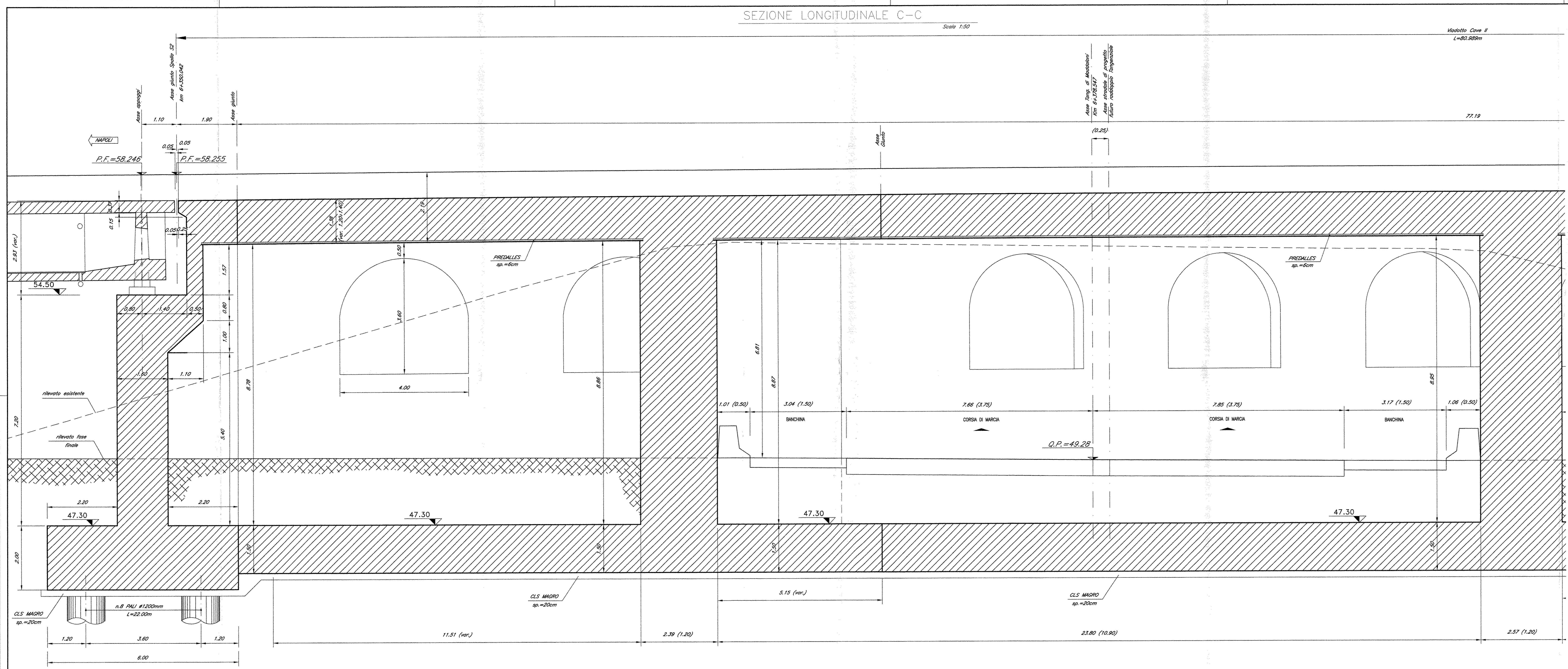
SEZIONE LONGITUDINALE C-C
