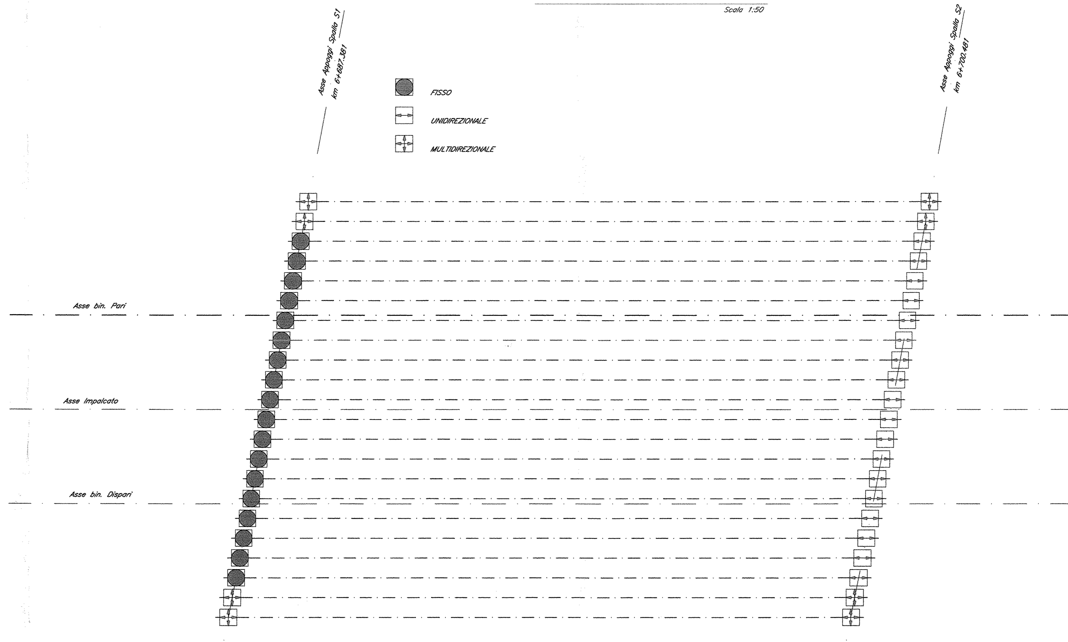
SCHEMA APPOGGI Scala 1:50
