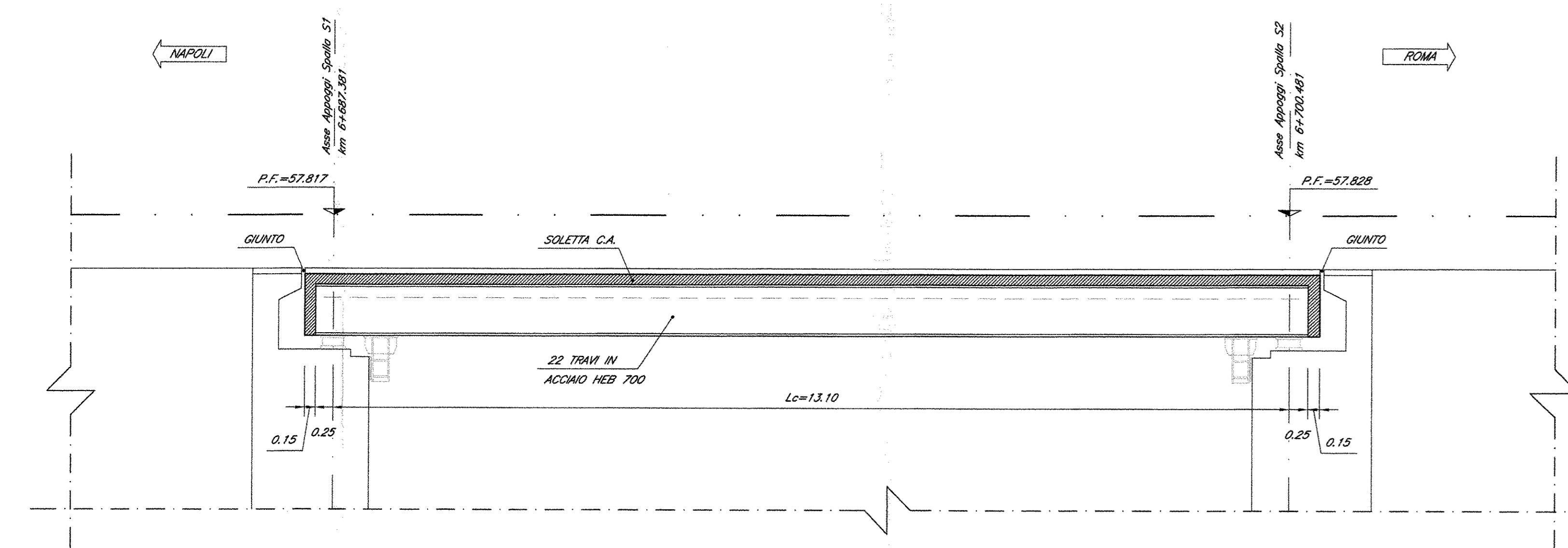
SEZIONE LONGITUDINALE Scala 1:50
