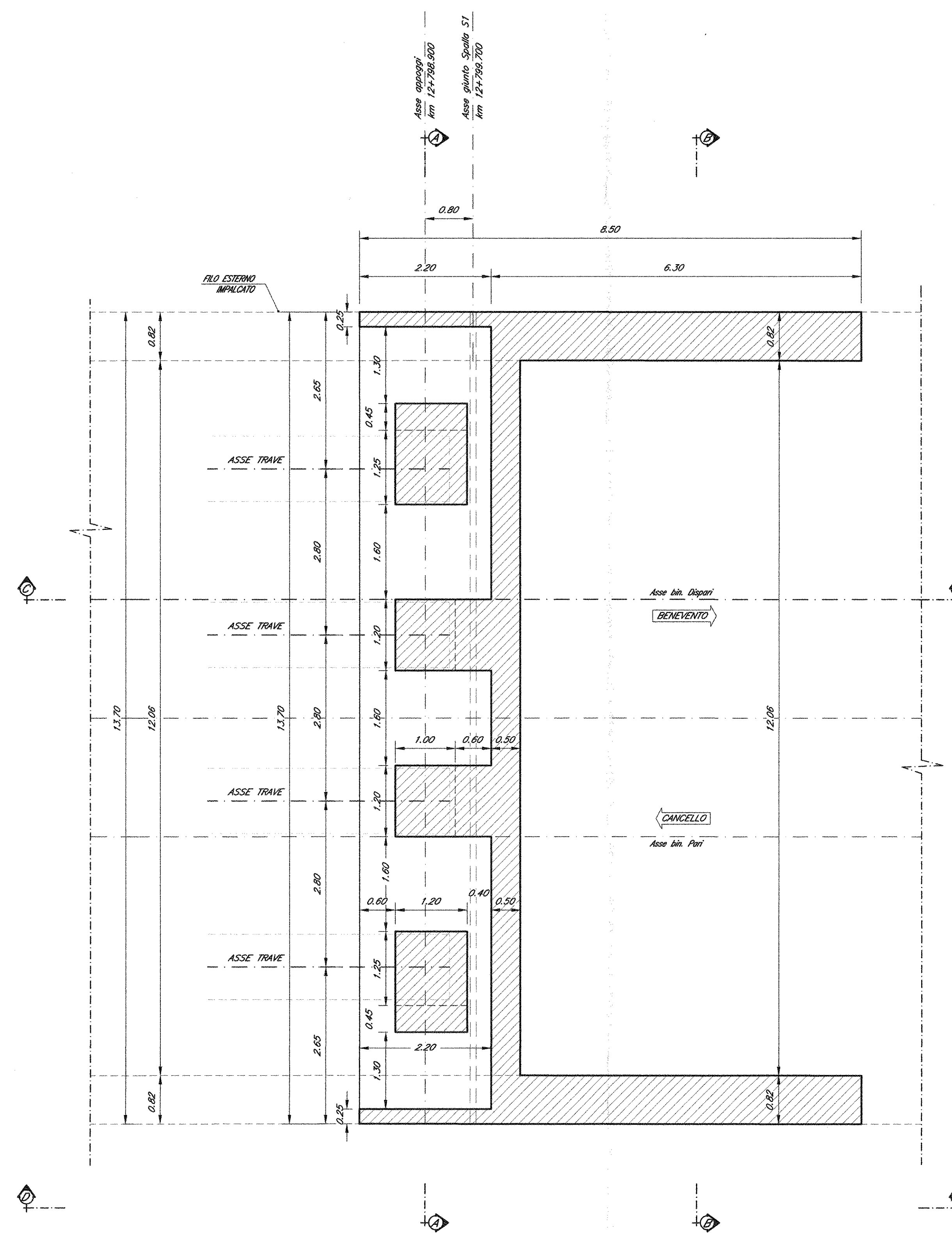
PIANTA APPOGGI
