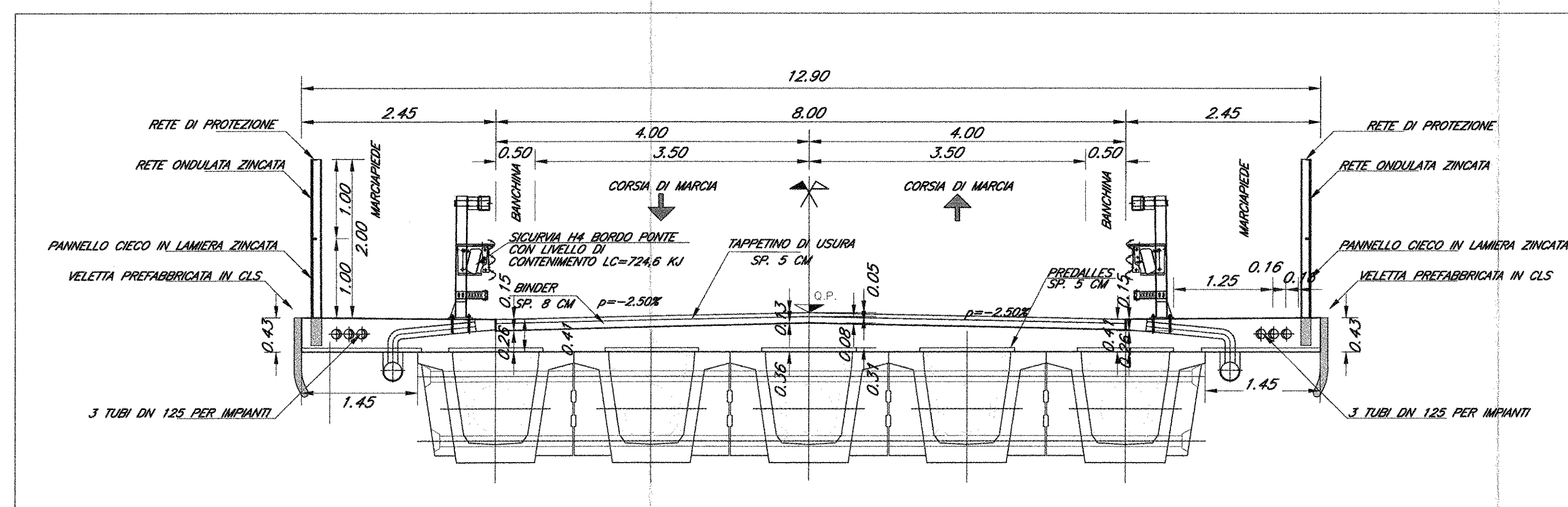
SEZIONE TIPO - PIATTAFORMA STRADALE DI VIA CARMIGNANA
