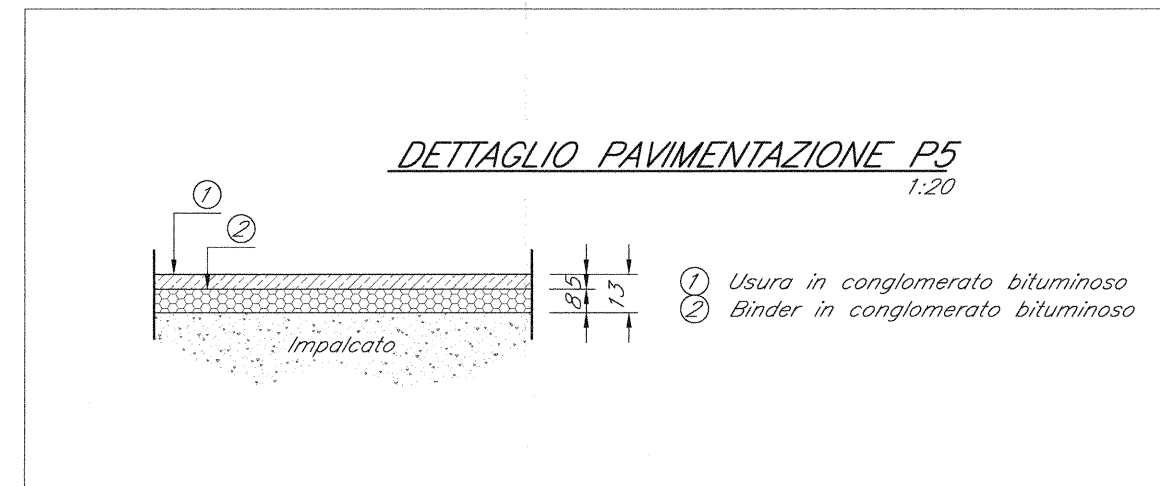
DETTAGLIO PAVIMENTAZIONE SU IMPALCATO
