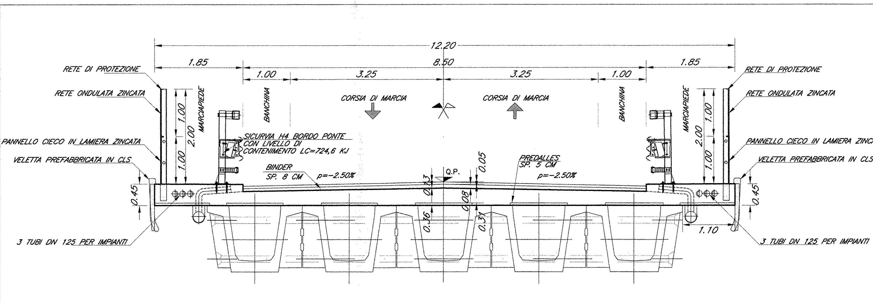
DETTAGLIO PAVIMENTAZIONE SU IMPALCATO
