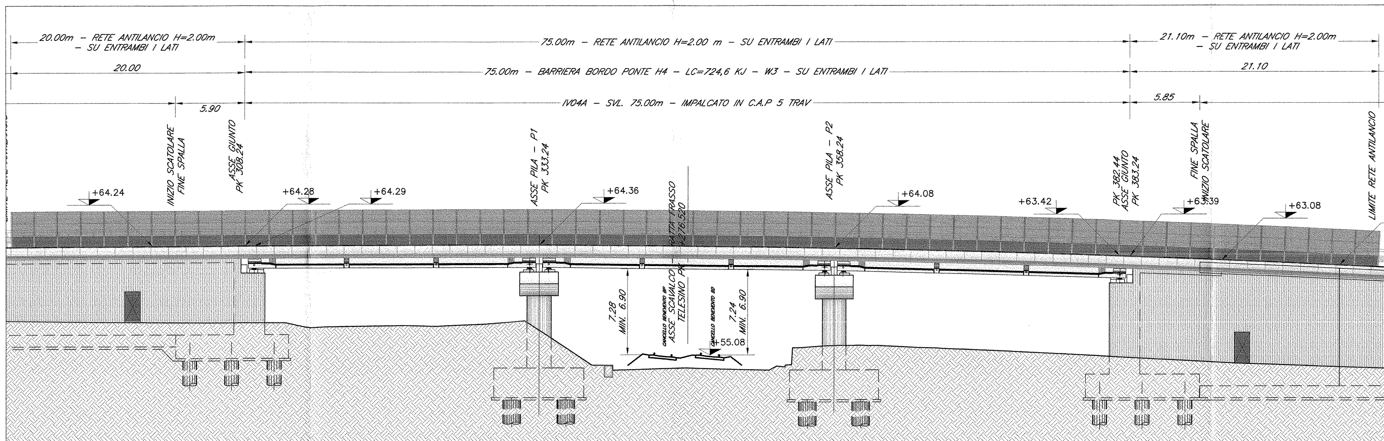
PROSPETTO LONGITUDINALE - IV04
