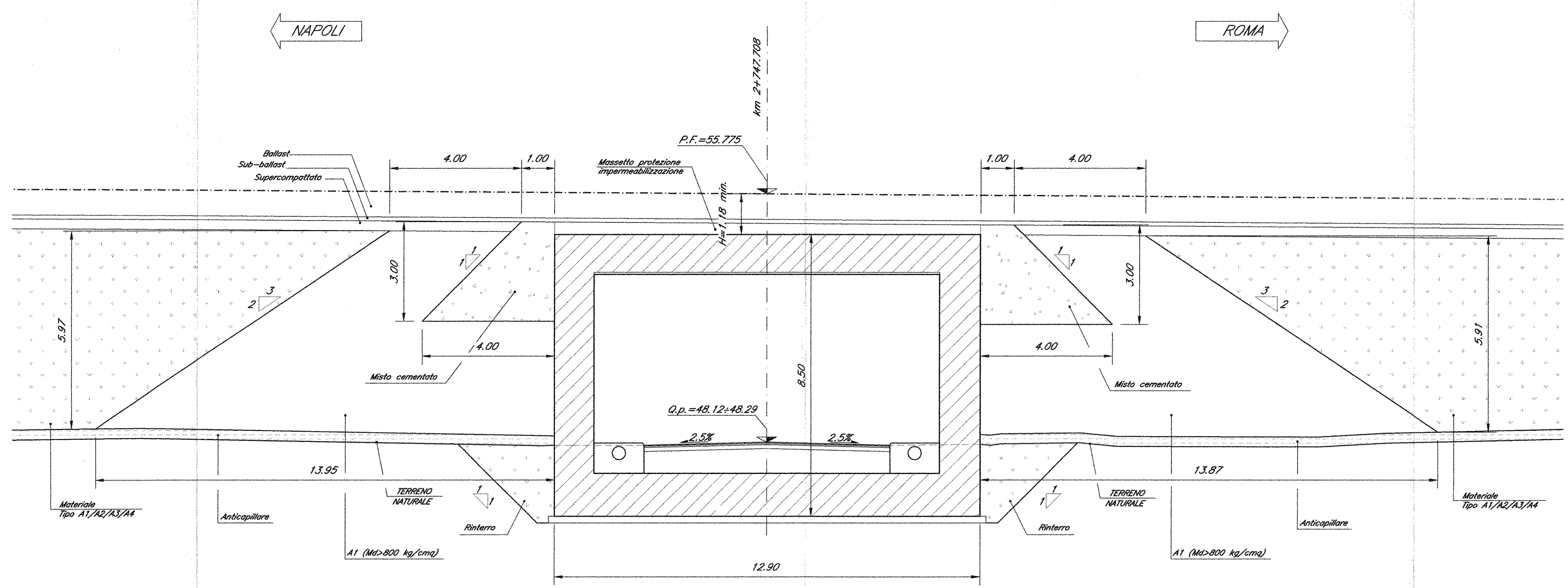
SEZIONE TRASVERSALE
