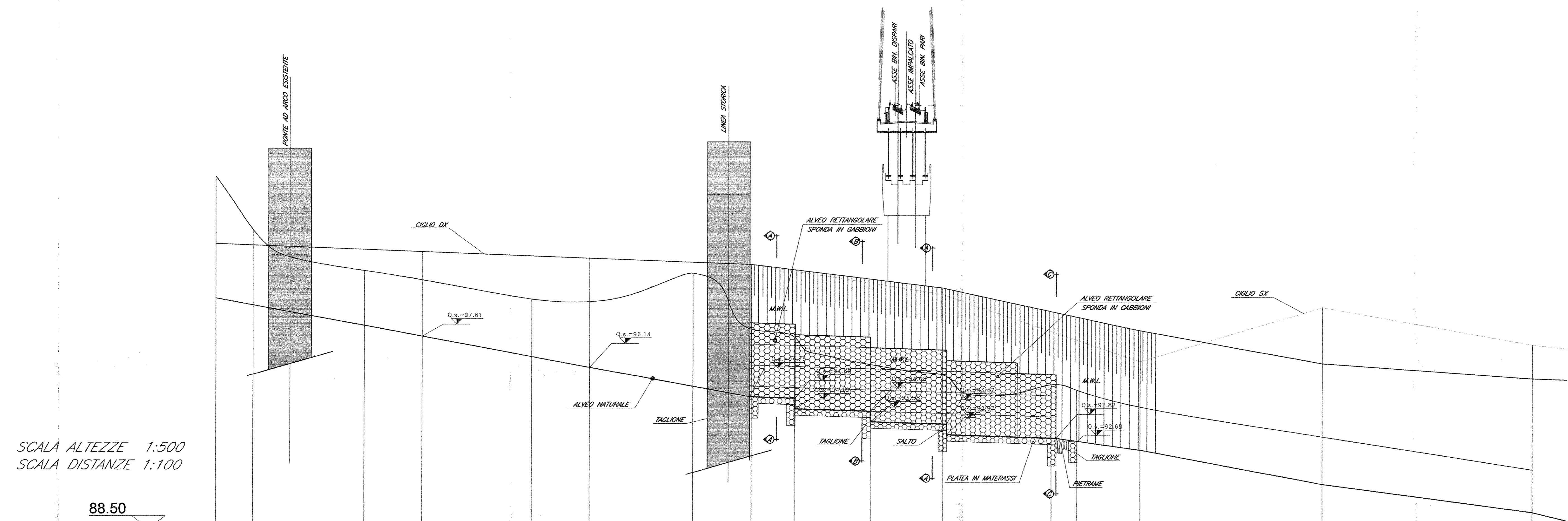
PROFILO LONGITUDINALE: Post-Operam Scala 1:500
